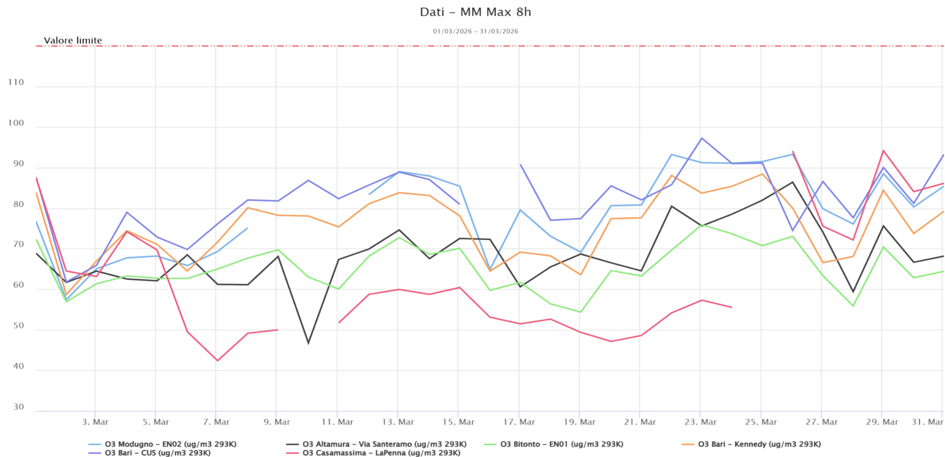
Figura n. 4 - O3 Massima media mobile 8 ore
