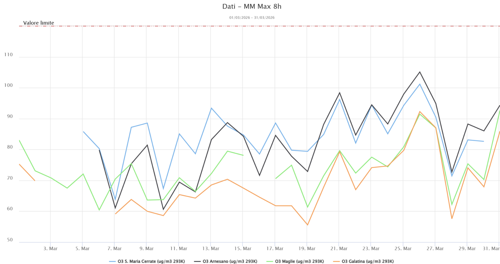
Figura n. 4 - O3 Massima media mobile 8 ore
