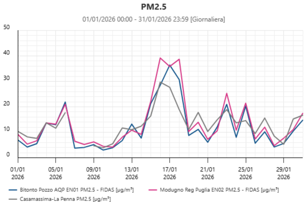
Figura n. 4 - PM2.5 Medie giornaliere rete Sorgenia e Casamassima-La Penna
