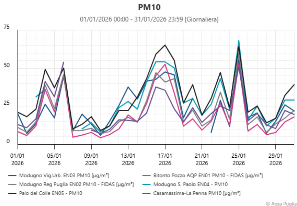
Figura n. 2 - PM10 medie giornaliere rete Sorgenia e Casamassima-La Penna
