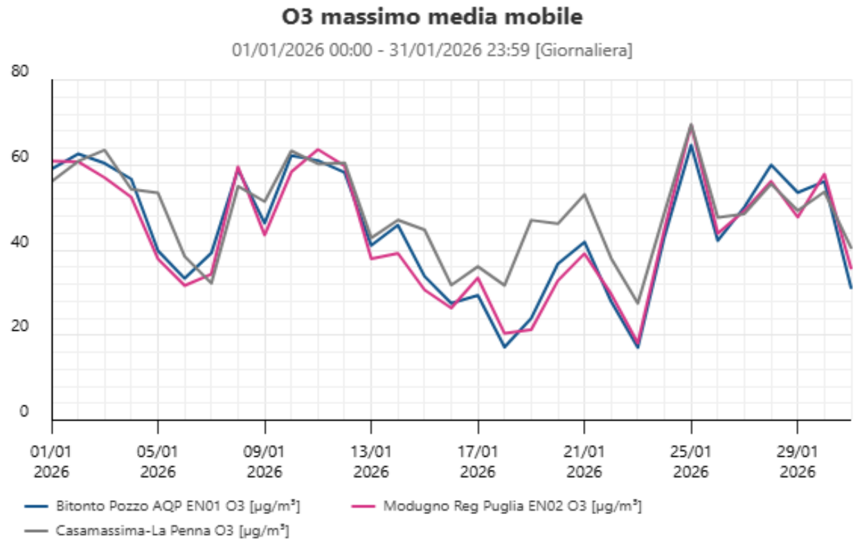
Figura n. 8 - O3 Massima media mobile 8 ore Sorgenia e Casamassima-La Penna
