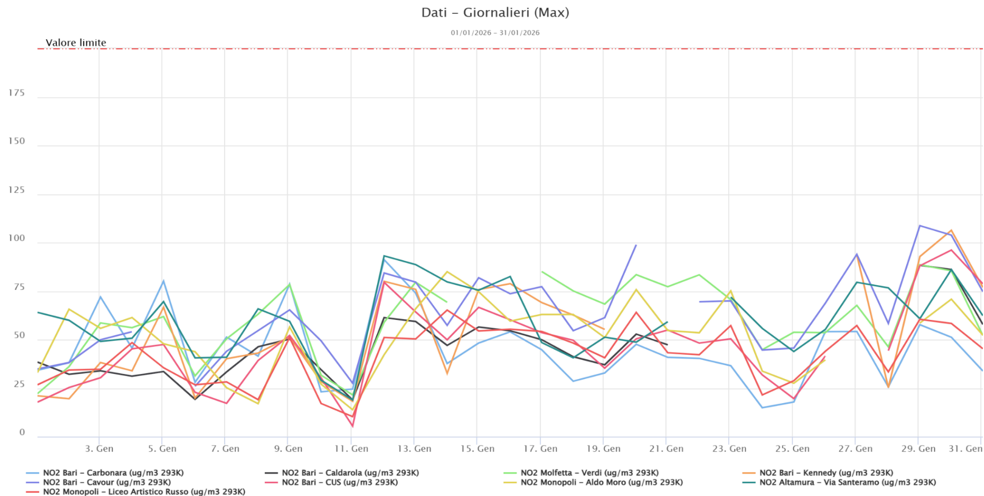
Figura n. 5 - NO2 Massimo orario giornaliero
