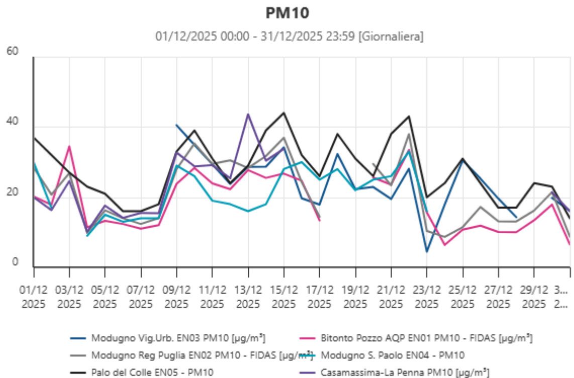
Figura n. 2 - PM10 medie giornaliere rete Sorgenia e Casamassima-La Penna
