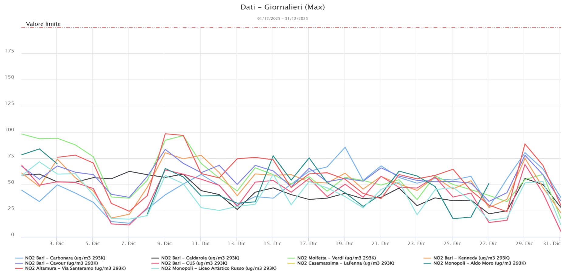
Figura n. 5 - NO2 Massimo orario giornaliero
