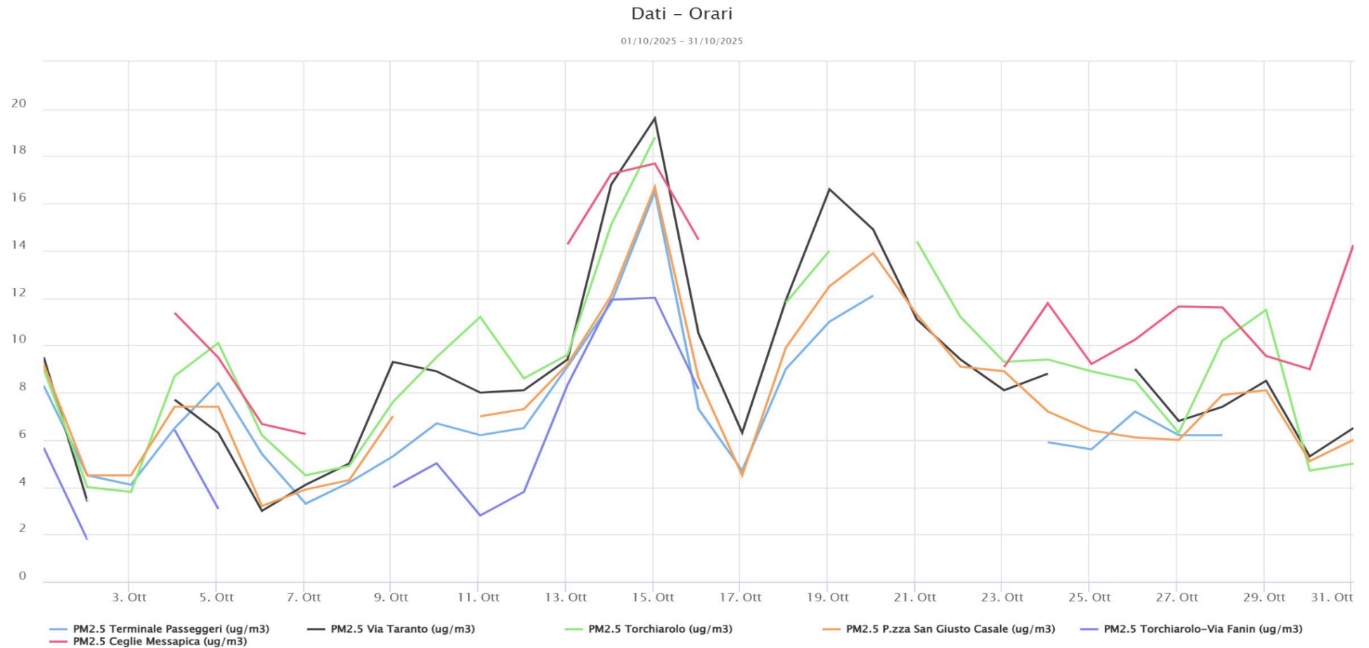
Figura n. 2 - PM2.5 medie giornaliere
