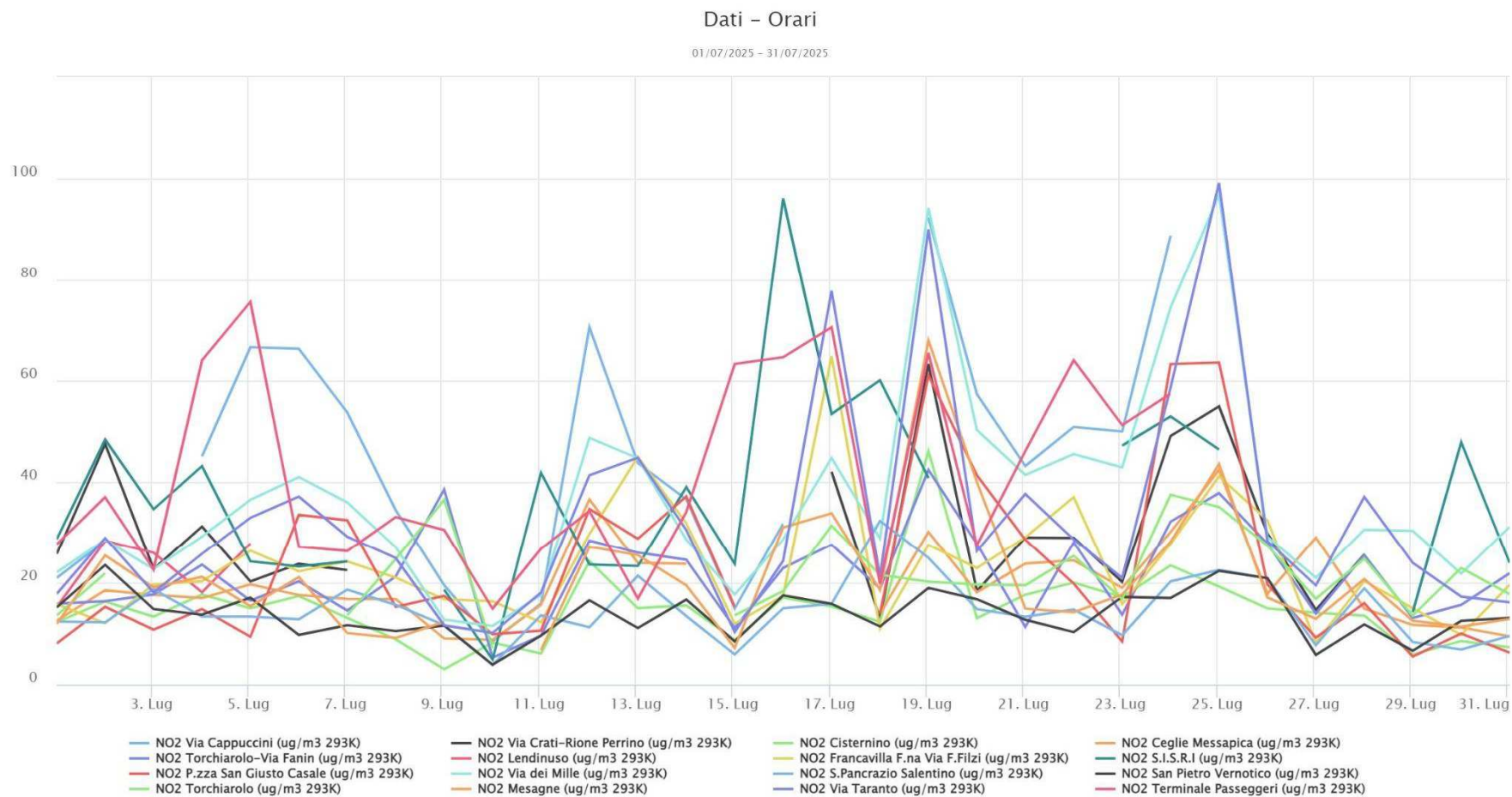
Figura n. 3 - NO 2 Massimo orario giornaliero
