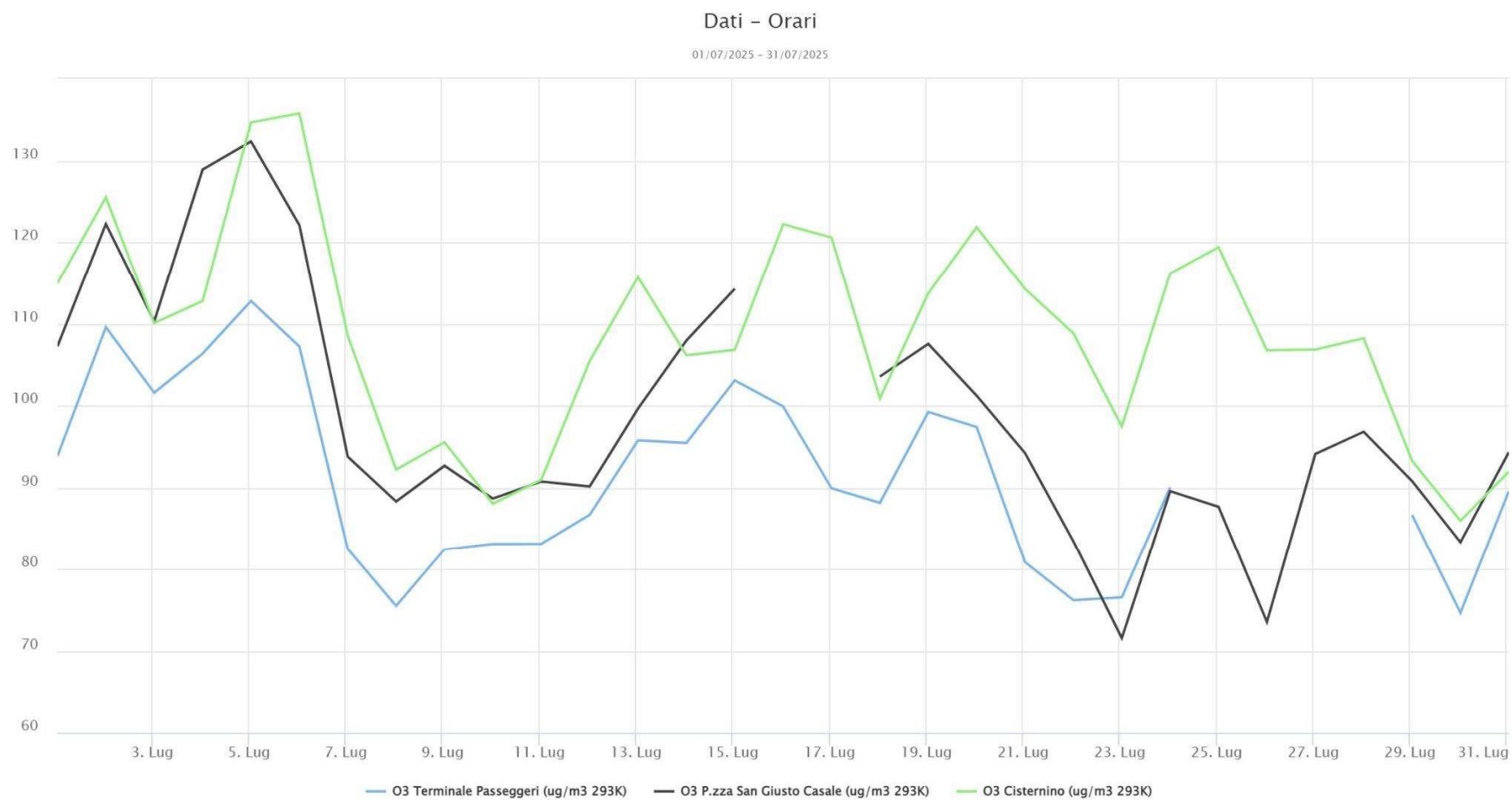
Figura n. 4 - O 3 Massimo media mobile 8 ore
