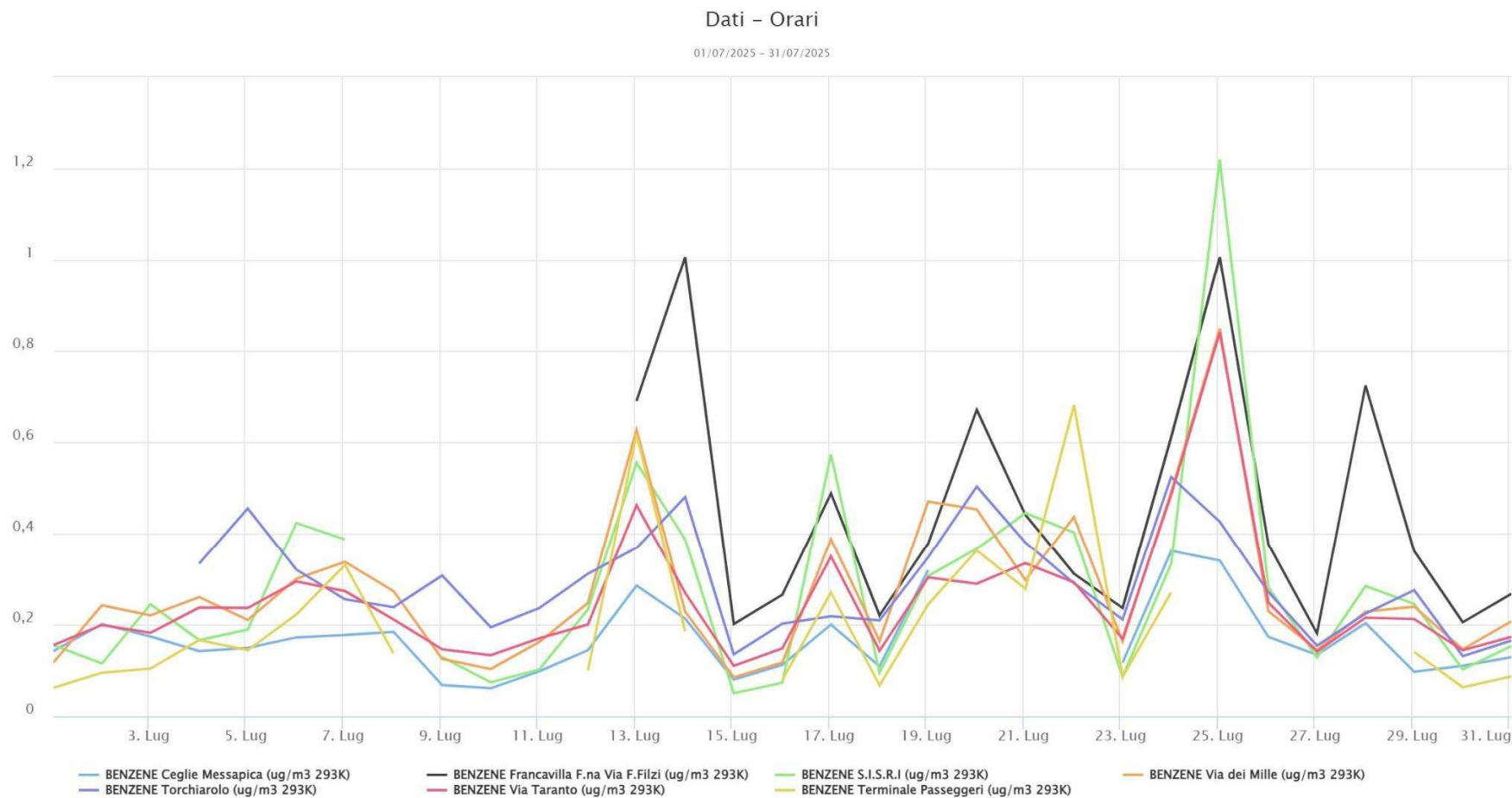
Figura n. 5 - Benzene medie giornaliere
