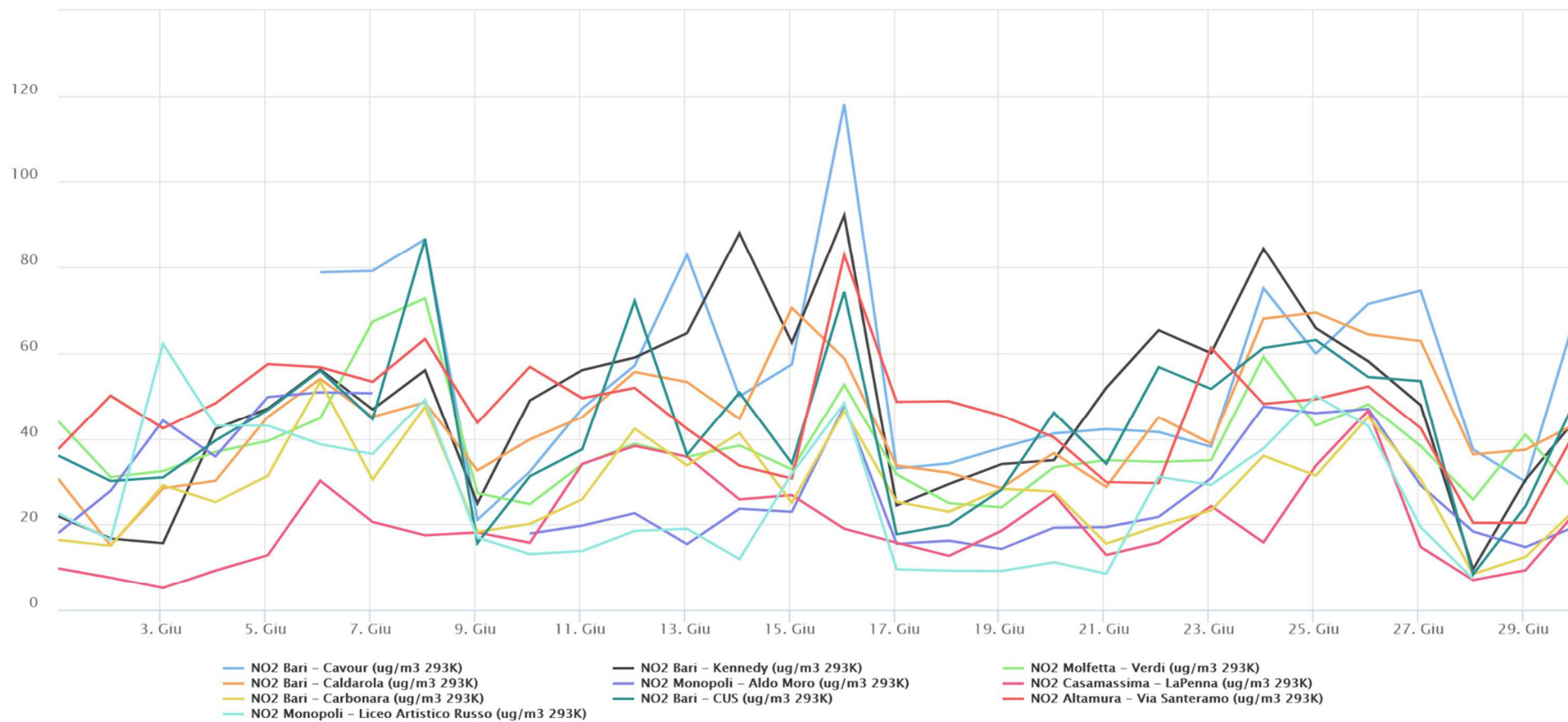
Figura n. 6 - NO2 Massimo orario giornaliero Sorgenia
