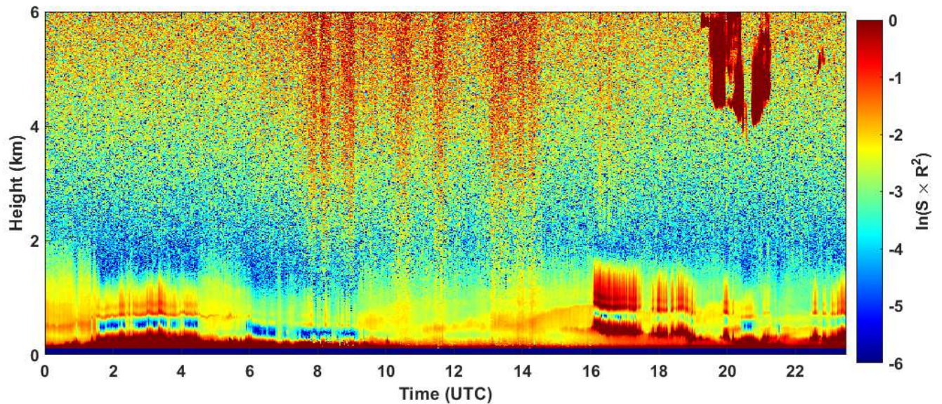
2025-01-27 RCS quick look CHM15k - ILVA LIDAR1 DIREZIONE
