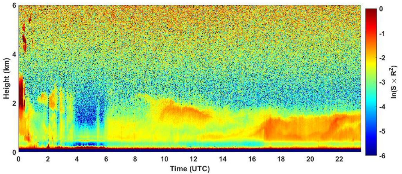
2025-01-08 RCS quick look CHM15k - ILVA LIDAR1 DIREZIONE
