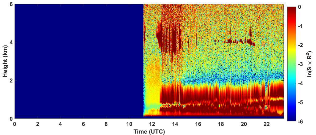
2025-01-23 RCS quick look CHM15k - ILVA LIDAR1 DIREZIONE
