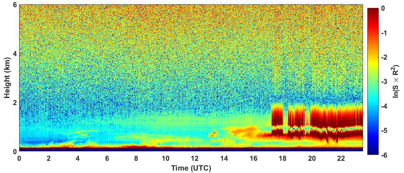
2025-01-02 RCS quick look CHM15k - ILVA LIDAR1 DIREZIONE
