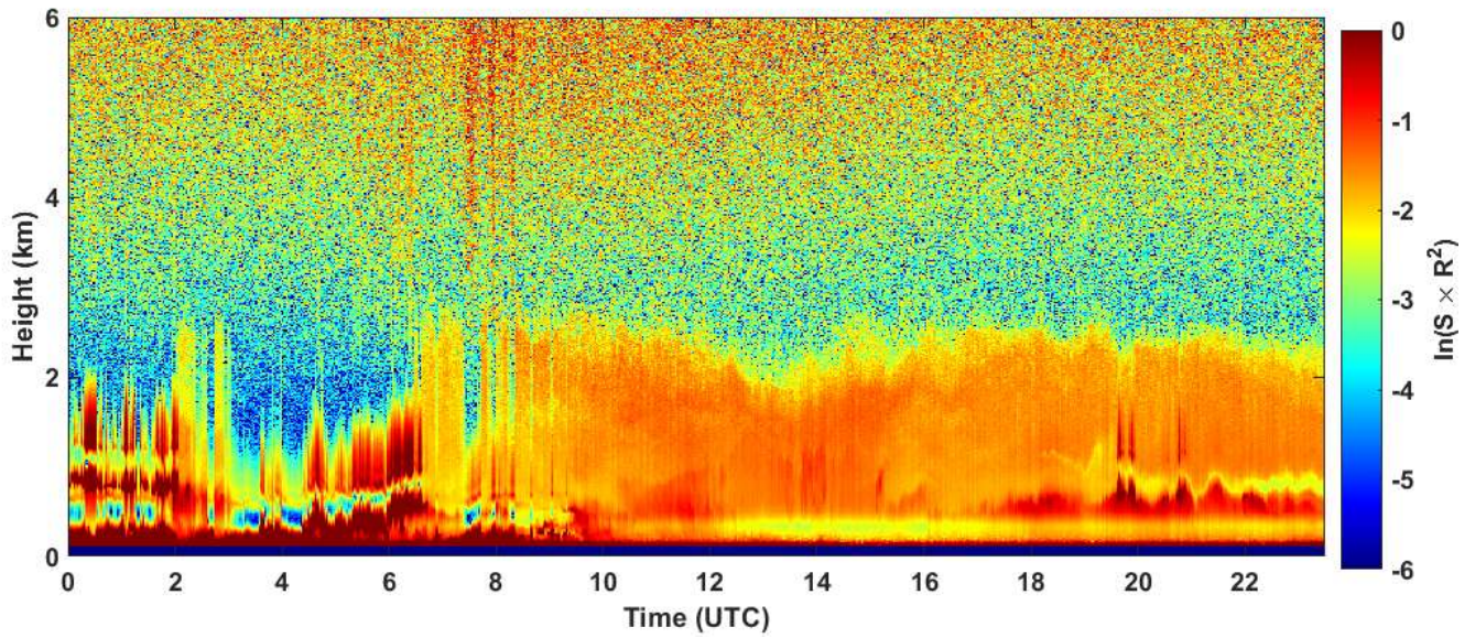
2025-01-25 RCS quick look CHM15k - ILVA LIDAR1 DIREZIONE
