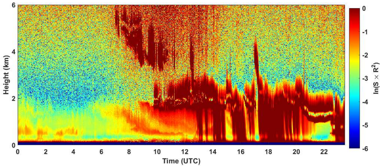
2025-01-29 RCS quick look CHM15k - ILVA LIDAR1 DIREZIONE
