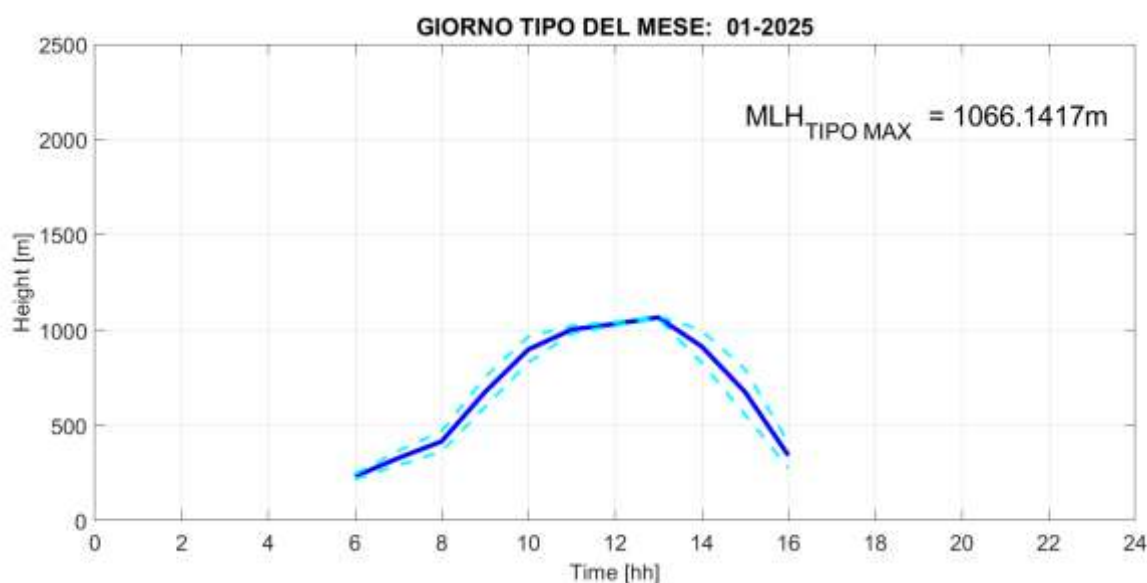
Fig. 2: Giorno tipo del parametro Mixing Layer Height nel mese di GENNAIO 2025, rappresentato mediante media oraria (linea blu continua) e deviazione standard (linee celesti tratteggiate).
