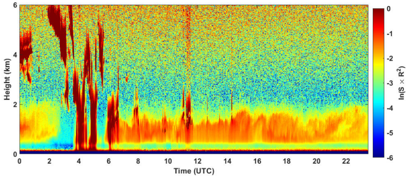
2024-12-22 RCS quick look CHM15k - ILVA LIDAR1 DIREZIONE
