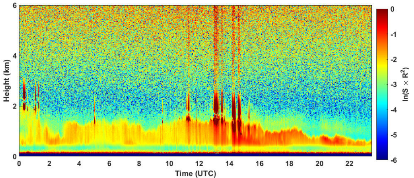
2024-12-16 RCS quick look CHM15k - ILVA LIDAR1 DIREZIONE
