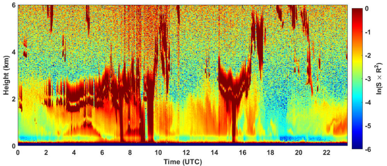
2024-12-20 RCS quick look CHM15k - ILVA LIDAR1 DIREZIONE
