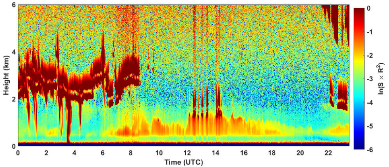
2024-12-08 RCS quick look CHM15k - ILVA LIDAR1 DIREZIONE
