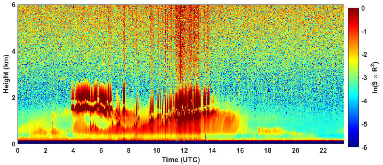
2024-12-30 RCS quick look CHM15k - ILVA LIDAR1 DIREZIONE
