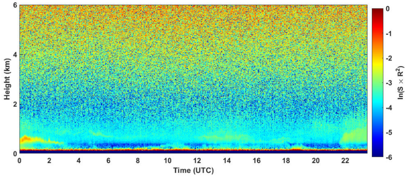
2024-12-18 RCS quick look CHM15k - ILVA LIDAR1 DIREZIONE
