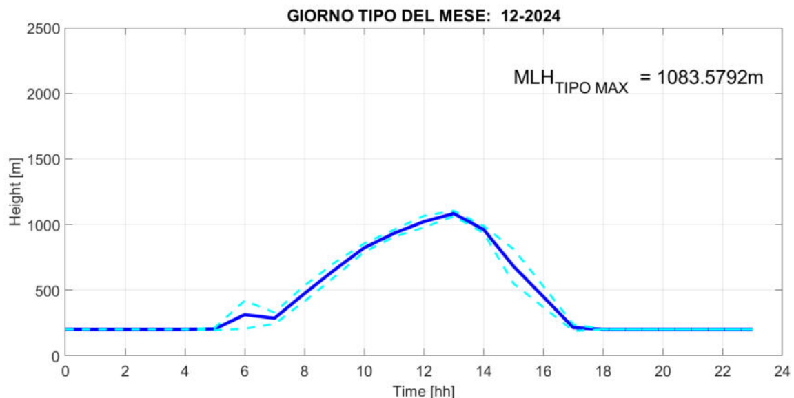
Fig. 2: Giorno tipo del parametro Mixing Layer Height nel mese di DICEMBRE 2024, rappresentato mediante media oraria (linea blu continua) e deviazione standard (linee celesti tratteggiate).
