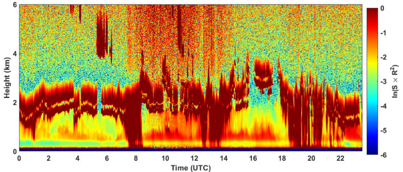
2024-12-02 RCS quick look CHM15k - ILVA LIDAR1 DIREZIONE
