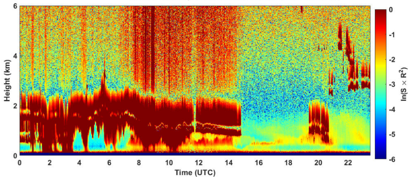
2024-12-06 RCS quick look CHM15k - ILVA LIDAR1 DIREZIONE
