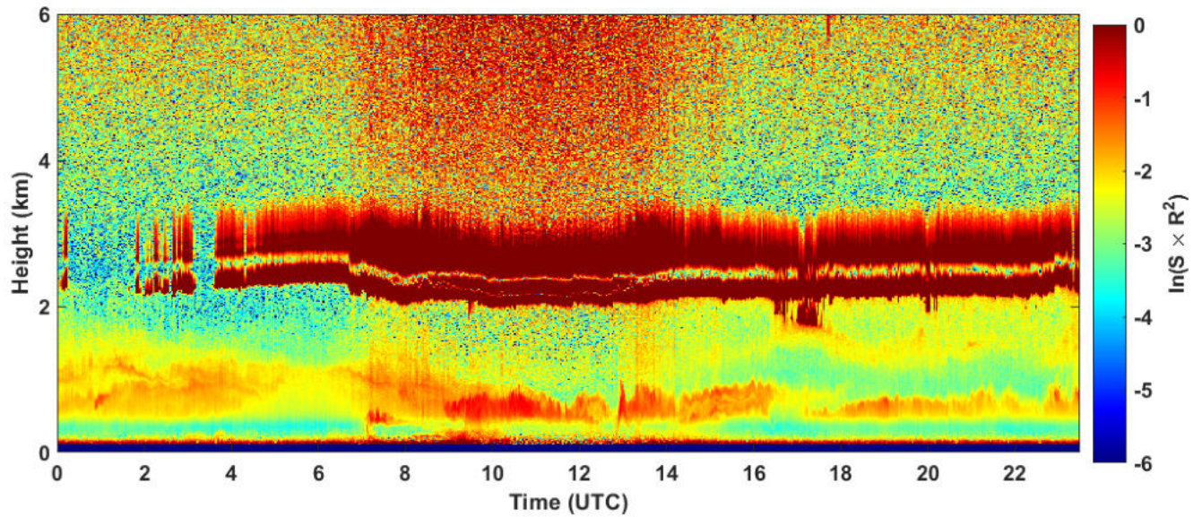
2024-12-04 RCS quick look CHM15k - ILVA LIDAR1 DIREZIONE
