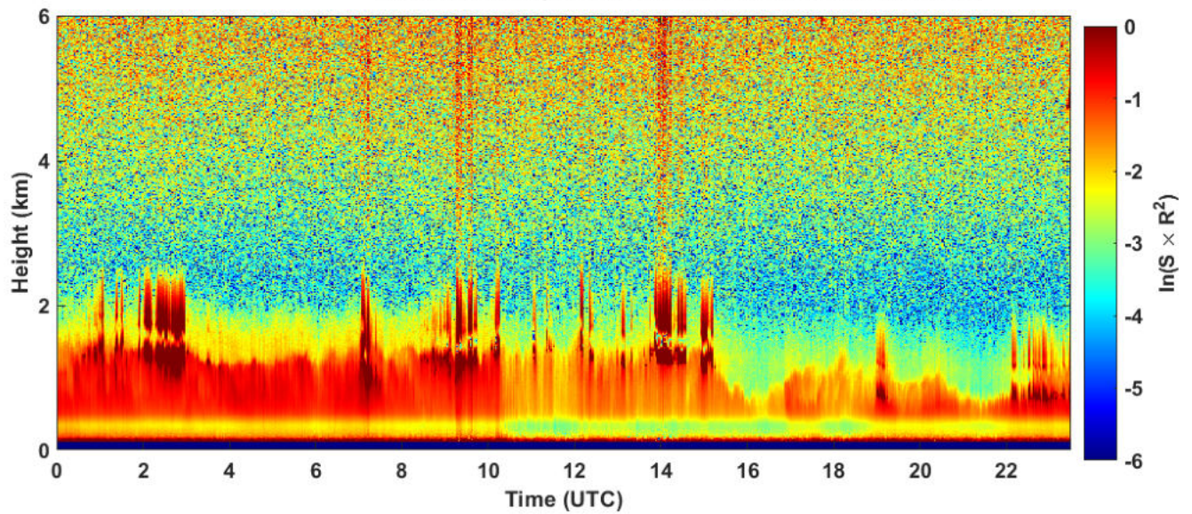
2024-12-28 RCS quick look CHM15k - ILVA LIDAR1 DIREZIONE
