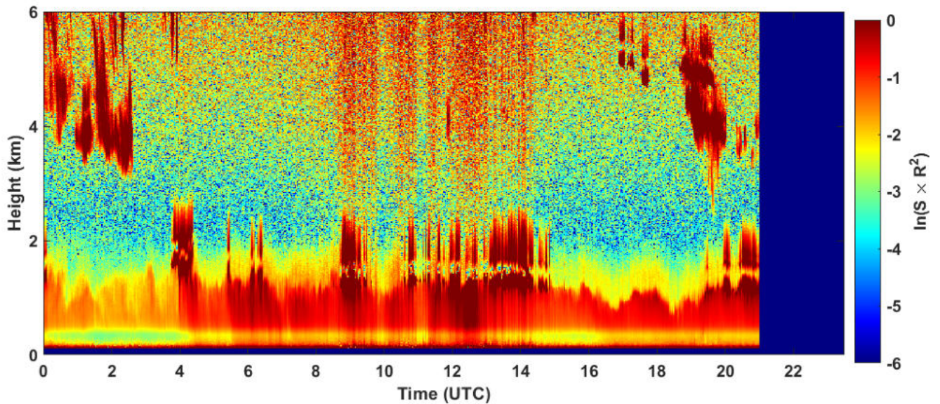
2024-12-26 RCS quick look CHM15k - ILVA LIDAR1 DIREZIONE
