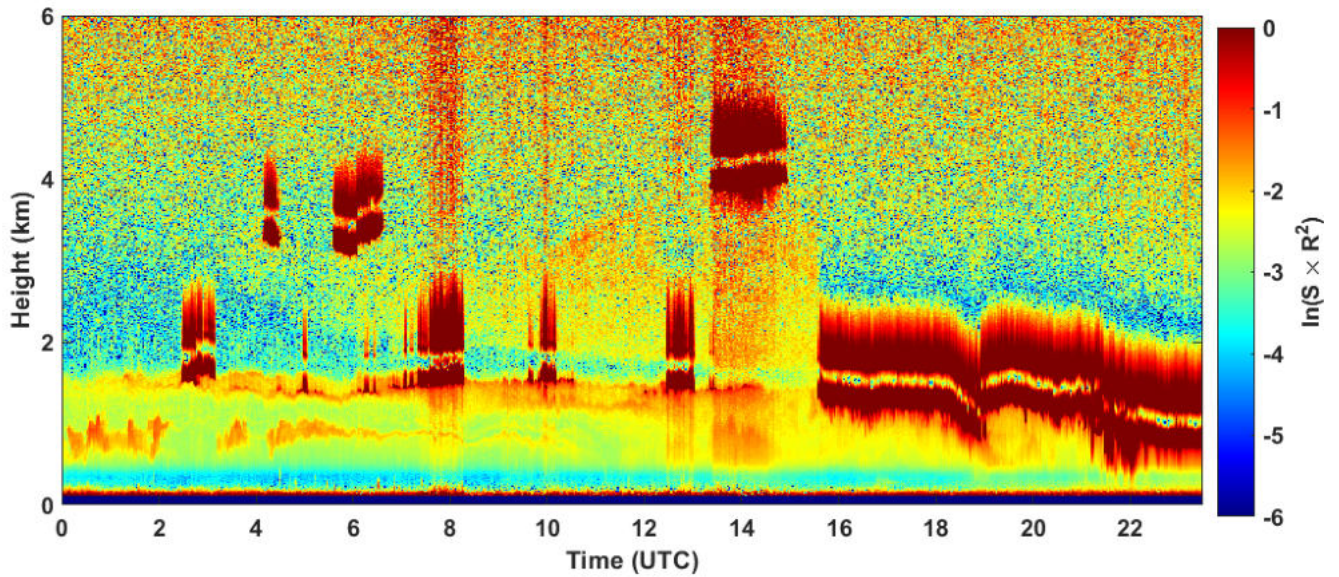
2024-12-14 RCS quick look CHM15k - ILVA LIDAR1 DIREZIONE
