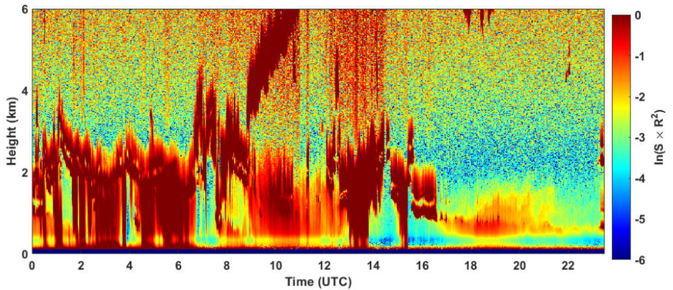
2024-12-24 RCS quick look CHM15k - ILVA LIDAR1 DIREZIONE
