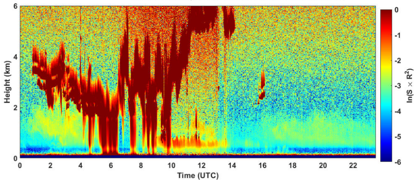
2024-12-10 RCS quick look CHM15k - ILVA LIDAR1 DIREZIONE
