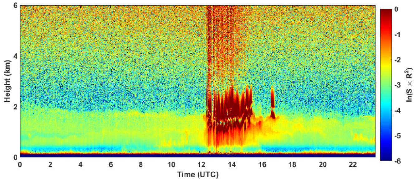
2024-12-12 RCS quick look CHM15k - ILVA LIDAR1 DIREZIONE
