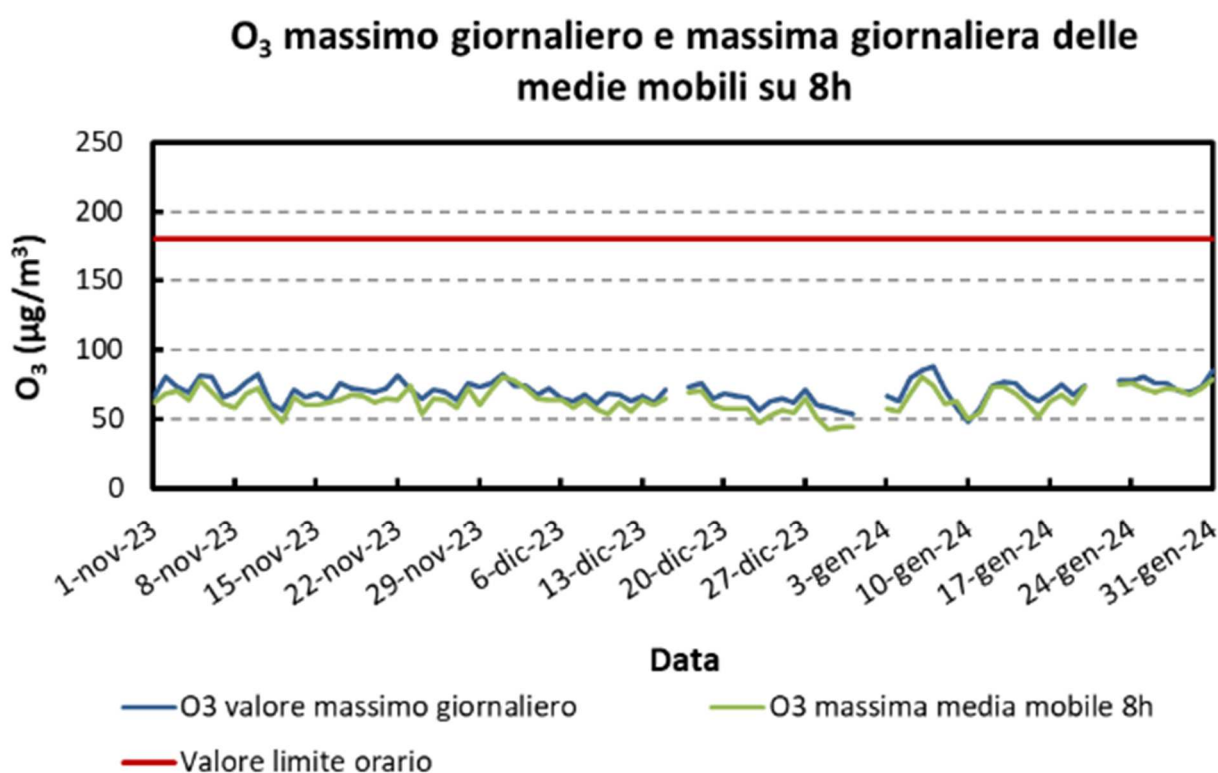
Figura 8: Andamento giornaliero del valore massimo e della massima media mobile misurata sulle 8 ore per l'inquinante ozono ( \mu\text{g}/\text{m}^3 ).
