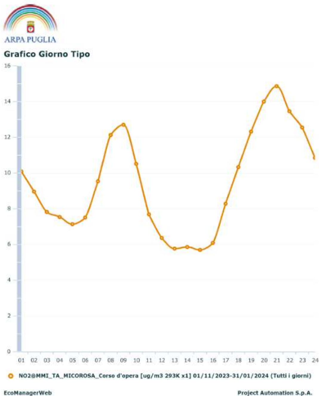
Figura 17: Grafico del giorno tipo per l'inquinante NO 2 .
