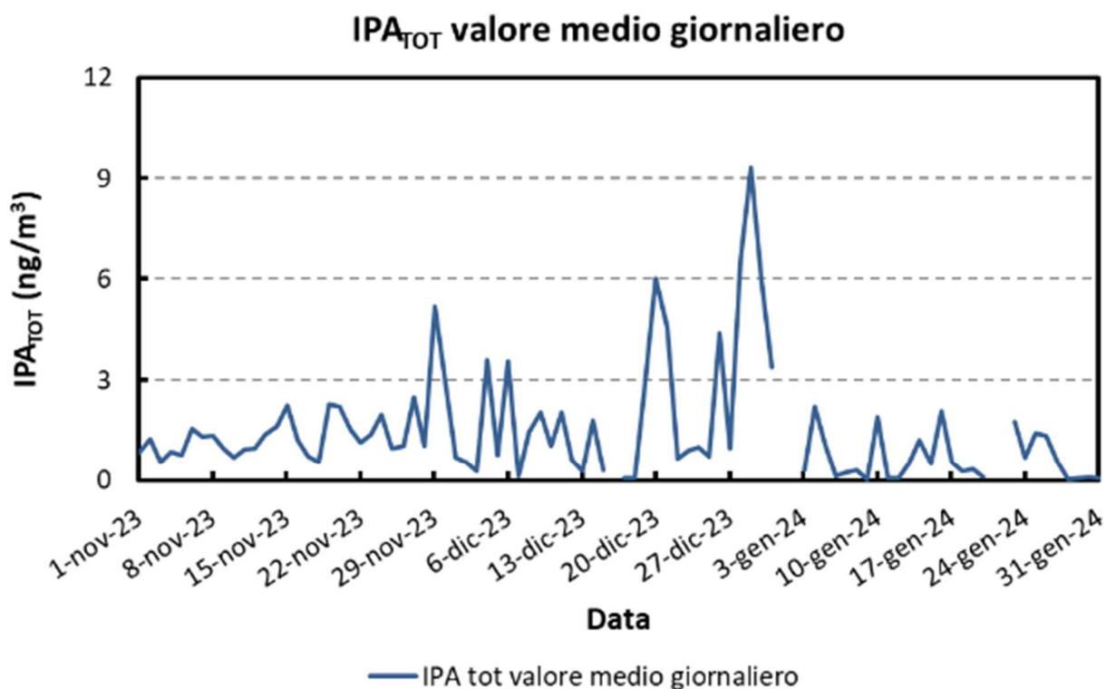
Figura 15: Andamento della concentrazione media giornaliera, per gli idrocarburi policiclici aromatici (ng/m 3 ), misurata presso il sito oggetto della campagna.
