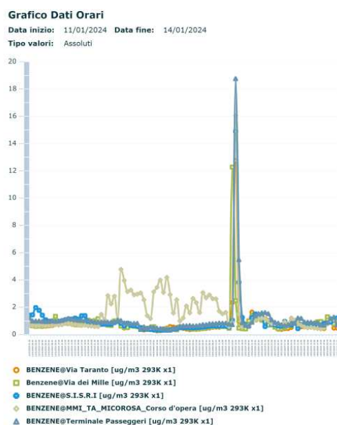
Figura 13a: Andamento delle concentrazioni orarie di benzene misurate nelle centraline di Brindisi (11÷14 gennaio 2024)
