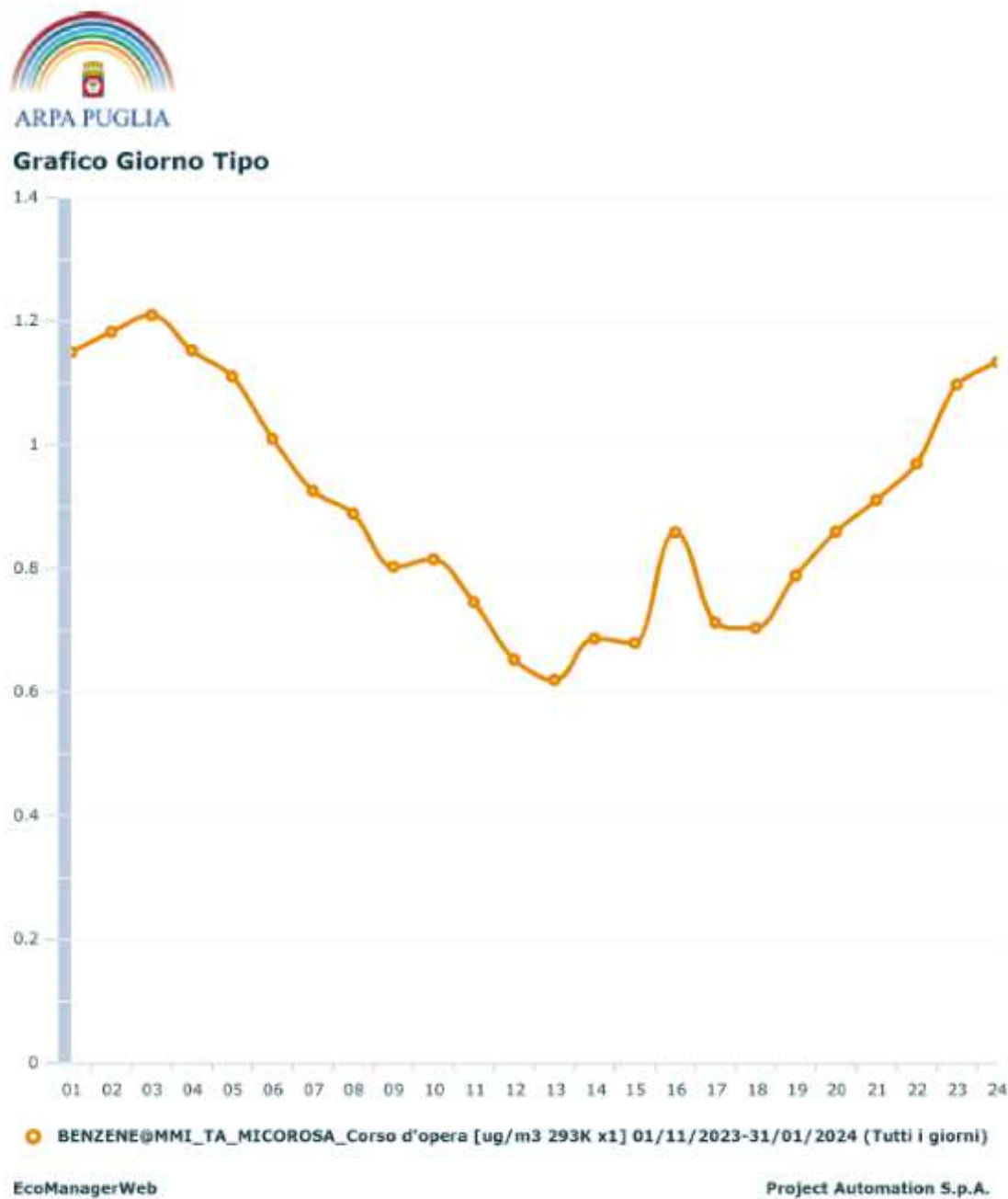
Figura 20: Grafico del giorno tipo per l'inquinante benzene.
