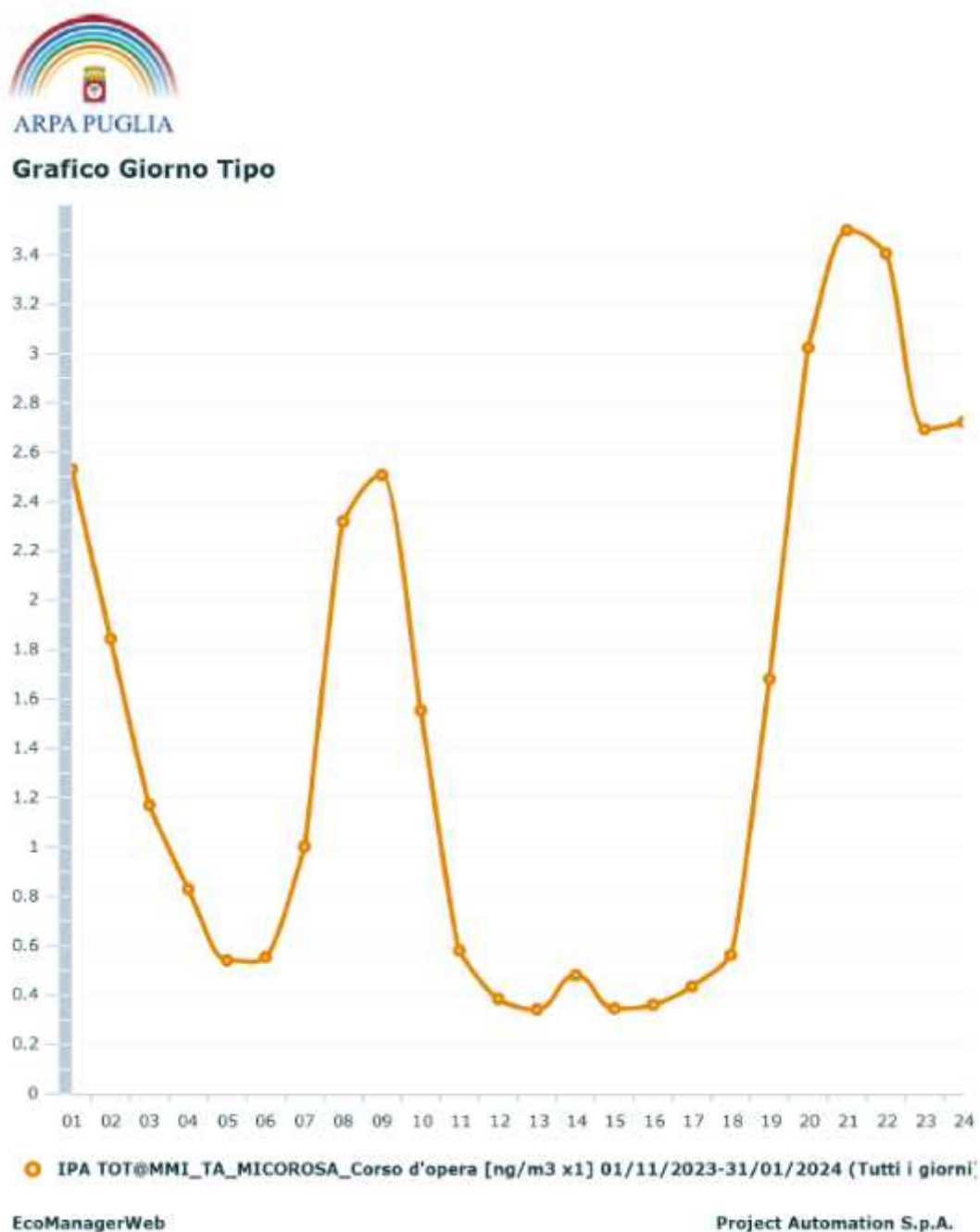
Figura 22: Grafico del giorno tipo per gli idrocarburi policiclici aromatici totali.
