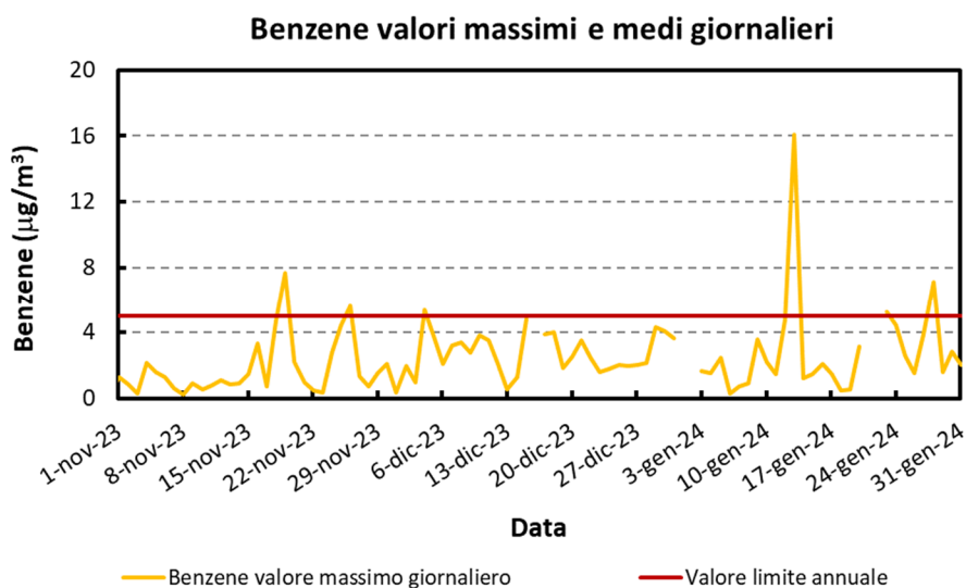
Figura 13: Andamento della concentrazione massima giornaliera di benzene misurata presso il sito oggetto della campagna.
