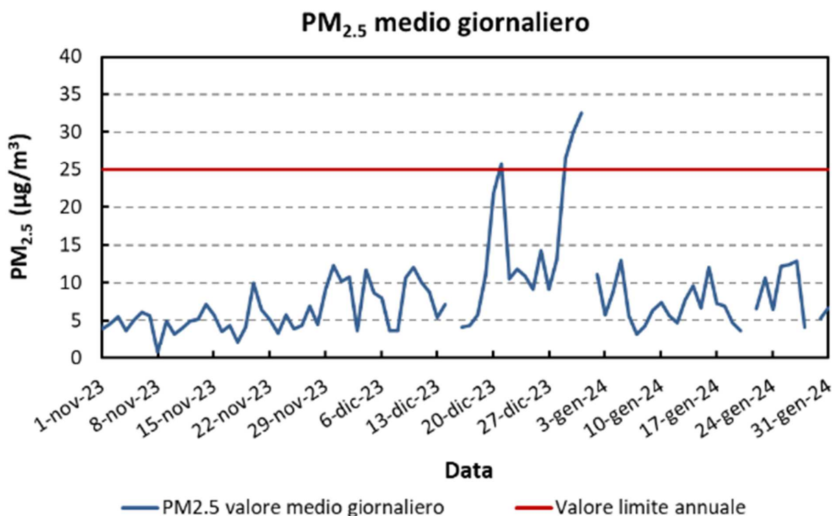
Figura 7: Andamento giornaliero del PM2,5 (µg/m 3 ) misurato presso il sito oggetto della campagna.
