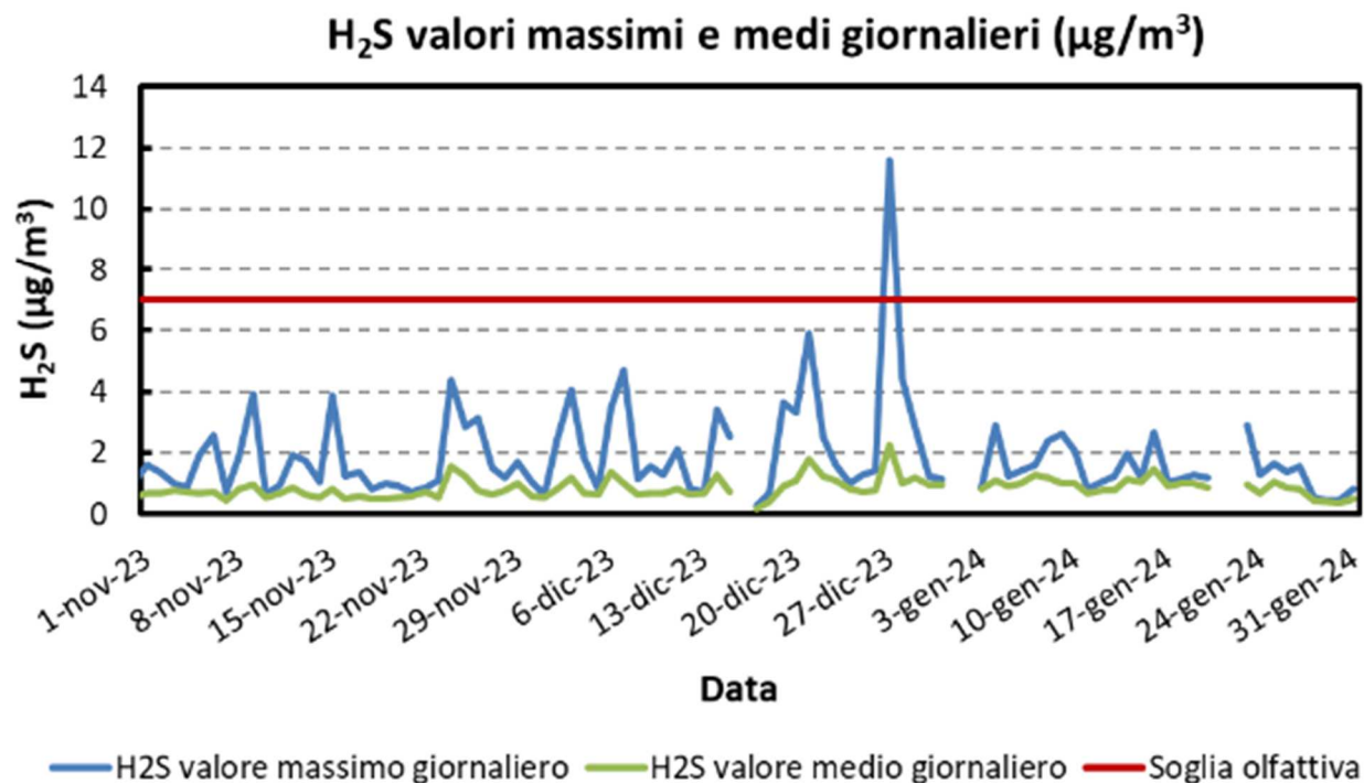
Figura 14: Andamento della concentrazione massima oraria e media giornaliera di H 2 S (µg/m 3 ), misurata presso il sito oggetto della campagna.
