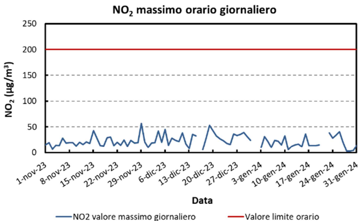
Figura 9: Andamento della concentrazione massima oraria giornaliera per il biossido di azoto (µg/m 3 ) misurata presso il sito oggetto della campagna.
