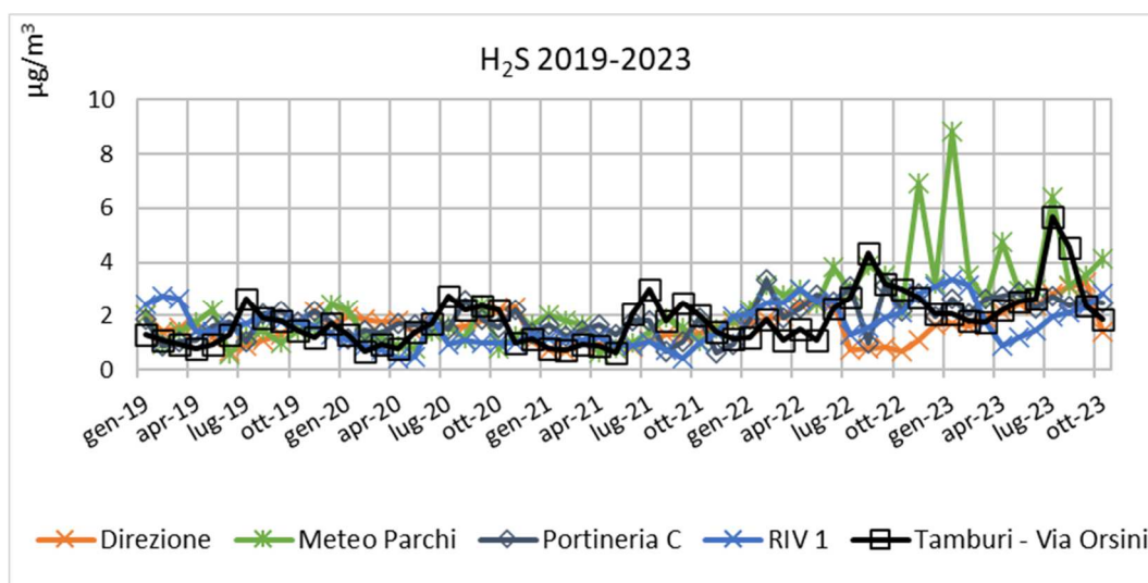
Figura 8 - Andamento dati medi mensili di H 2 S (µg/m 3 ) 2019÷2023 (Rete ADI senza Cokeria)
