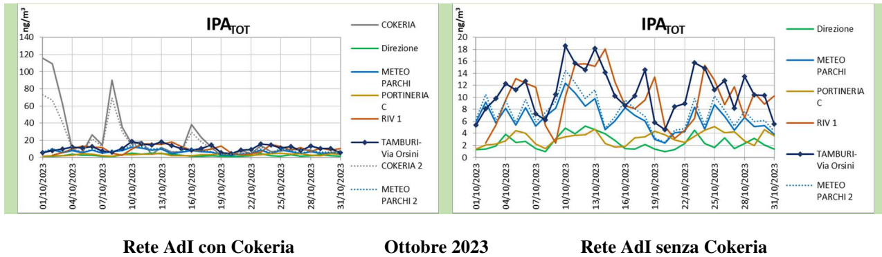
Figura 34 - Livelli di concentrazione di IPA TOT in ng/m 3
