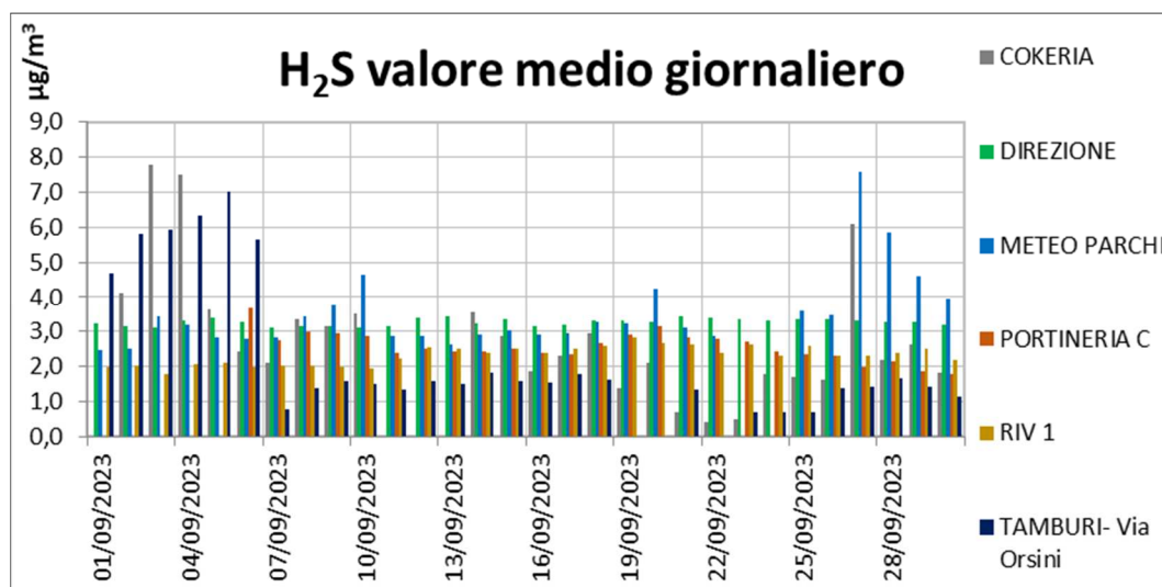
Figura 5 - Valori medi giornalieri H 2 S in µg/m 3 - settembre 2023 (Rete AdI con Cokeria)
