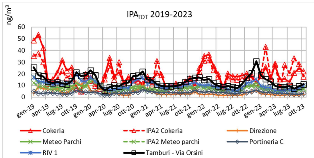
Figura 37 - Livelli medi mensili di concentrazione di IPA TOT 2019 ÷ 2023 in ng/m 3 (Rete ADI con Cokeria)
