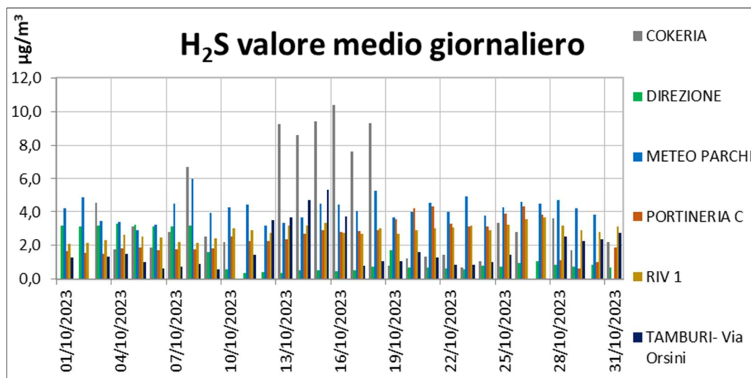
Figura 3 - Livelli medi giornalieri di concentrazione di H 2 S in \mu\text{g}/\text{m}^3 ottobre 2023 (Rete AdI con Cokeria)
