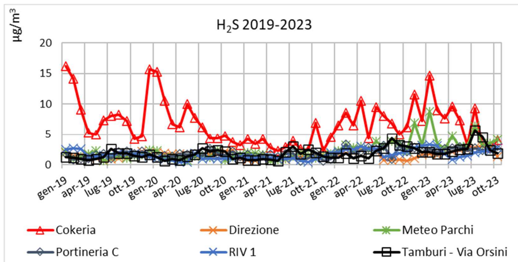
Figura 7 - Andamento dati medi mensili di H 2 S (µg/m 3 ) 2019÷2023 (Rete ADI con Cokeria)
