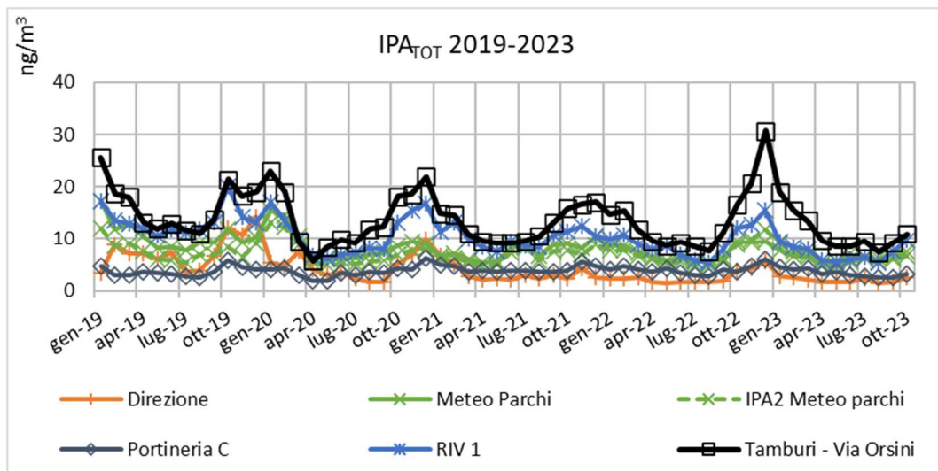
Figura 38 - Livelli medi mensili di concentrazione di IPA TOT 2019 ÷ 2023 in ng/m 3 (Rete ADI senza Cokeria)
