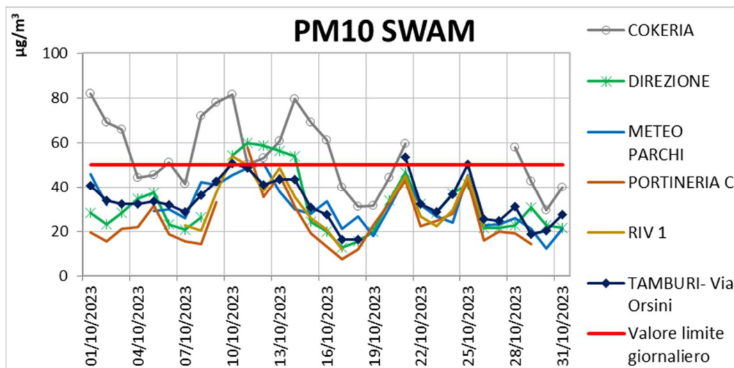
Figura 9 - Livelli di concentrazione ottobre 2023 di PM10 (SWAM) in µg/m 3 (Rete ADI con Cokeria)
