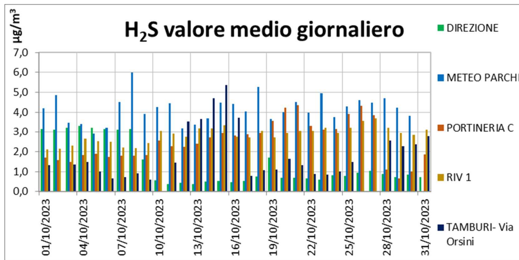
Figura 4 - Livelli medi giornalieri di concentrazione di H 2 S in µg/m 3 ottobre 2023 (Rete AdI senza Cokeria)
