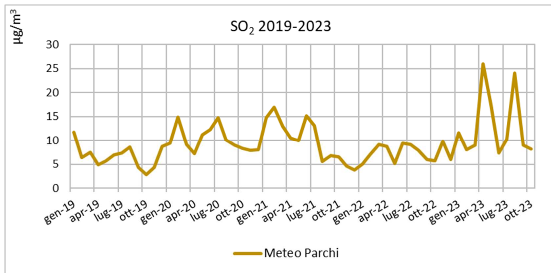
Figura 40 - Livelli medi mensili di concentrazione di SO 2 , 2019-2023 in µg/m 3
