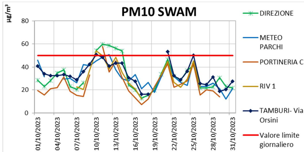
Figura 10 - Livelli di concentrazione ottobre 2023 di PM10 (SWAM) in \mu\text{g}/\text{m}^3 (Rete ADI senza Cokeria)
