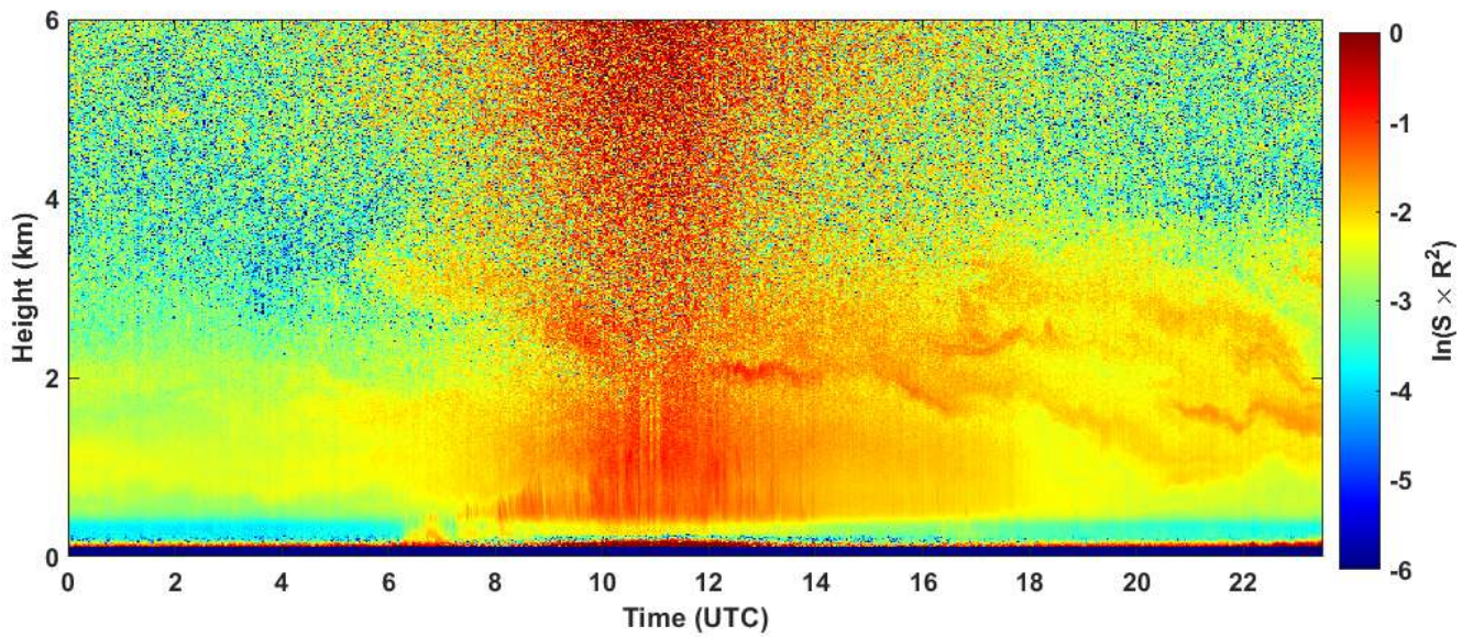
2023-06-22 RCS quick look CHM15k - ILVA LIDAR1 DIREZIONE
