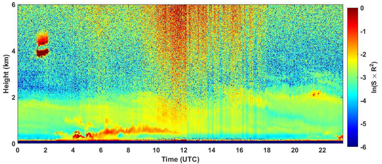
2023-06-10 RCS quick look CHM15k - ILVA LIDAR1 DIREZIONE
