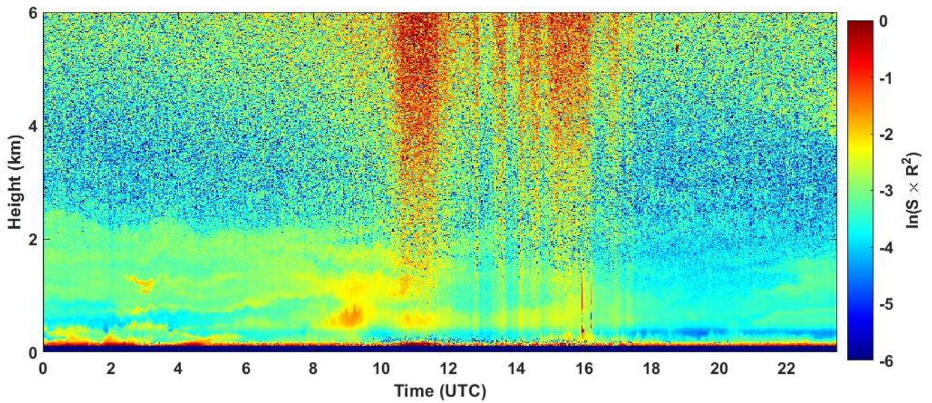
2023-06-04 RCS quick look CHM15k - ILVA LIDAR1 DIREZIONE
