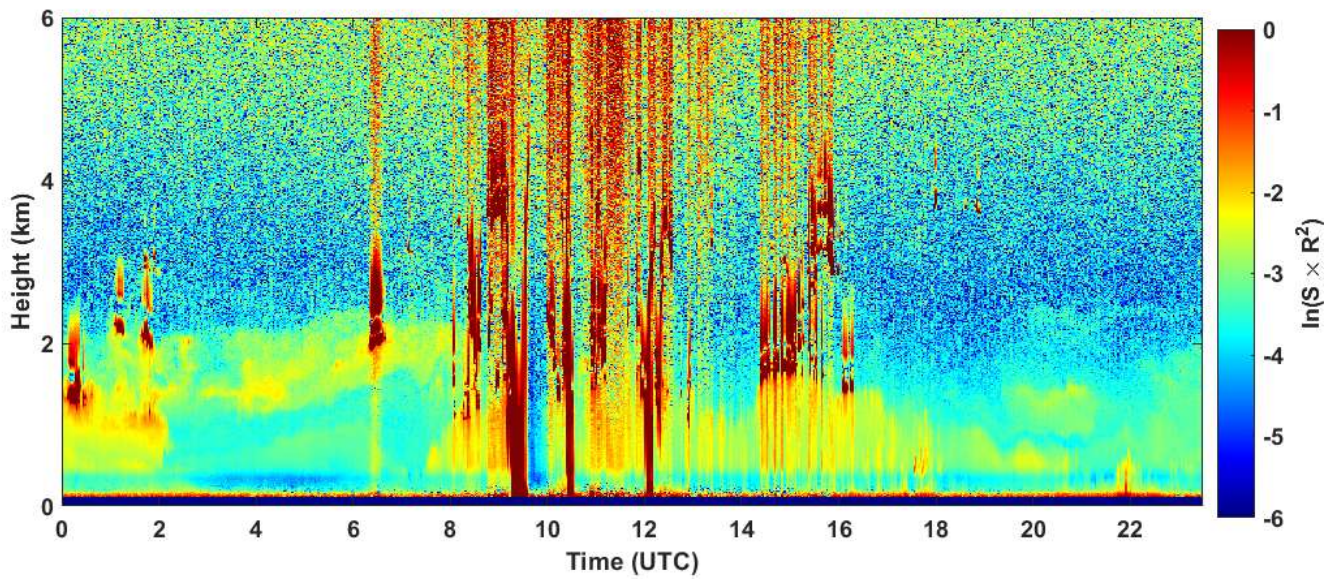
2023-06-12 RCS quick look CHM15k - ILVA LIDAR1 DIREZIONE
