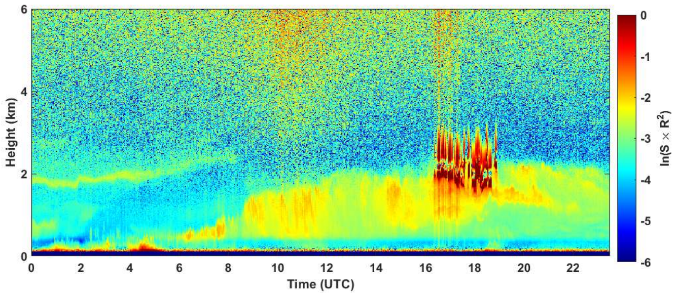
2023-06-08 RCS quick look CHM15k - ILVA LIDAR1 DIREZIONE
