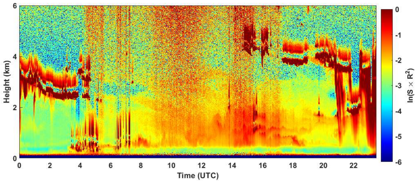
2023-06-06 RCS quick look CHM15k - ILVA LIDAR1 DIREZIONE
