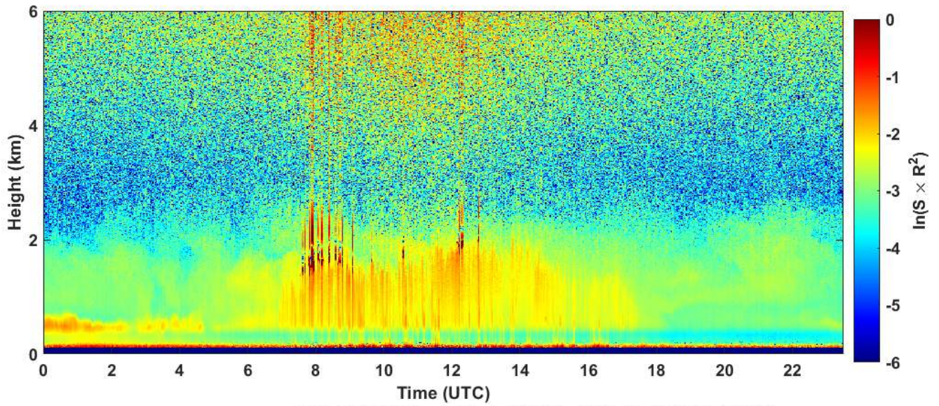
2023-06-18 RCS quick look CHM15k - ILVA LIDAR1 DIREZIONE
