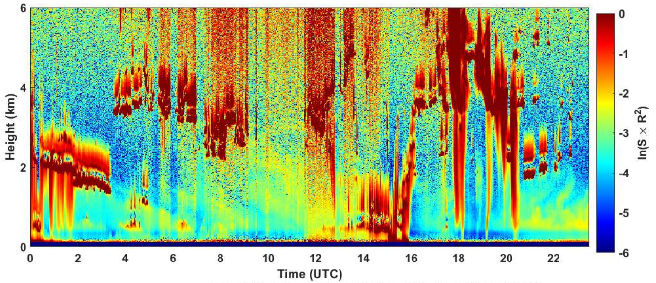
2023-06-16 RCS quick look CHM15k - ILVA LIDAR1 DIREZIONE
