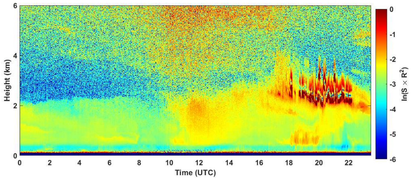
2023-06-28 RCS quick look CHM15k - ILVA LIDAR1 DIREZIONE
