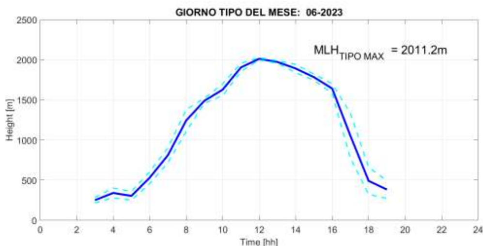
Fig. 2: Giorno tipo del parametro Mixing Layer Height nel mese di GIUGNO 2023, rappresentato mediante media oraria (linea blu continua) e deviazione standard (linee celesti tratteggiate).
