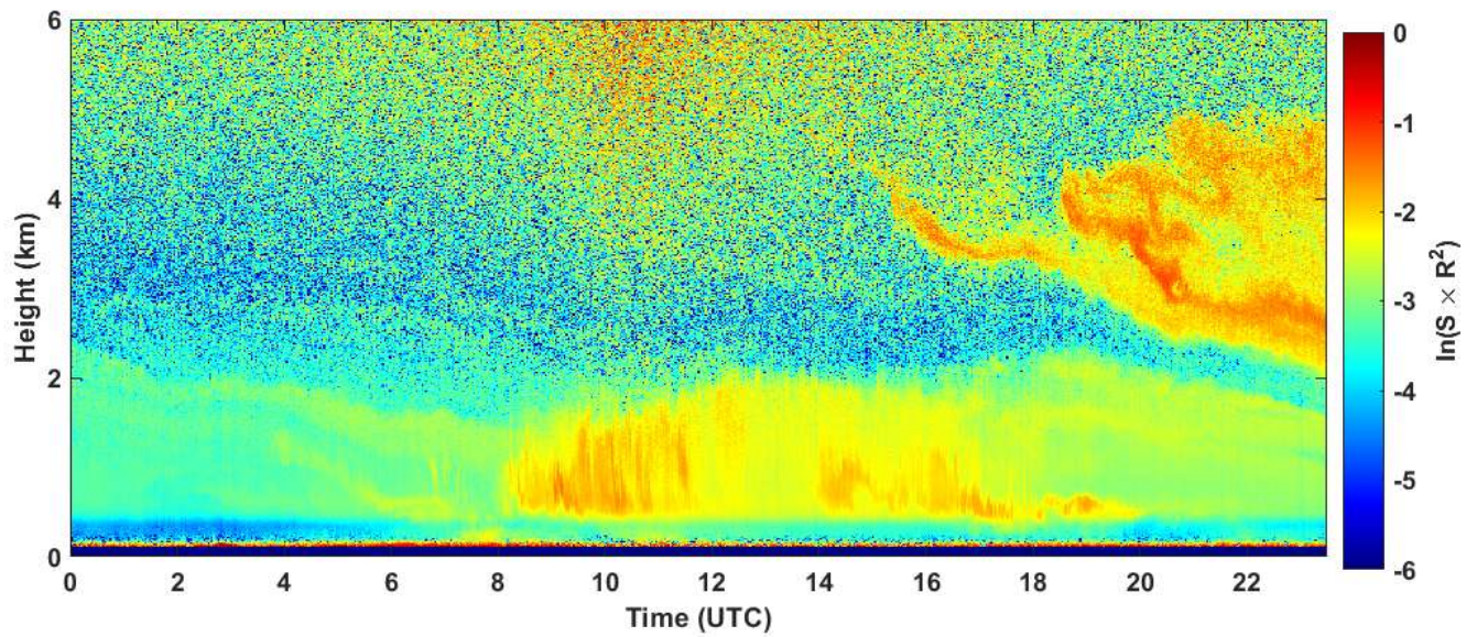
2023-06-20 RCS quick look CHM15k - ILVA LIDAR1 DIREZIONE
