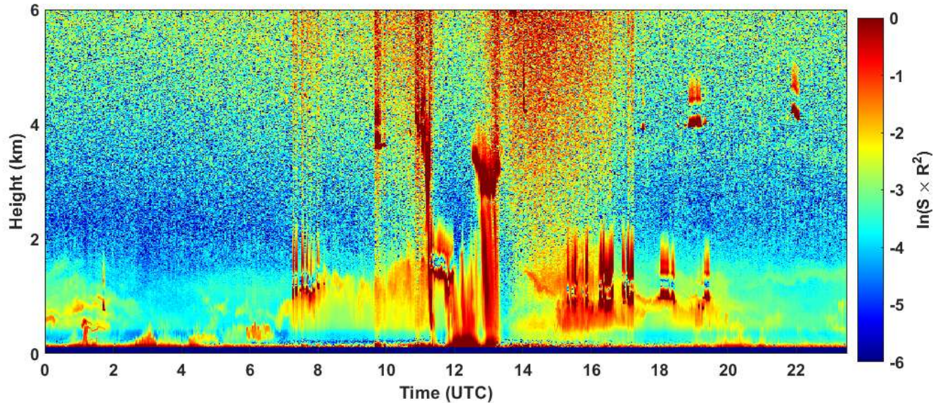
2023-06-02 RCS quick look CHM15k - ILVA LIDAR1 DIREZIONE
