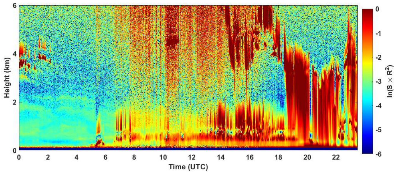
2023-06-14 RCS quick look CHM15k - ILVA LIDAR1 DIREZIONE
