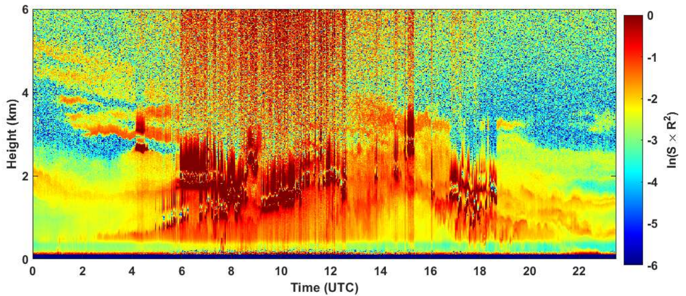
2023-06-30 RCS quick look CHM15k - ILVA LIDAR1 DIREZIONE
