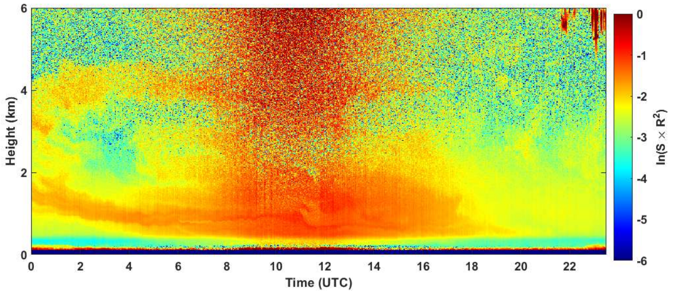
2023-06-24 RCS quick look CHM15k - ILVA LIDAR1 DIREZIONE
