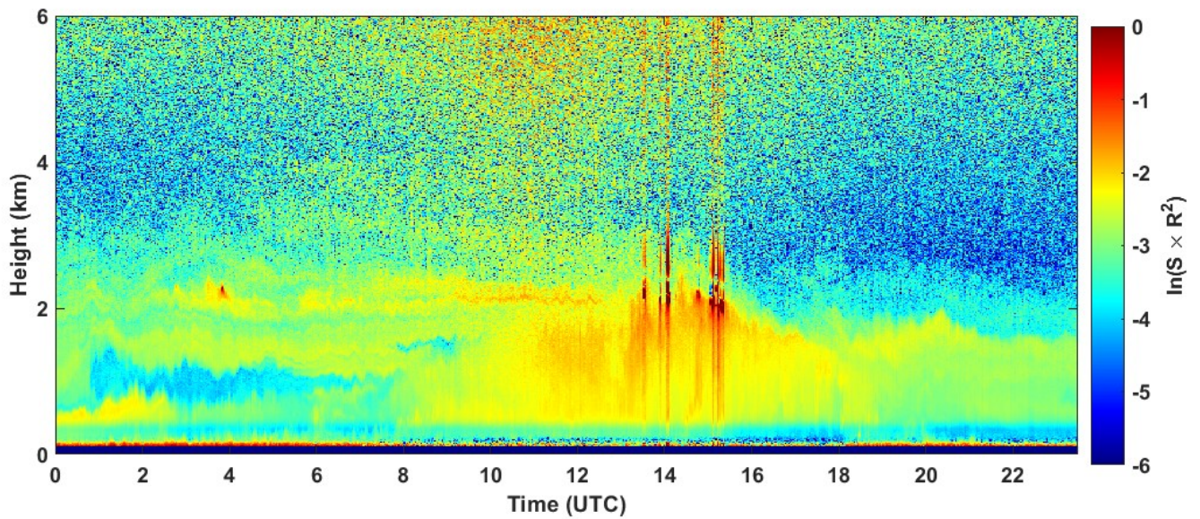
2022-07-28 RCS quick look CHM15k - ILVA LIDAR1 DIREZIONE
