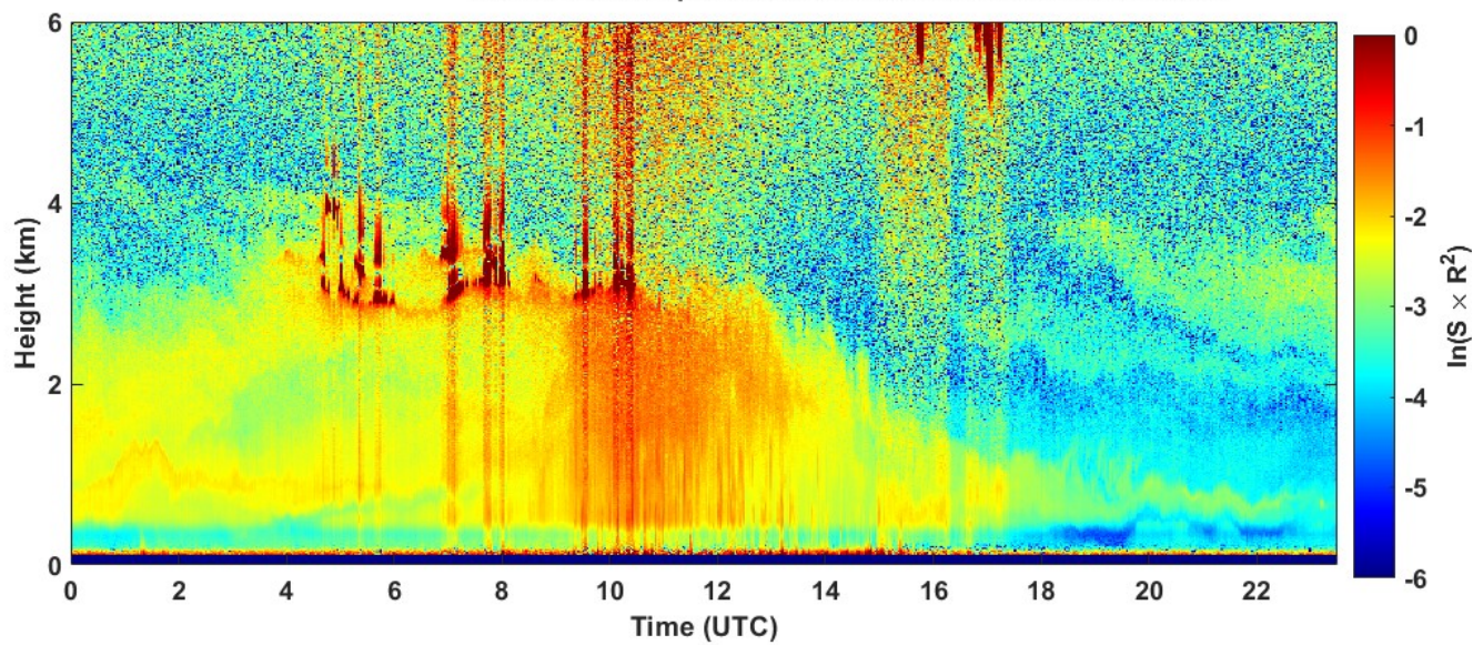
2022-07-06 RCS quick look CHM15k - ILVA LIDAR1 DIREZIONE
