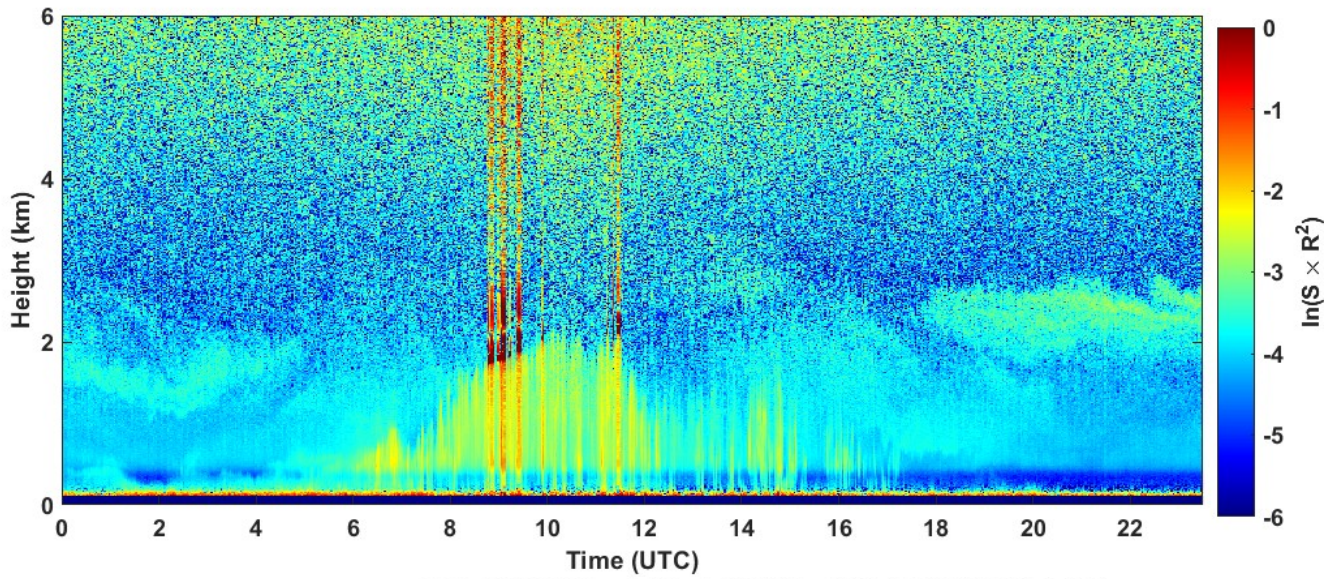
2022-07-12 RCS quick look CHM15k - ILVA LIDAR1 DIREZIONE
