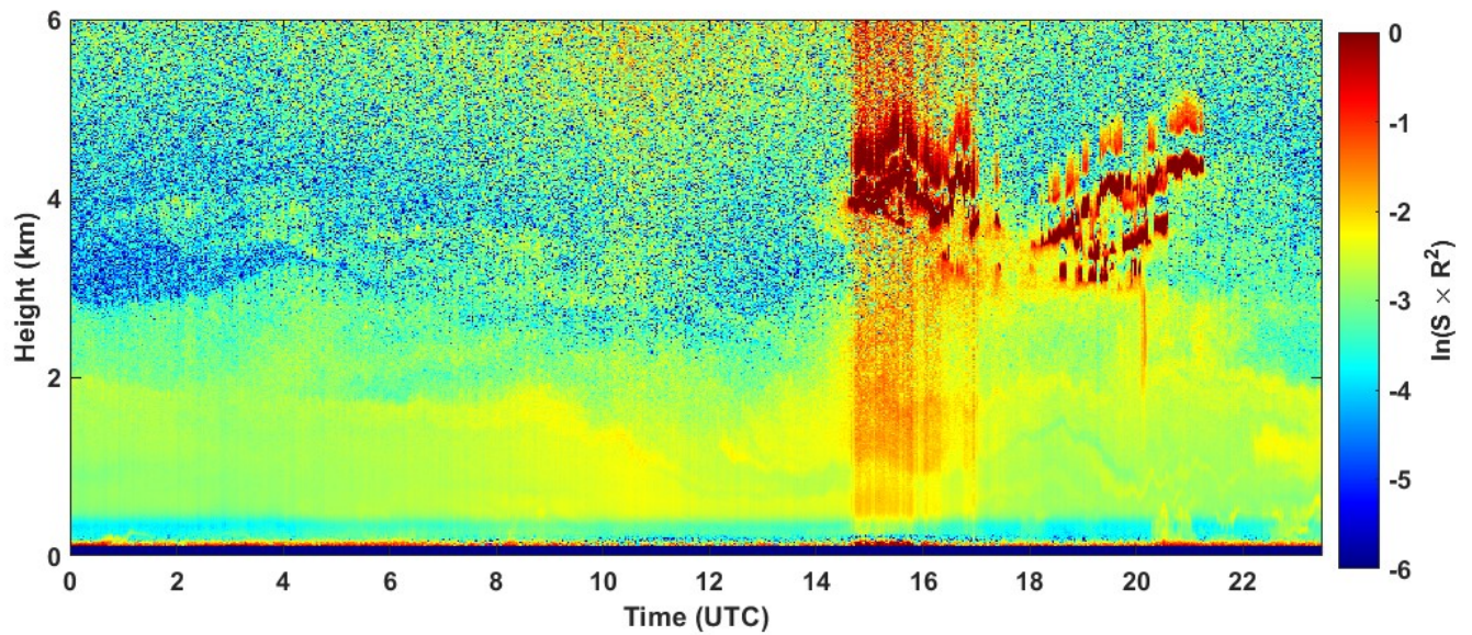
2022-07-26 RCS quick look CHM15k - ILVA LIDAR1 DIREZIONE
