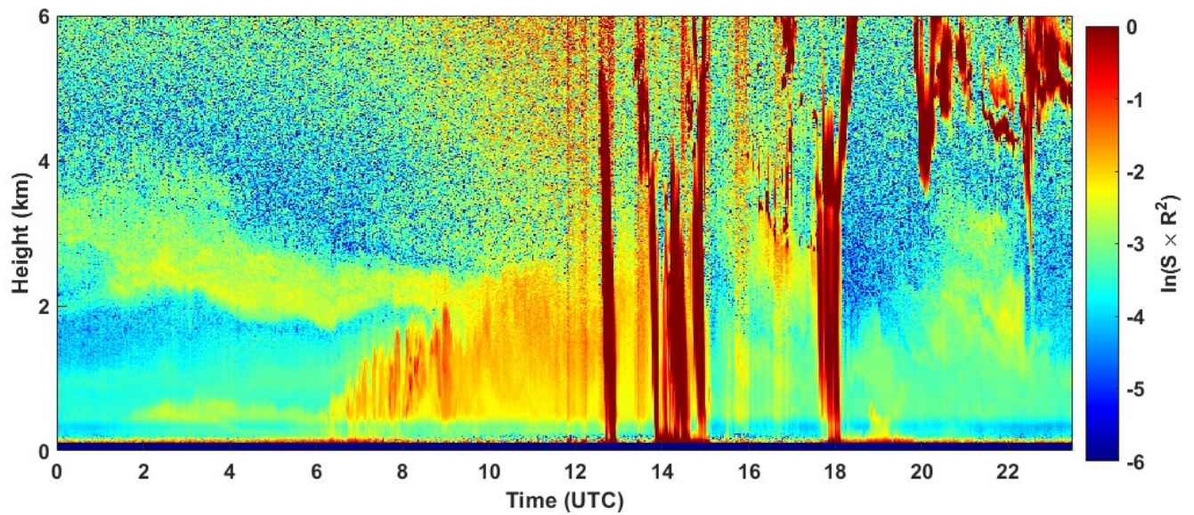
2022-07-08 RCS quick look CHM15k - ILVA LIDAR1 DIREZIONE
