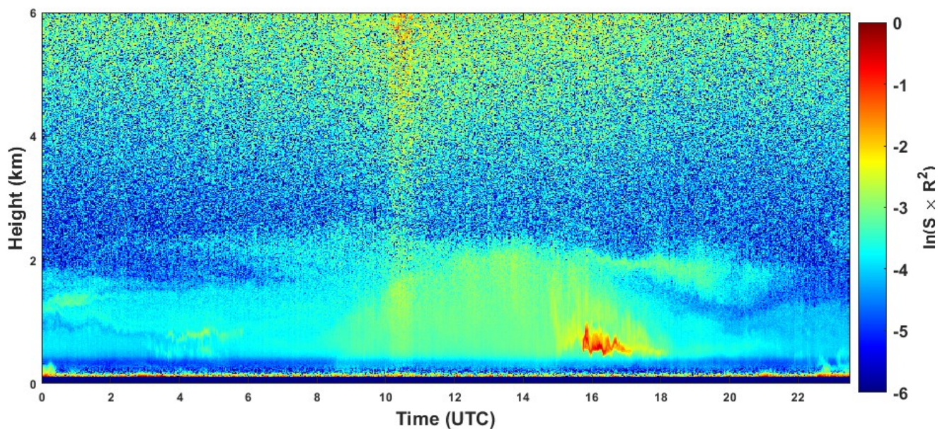
2022-07-16 RCS quick look CHM15k - ILVA LIDAR1 DIREZIONE
