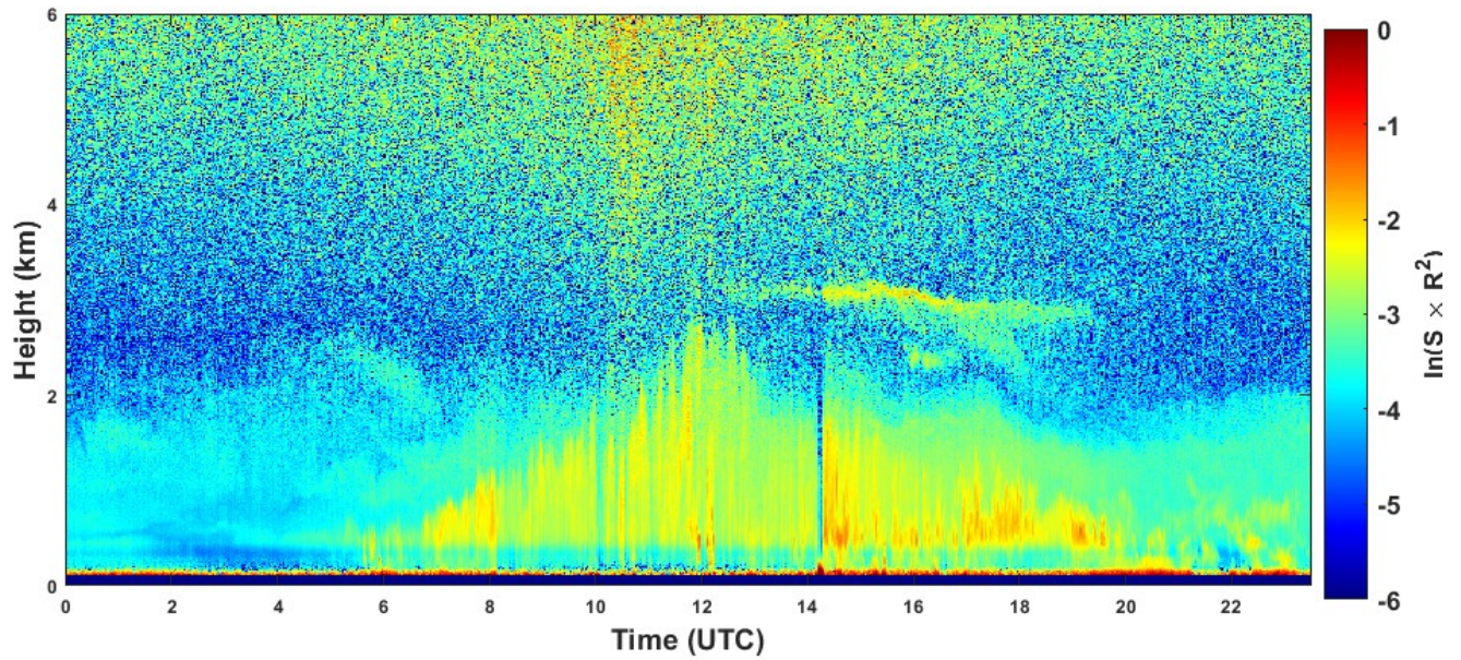
2022-07-20 RCS quick look CHM15k - ILVA LIDAR1 DIREZIONE
