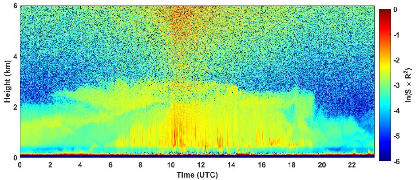
2022-07-04 RCS quick look CHM15k - ILVA LIDAR1 DIREZIONE
