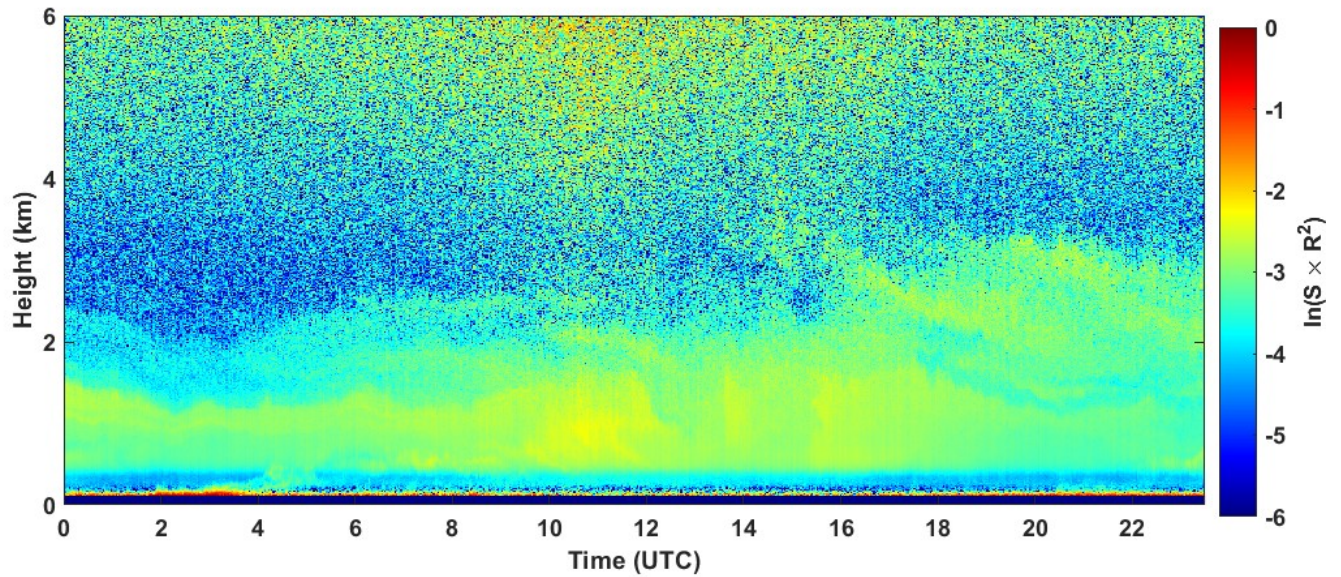
2022-07-30 RCS quick look CHM15k - ILVA LIDAR1 DIREZIONE
