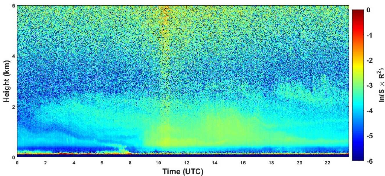
2022-07-16 RCS quick look CHM15k - ILVA LIDAR1 DIREZIONE
