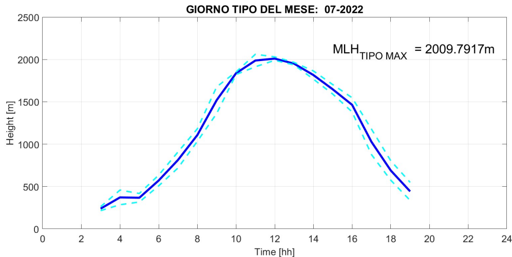
Fig. 2: Giorno tipo del parametro Mixing Layer Height nel mese di LUGLIO 2022, rappresentato mediante media oraria (linea blu continua) e deviazione standard (linee celesti tratteggiate).
