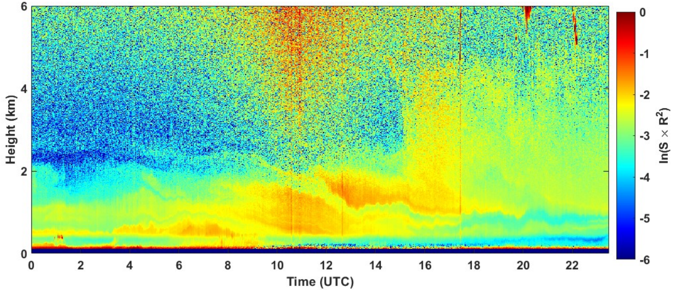
2022-07-02 RCS quick look CHM15k - ILVA LIDAR1 DIREZIONE
