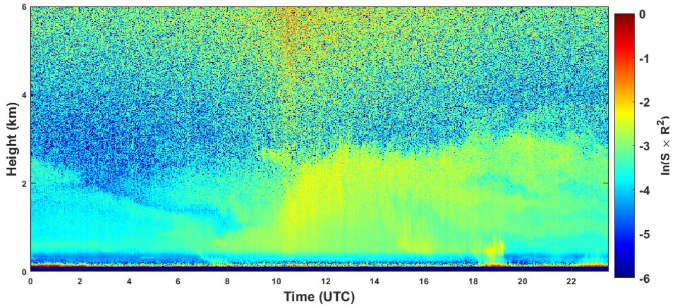
2022-07-18 RCS quick look CHM15k - ILVA LIDAR1 DIREZIONE
