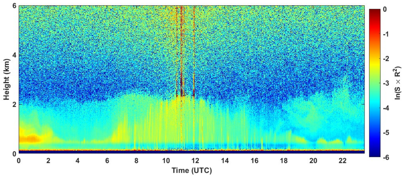
2022-07-10 RCS quick look CHM15k - ILVA LIDAR1 DIREZIONE
