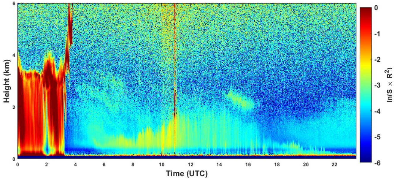
2022-07-14 RCS quick look CHM15k - ILVA LIDAR1 DIREZIONE
