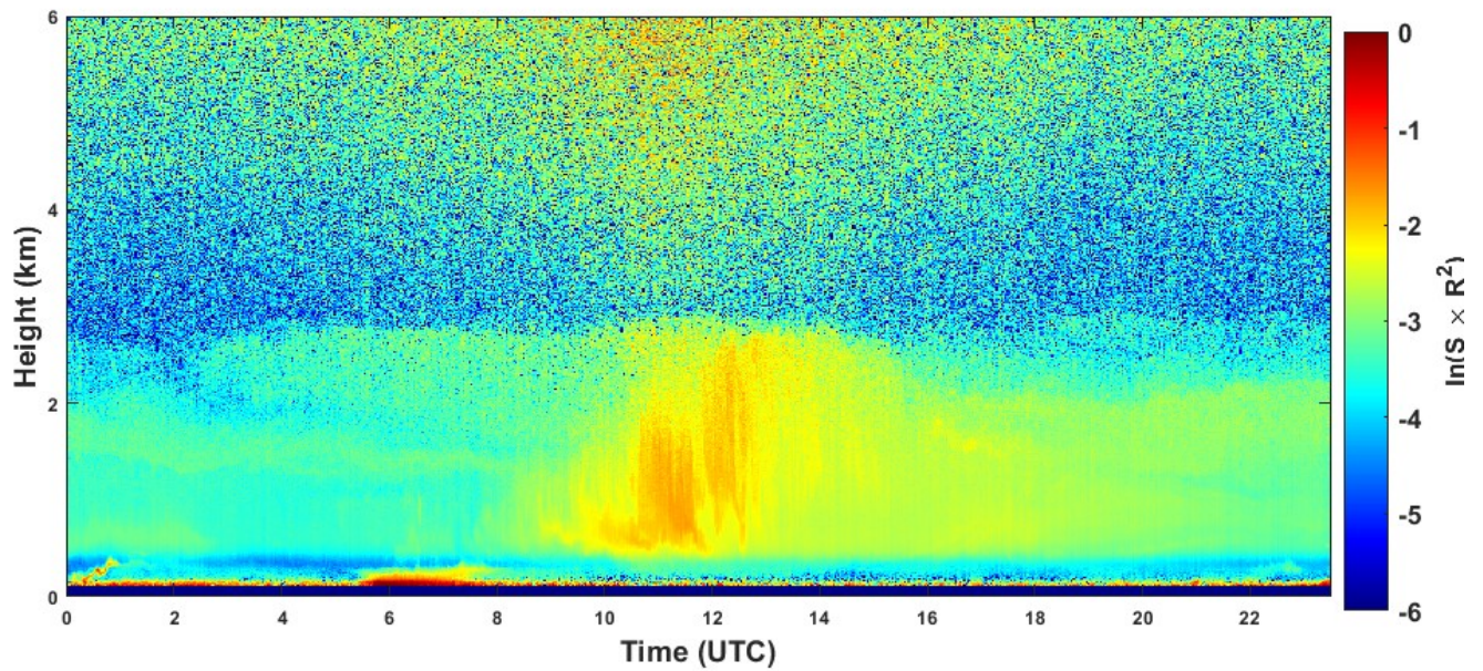
2022-07-22 RCS quick look CHM15k - ILVA LIDAR1 DIREZIONE
