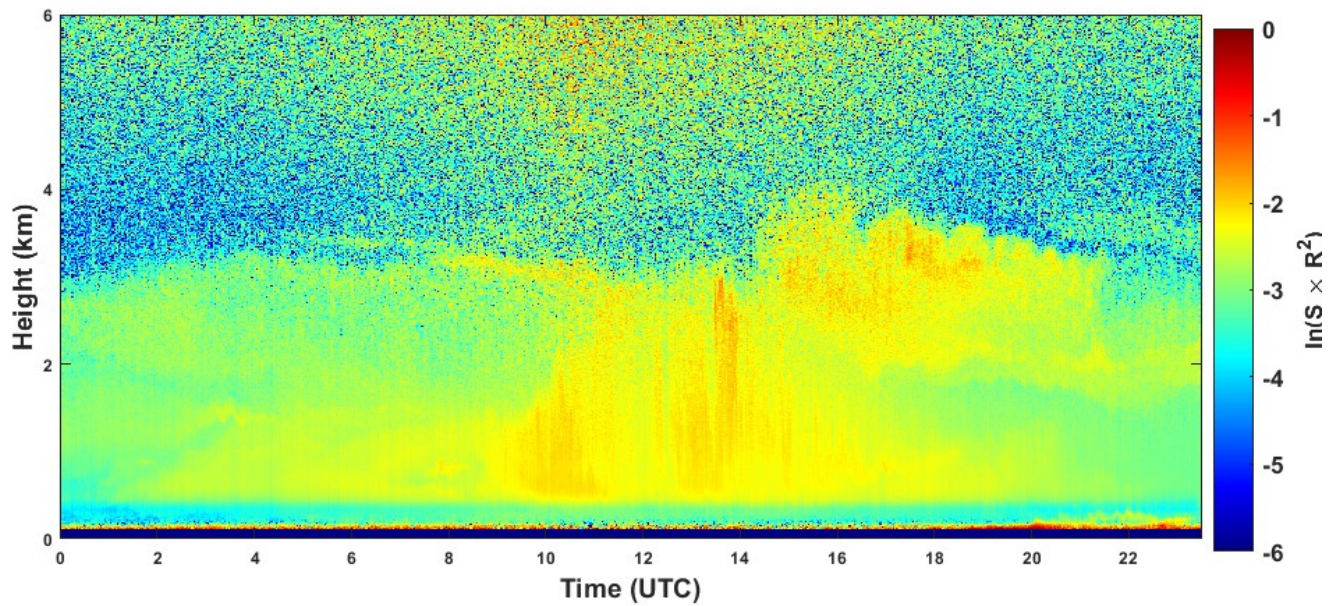
2022-07-24 RCS quick look CHM15k - ILVA LIDAR1 DIREZIONE
