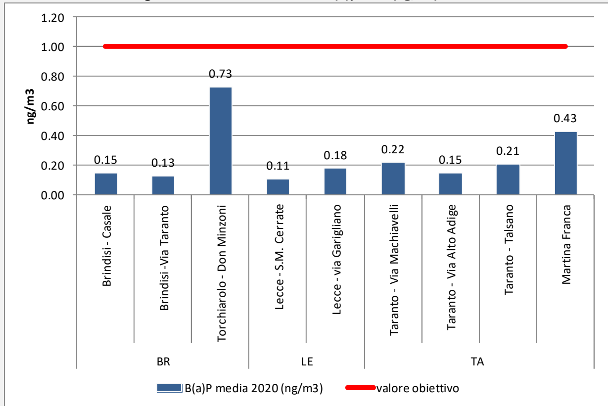
Figura 1: media annuale di Benzo(a)pirene (ng/m 3 ) - 2020
