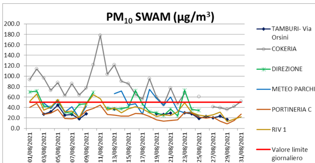
Figura 10 Livelli di concentrazione Agosto 2021 di PM_{10} (SWAM) in \mu g/m^3
