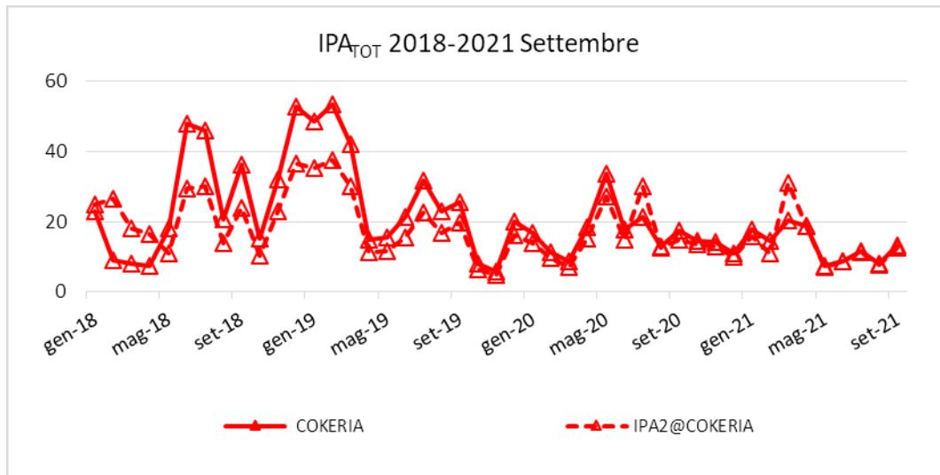
Figura 35 Livelli medi mensili di concentrazione di IPA TOT 2018-Settembre 2021 Cokeria in ng/m 3
