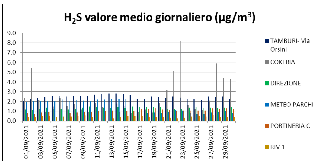
Figura 2 Livelli medi giornalieri di concentrazione di \text{H}_2\text{S} in \mu\text{g}/\text{m}^3 Settembre 2021 (Rete AdI con Cokeria)
