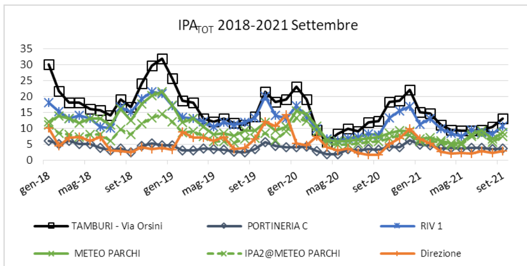
Figura 34 Livelli medi mensili di concentrazione di IPA_{TOT} 2018-Settembre 2021 in ng/m^3 (Rete ADI senza Cokeria)
