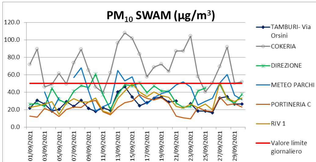
Figura 9 Livelli di concentrazione Settembre 2021 di PM_{10} (SWAM) in \mu g/m^3
