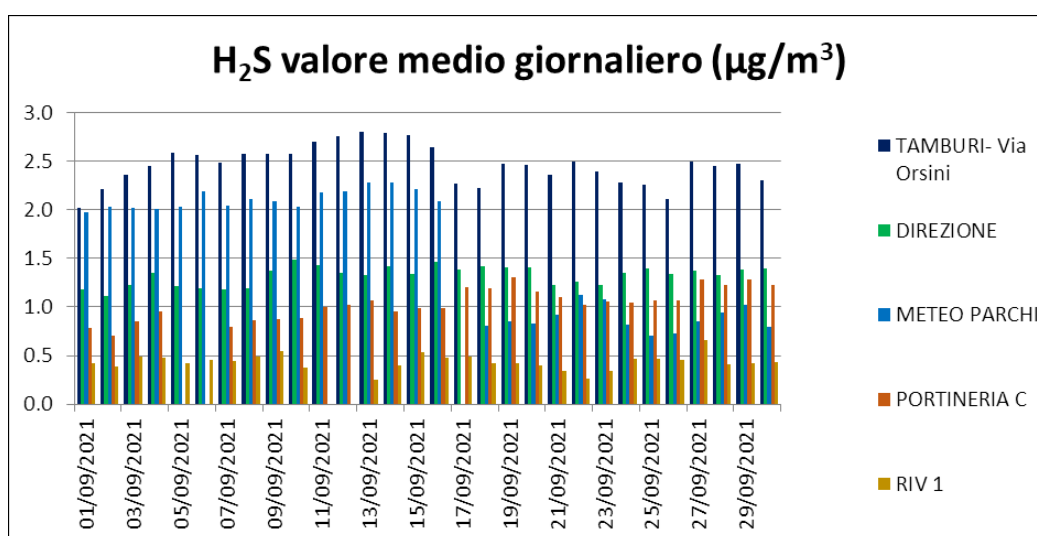
Figura 3 Livelli medi giornalieri di concentrazione di \text{H}_2\text{S} in \mu\text{g}/\text{m}^3 Settembre 2021 (Rete AdI senza Cokeria)
