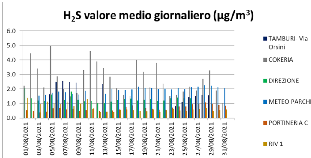
Figura 4 valori medi giornalieri H_2S in \mu g/m^3 - Agosto 2021 (Rete AdI con Cokeria)
