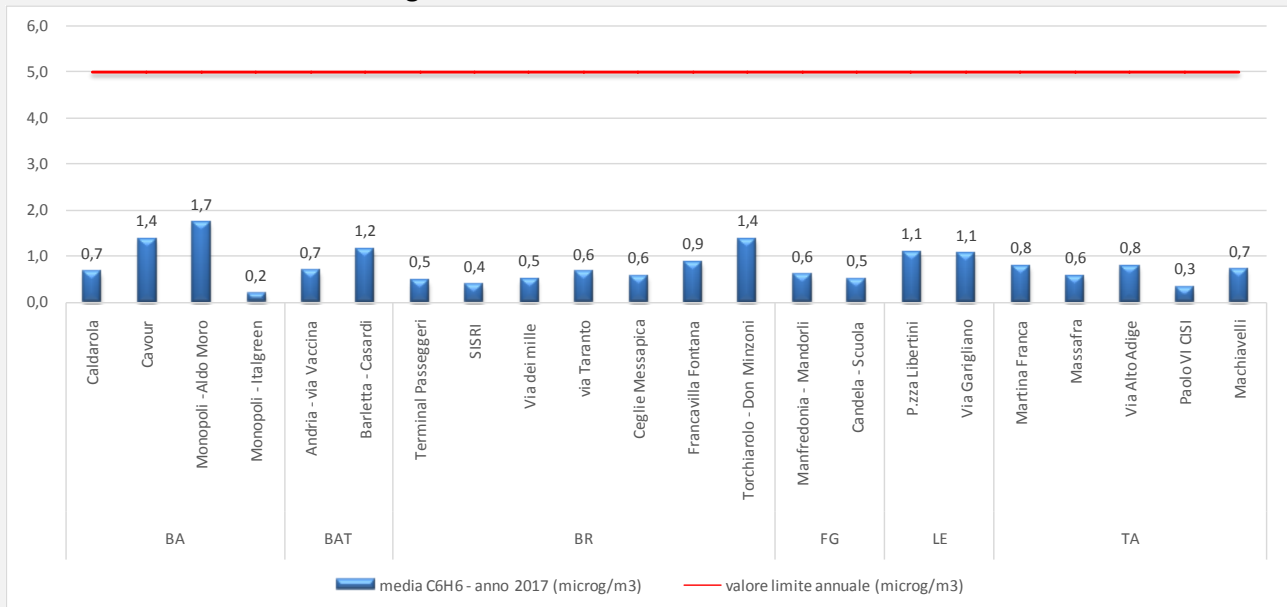
Fig. 1 - Valori medi annui di benzene - 2017
