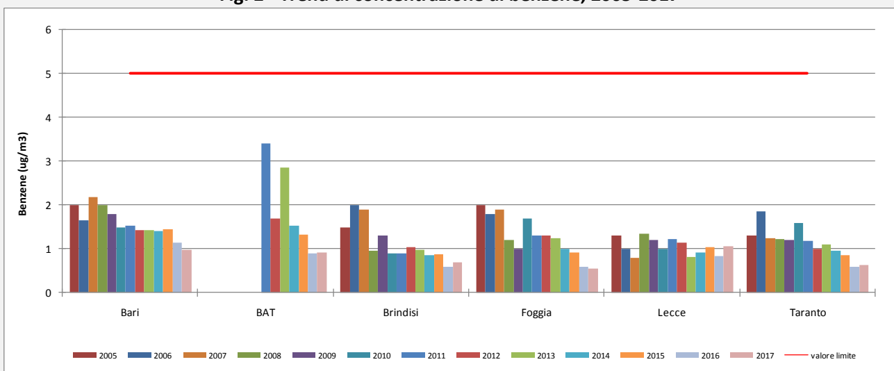
Fig. 2 - Trend di concentrazione di benzene, 2005-2017
