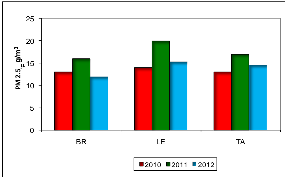
Figura 2: trend di concentrazione di PM 2.5
