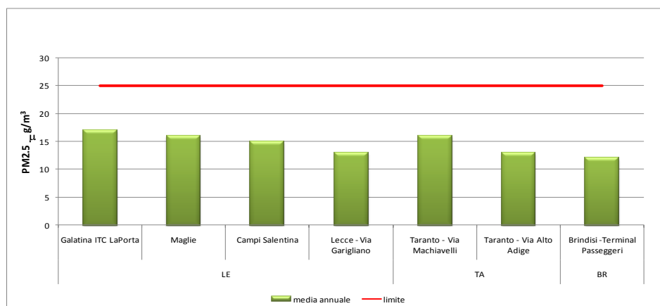
Figura 1: valori medi annui di PM 2.5
