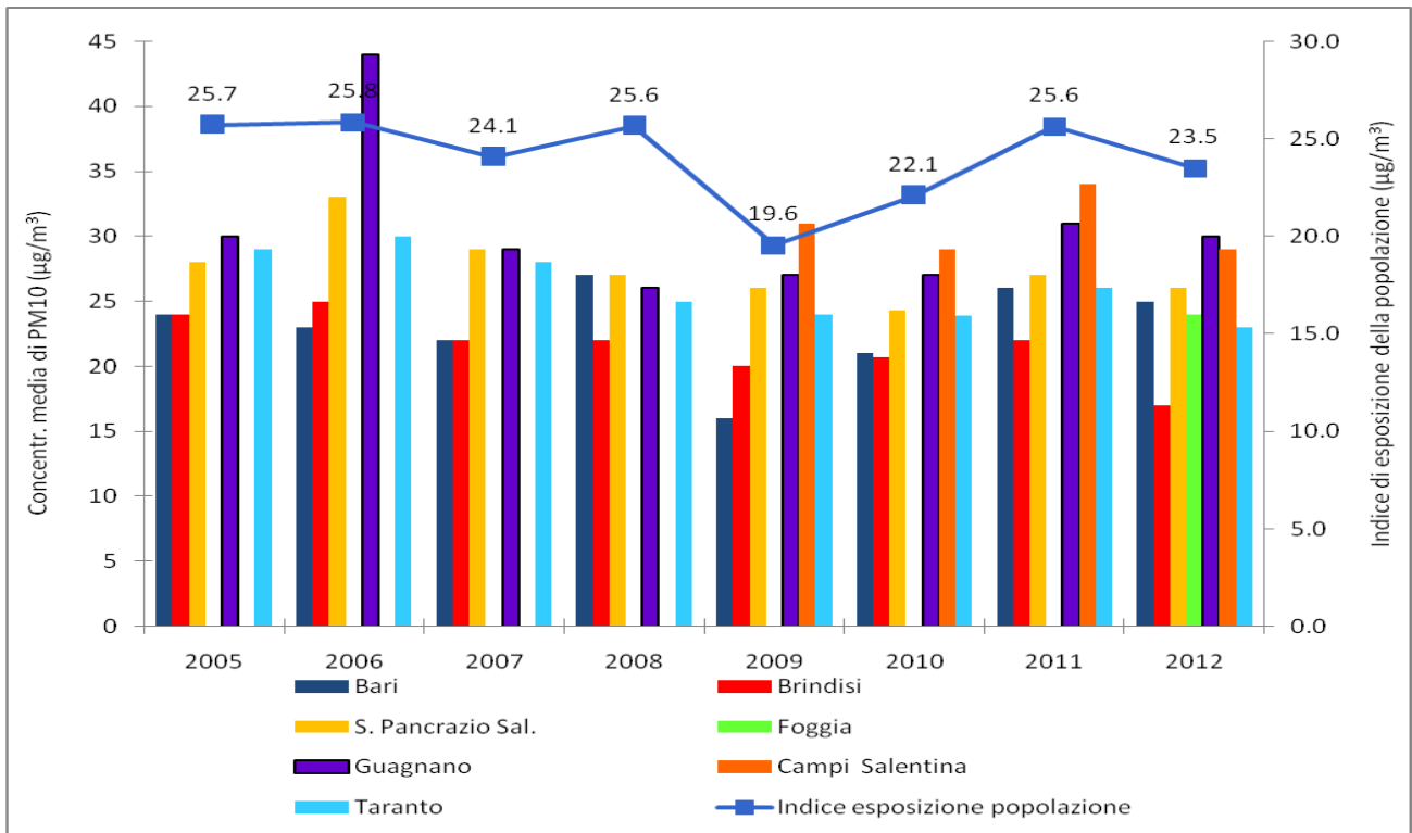
Grafico 2. Concentrazione media di PM10 ( \mu\text{g}/\text{m}^3 ) nei comuni coperti dall'indagine e Indice di esposizione della popolazione generale. Anni 2005-2012
