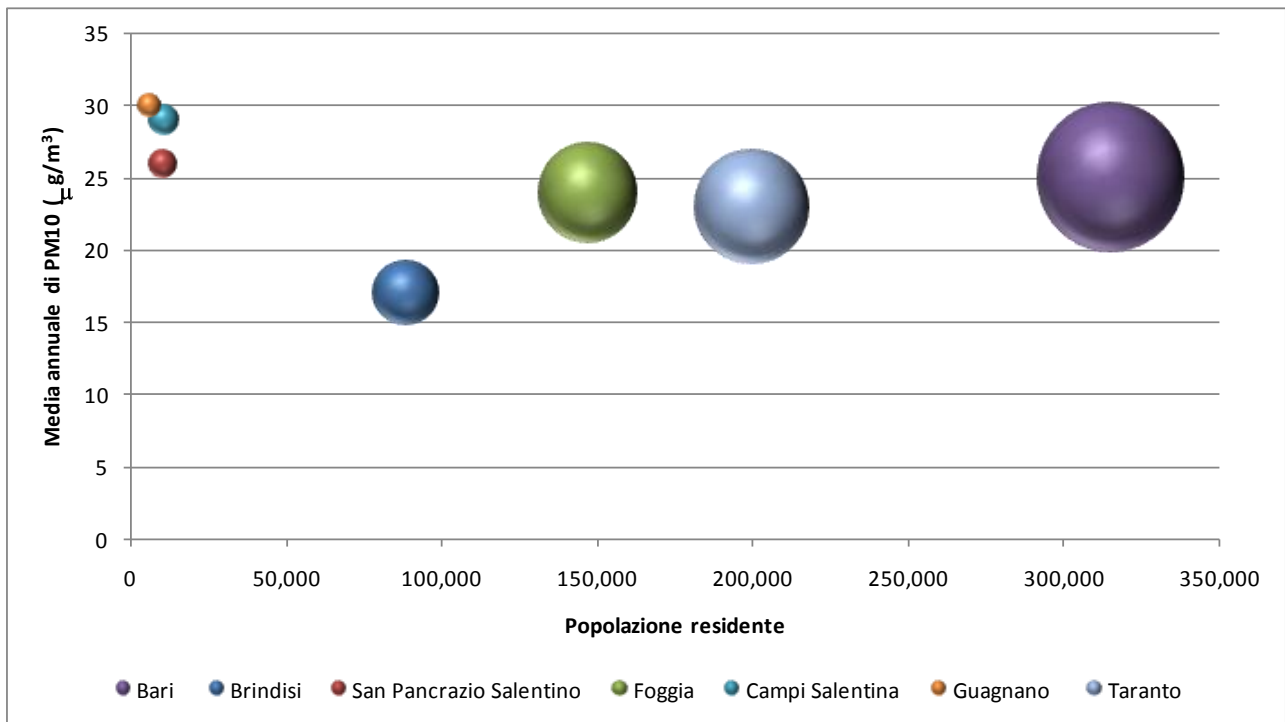
Grafico 1 – Esposizione della popolazione al PM10 ( \mu\text{g}/\text{m}^3 ) nei comuni coperti dall'indagine. Anno 2012
