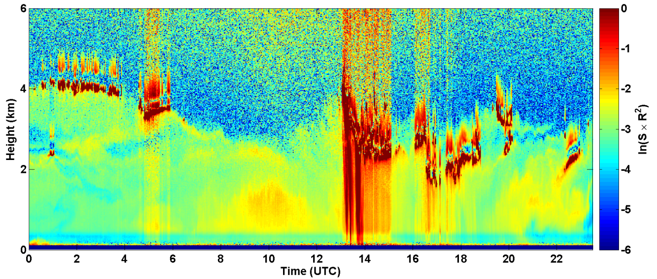
2017-05-20 RCS quick look CHM15k - ILVA LIDAR1 DIREZIONE
