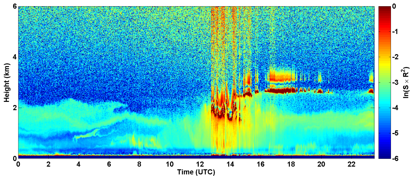
2017-05-02 RCS quick look CHM15k - ILVA LIDAR1 DIREZIONE
