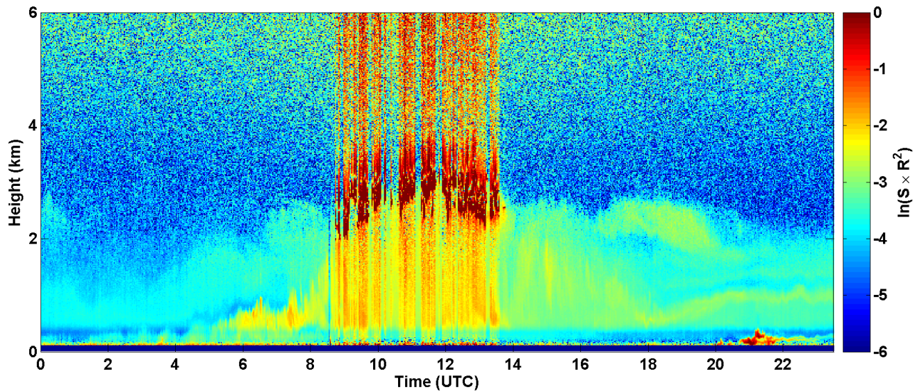
2017-05-30 RCS quick look CHM15k - ILVA LIDAR1 DIREZIONE
