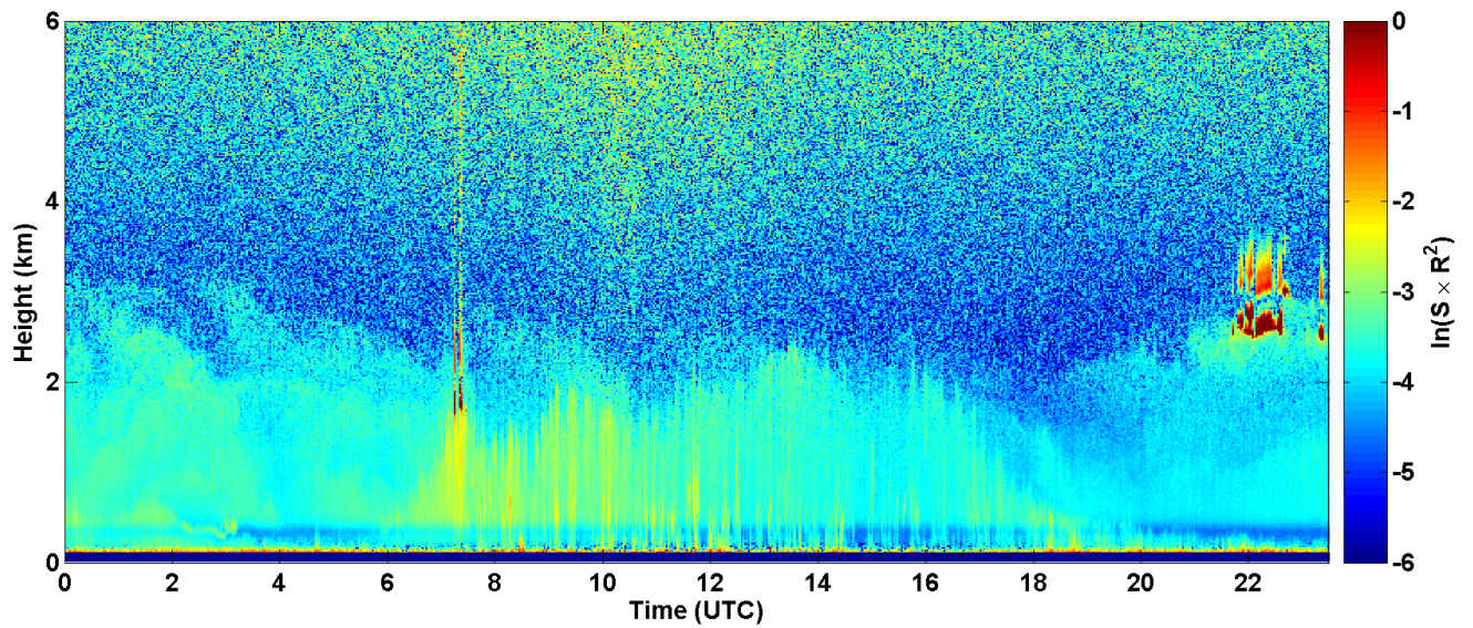
2017-05-28 RCS quick look CHM15k - ILVA LIDAR1 DIREZIONE
