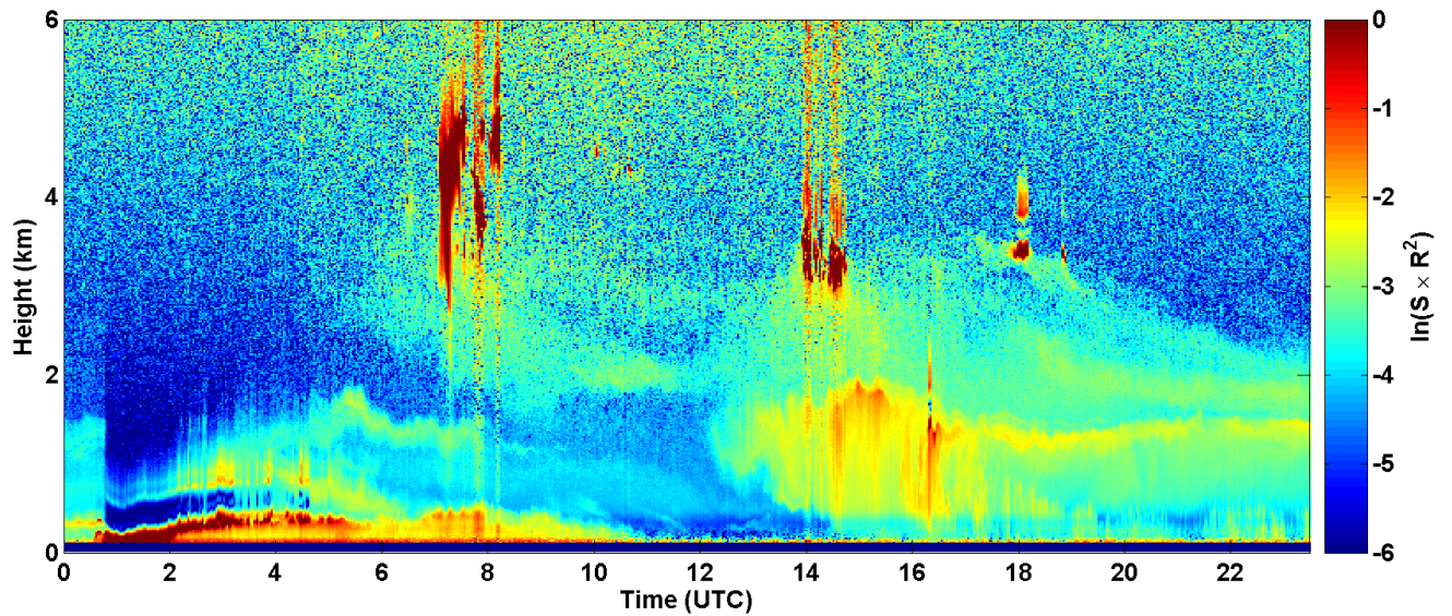
2017-05-06 RCS quick look CHM15k - ILVA LIDAR1 DIREZIONE
