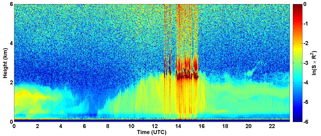
2017-05-14 RCS quick look CHM15k - ILVA LIDAR1 DIREZIONE
