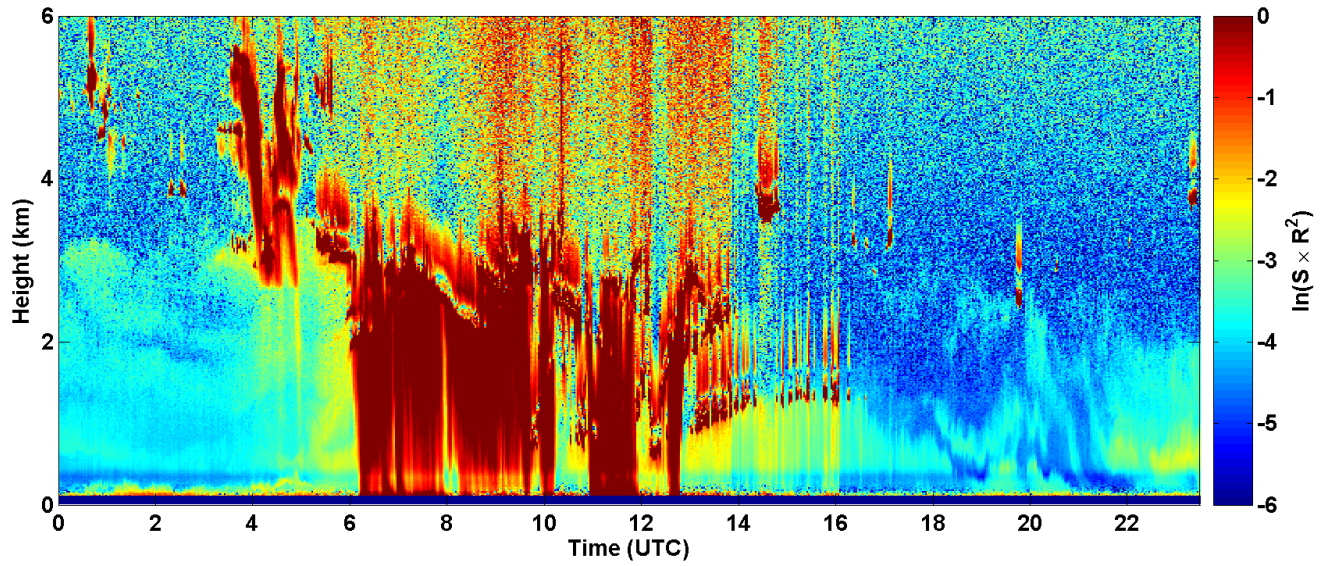
2017-05-26 RCS quick look CHM15k - ILVA LIDAR1 DIREZIONE
