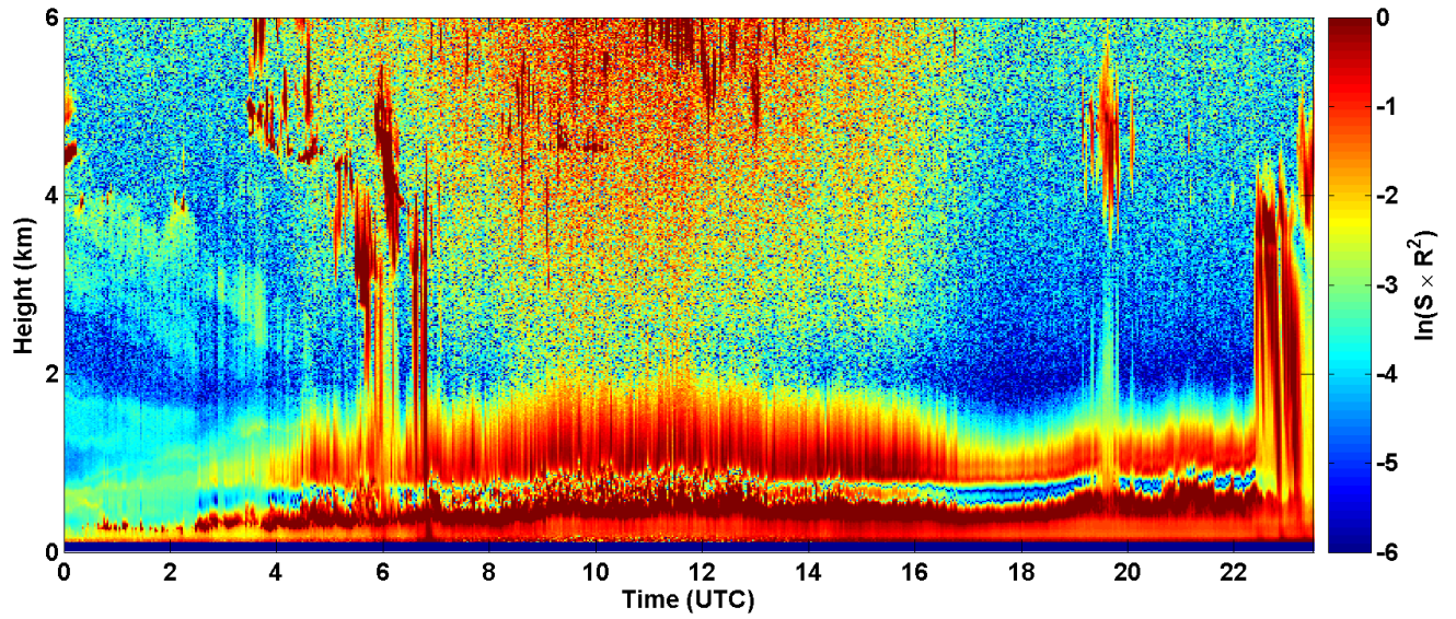
2017-05-12 RCS quick look CHM15k - ILVA LIDAR1 DIREZIONE
