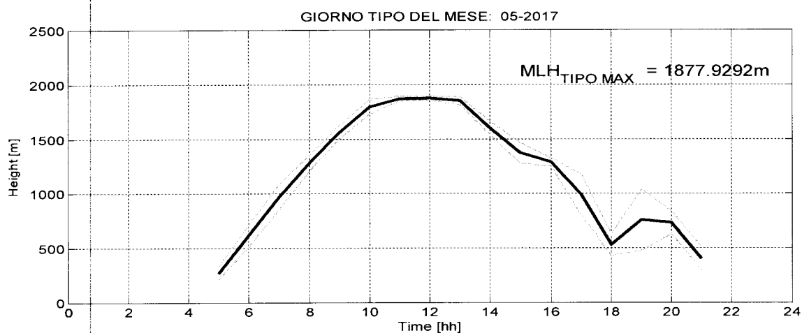
Fig. 2: Giorno tipo del parametro Mixing Layer Height nel mese di MAGGIO 2017, rappresentato mediante media oraria (linea blu continua), e quartili corrispondenti ad una deviazione standard (linee celesti tratteggiate).
