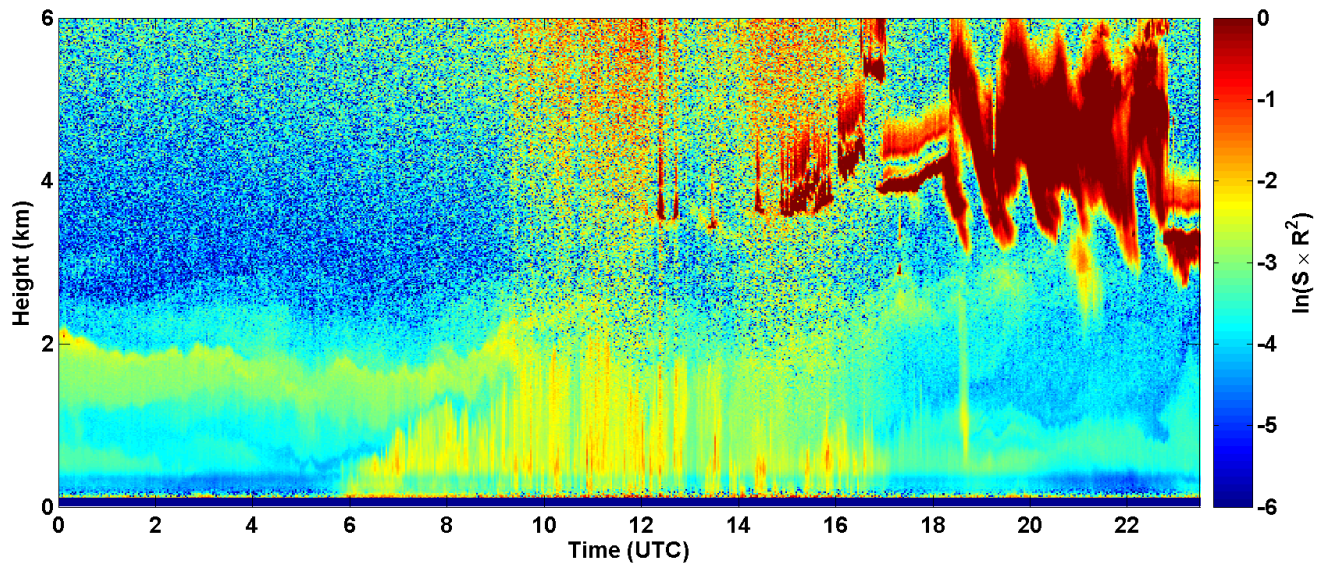
2017-05-16 RCS quick look CHM15k - ILVA LIDAR1 DIREZIONE
