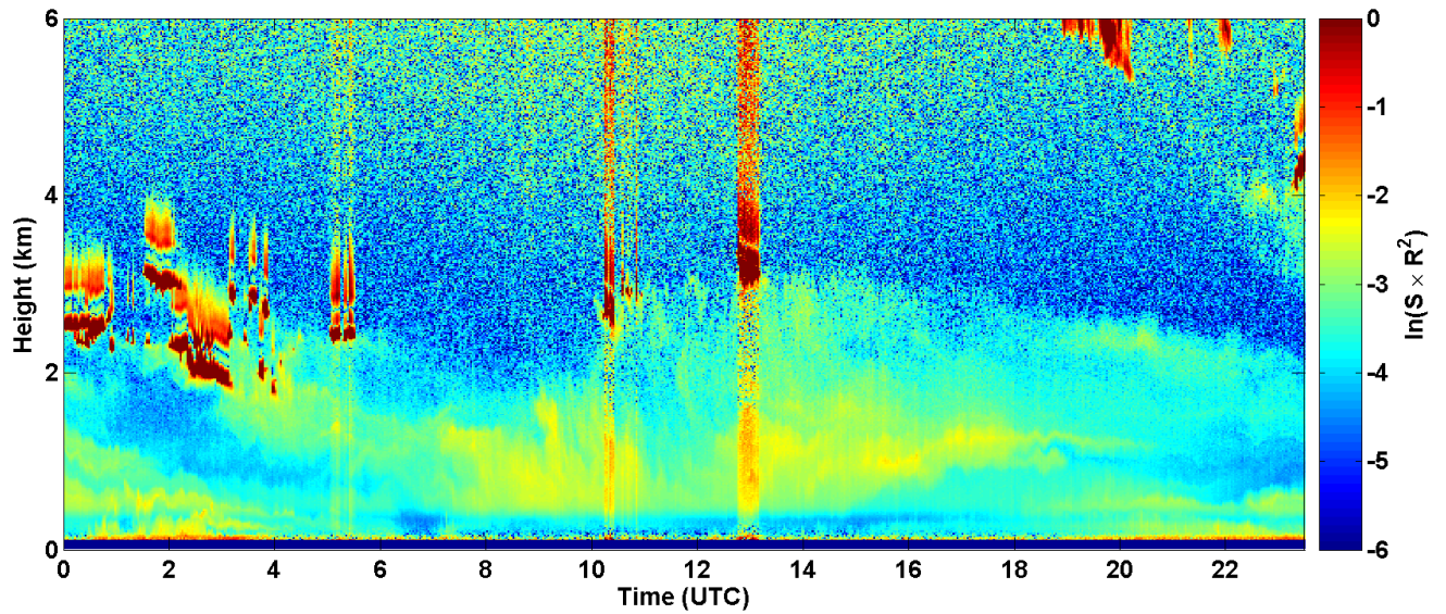
2017-05-10 RCS quick look CHM15k - ILVA LIDAR1 DIREZIONE
