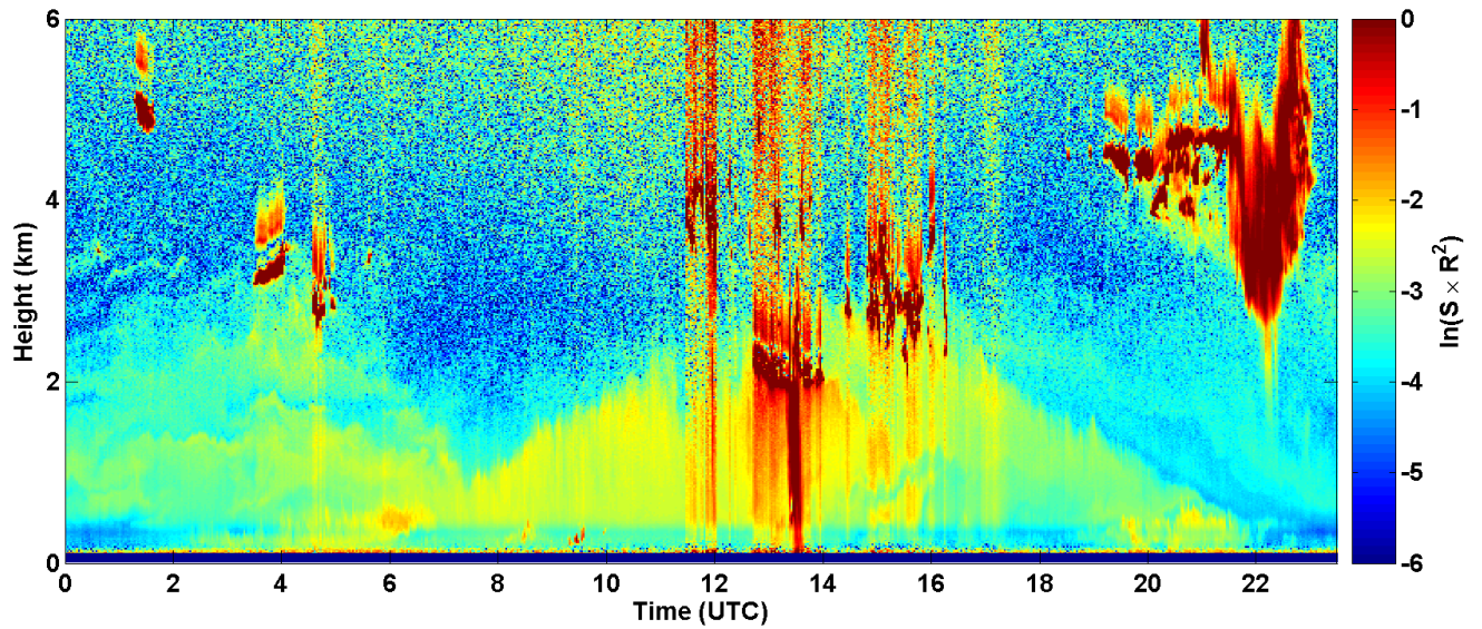
2017-05-24 RCS quick look CHM15k - ILVA LIDAR1 DIREZIONE
