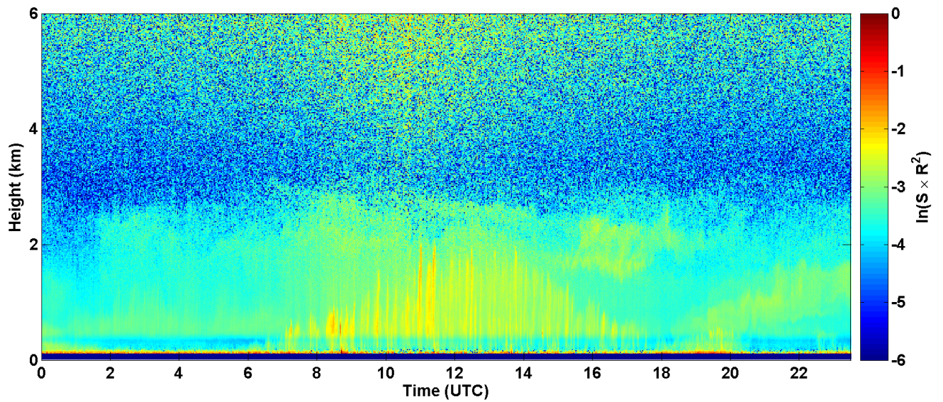
2017-05-22 RCS quick look CHM15k - ILVA LIDAR1 DIREZIONE
