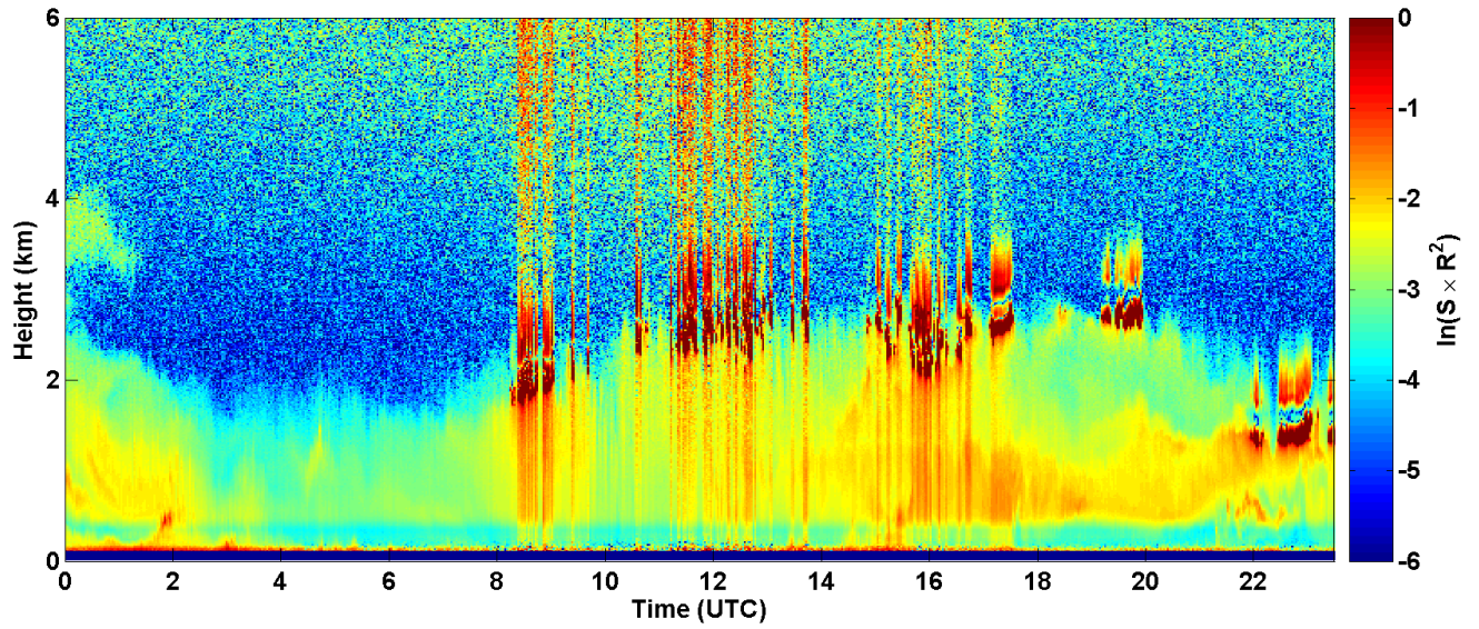
2017-05-08 RCS quick look CHM15k - ILVA LIDAR1 DIREZIONE
