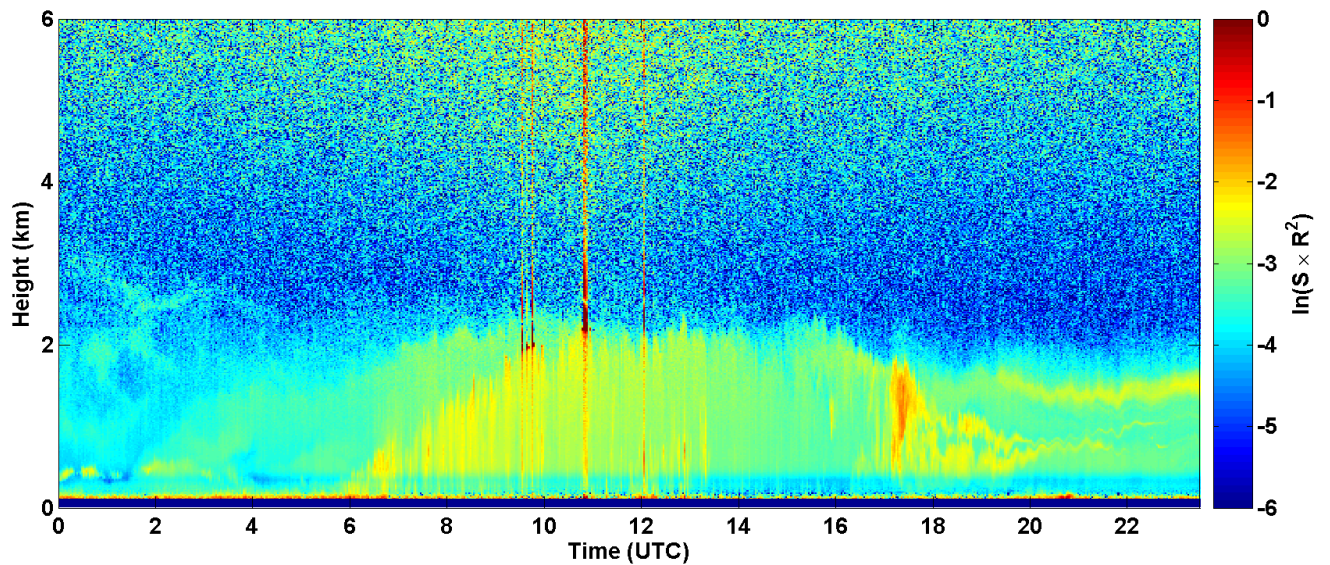
2017-05-18 RCS quick look CHM15k - ILVA LIDAR1 DIREZIONE
