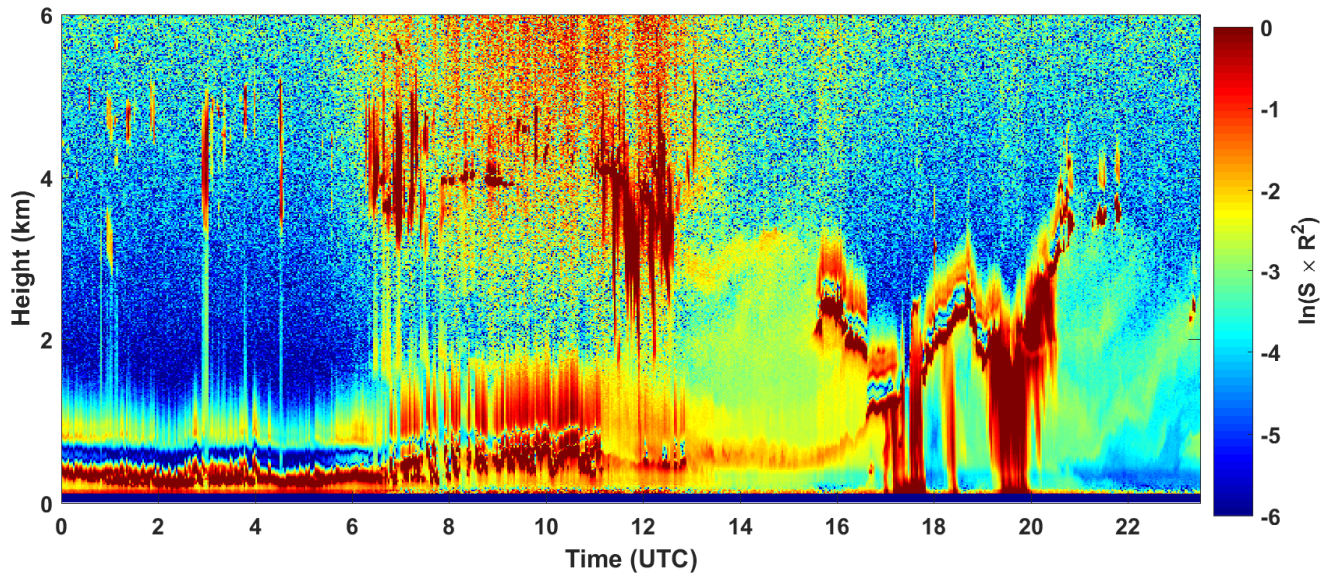
2018-04-06 RCS quick look CHM15k - ILVA LIDAR1 DIREZIONE
