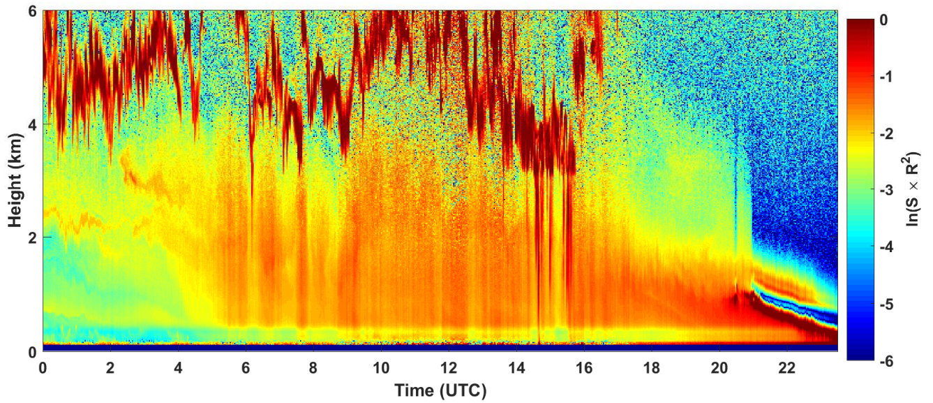
2018-04-16 RCS quick look CHM15k - ILVA LIDAR1 DIREZIONE
