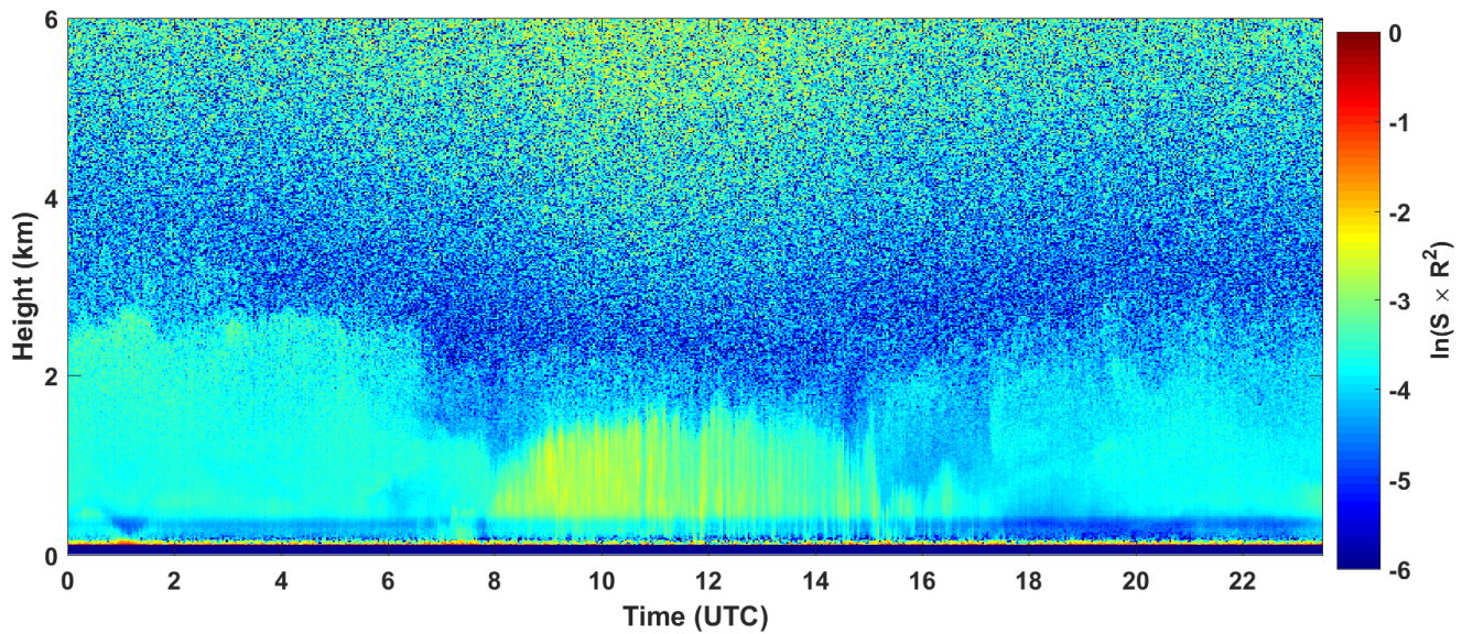
2018-04-20 RCS quick look CHM15k - ILVA LIDAR1 DIREZIONE
