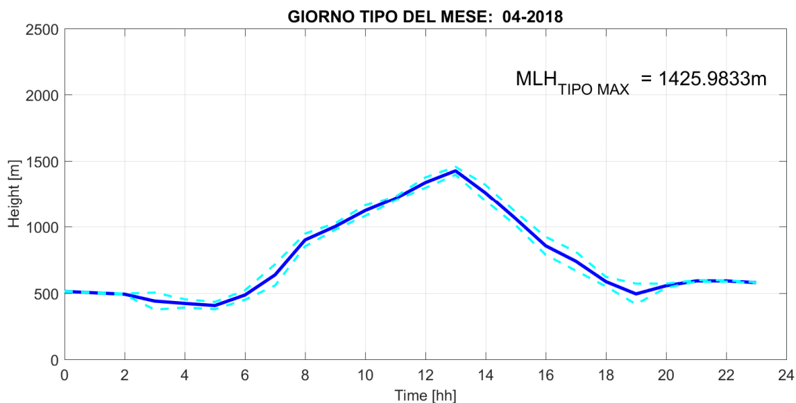
Fig. 2: Giorno tipo del parametro Mixing Layer Height nel mese di APRILE 2018, rappresentato mediante media oraria (linea blu continua), e quartili corrispondenti ad una deviazione standard (linee celesti tratteggiate).
