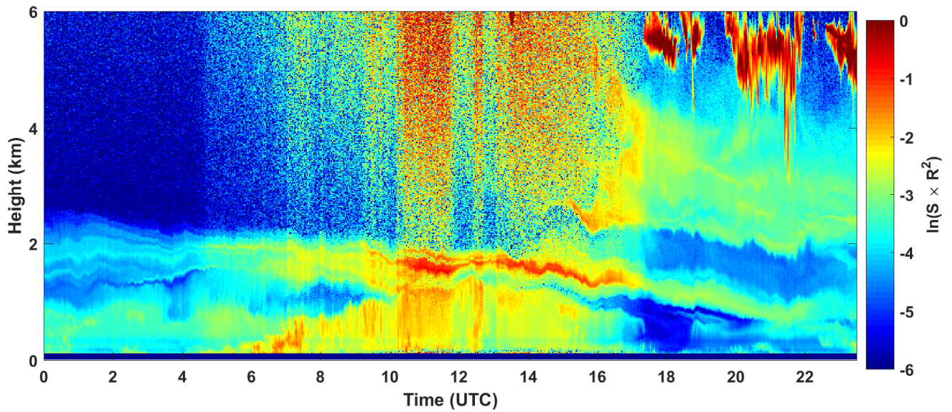
2018-04-14 RCS quick look CHM15k - ILVA LIDAR2 PARCHI
