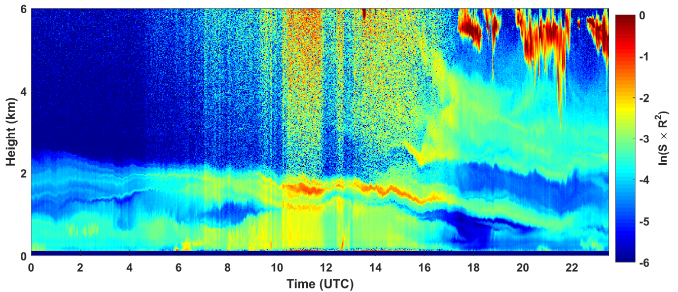
2018-04-14 RCS quick look CHM15k - ILVA LIDAR3 AGGLOMERATO
