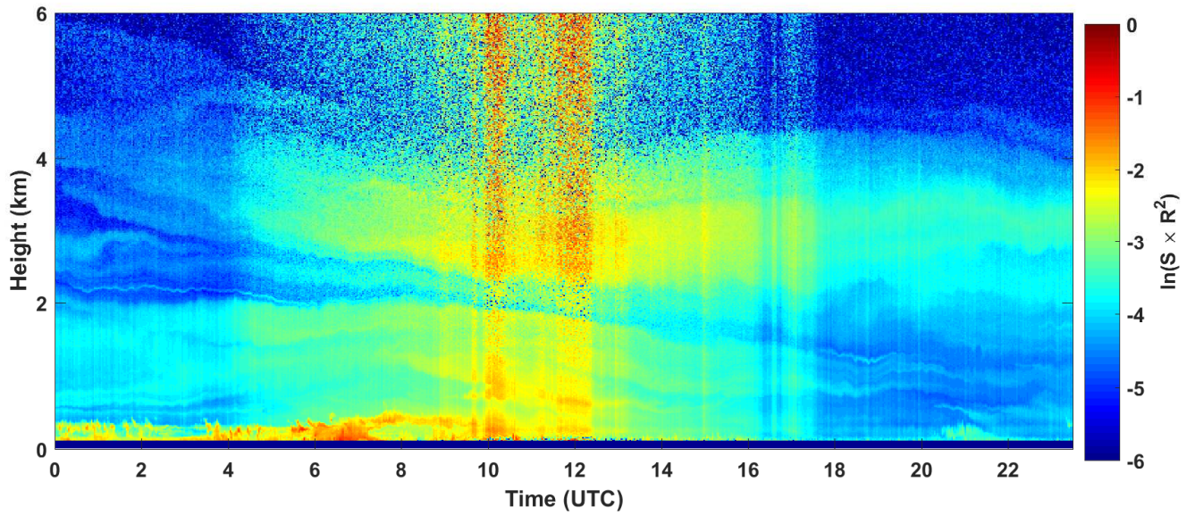
2018-04-26 RCS quick look CHM15k - ILVA LIDAR3 AGGLOMERATO
