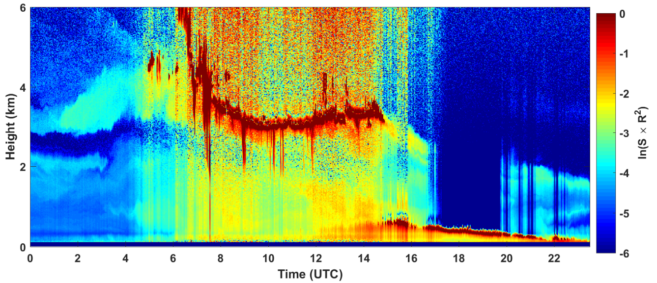
2018-04-10 RCS quick look CHM15k - ILVA LIDAR2 PARCHI
