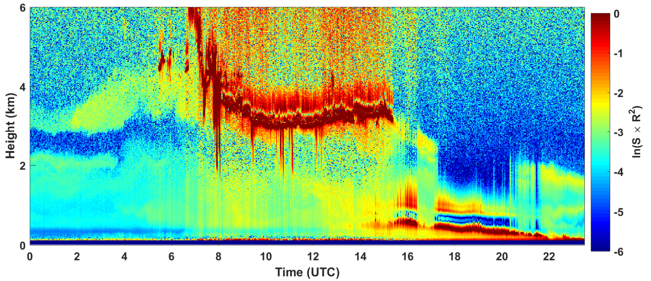
2018-04-10 RCS quick look CHM15k - ILVA LIDAR1 DIREZIONE
