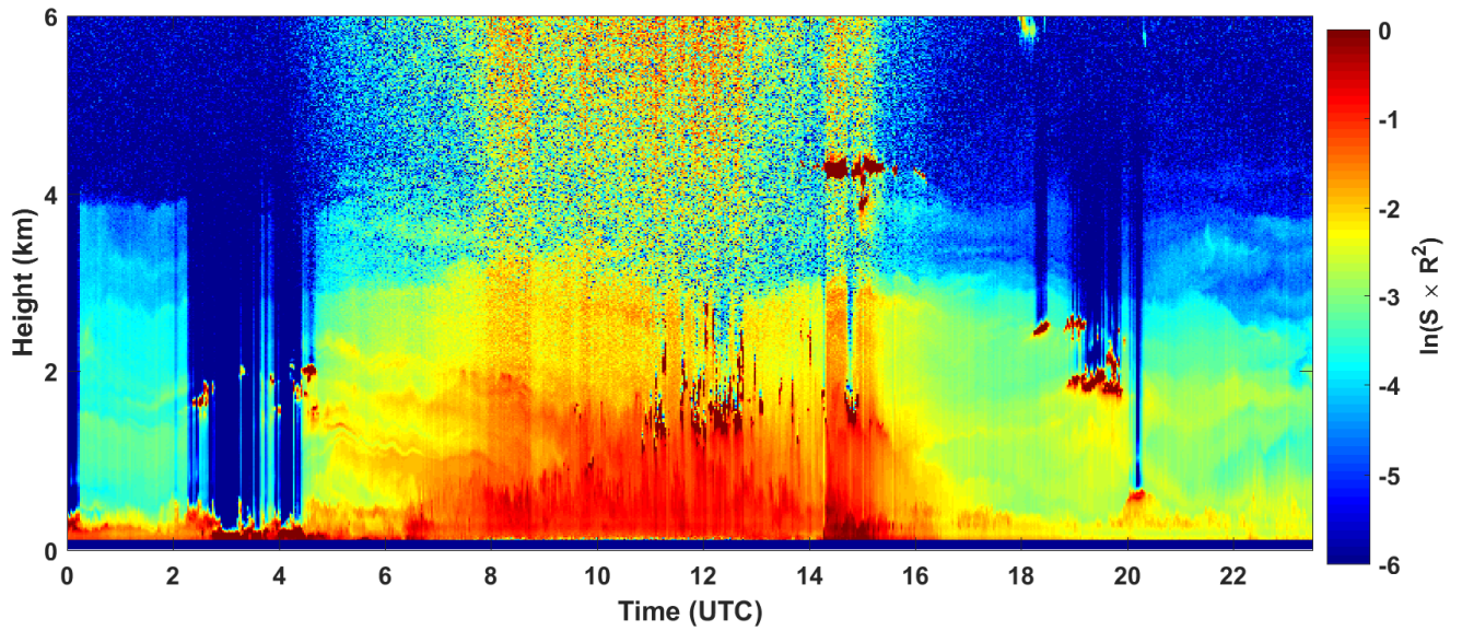
2018-04-18 RCS quick look CHM15k - ILVA LIDAR3 AGGLOMERATO
