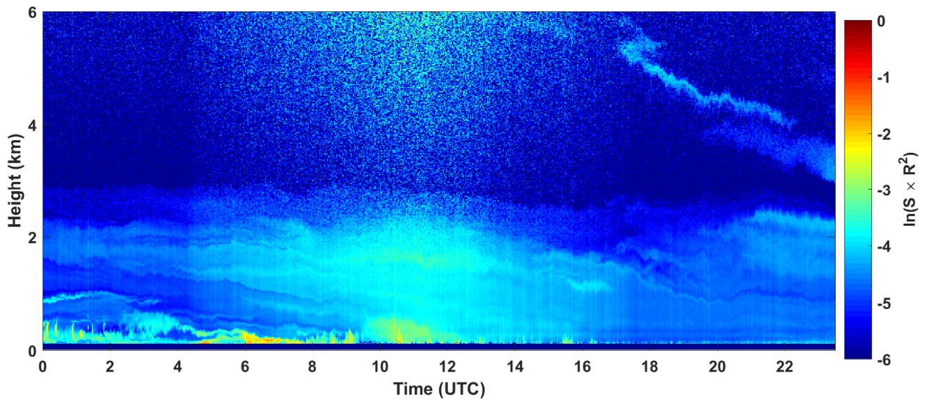
2018-04-08 RCS quick look CHM15k - ILVA LIDAR3 AGGLOMERATO
