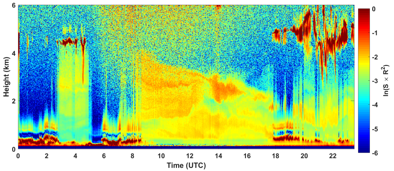
2018-04-12 RCS quick look CHM15k - ILVA LIDAR1 DIREZIONE
