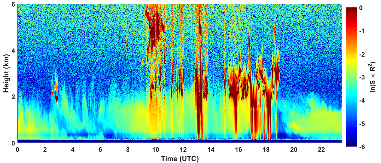
2018-04-04 RCS quick look CHM15k - ILVA LIDAR1 DIREZIONE
