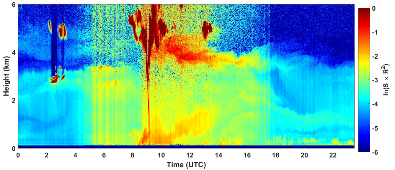
2018-04-30 RCS quick look CHM15k - ILVA LIDAR3 AGGLOMERATO
