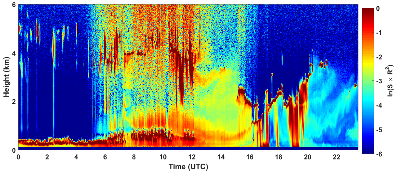
2018-04-06 RCS quick look CHM15k - ILVA LIDAR2 PARCHI
