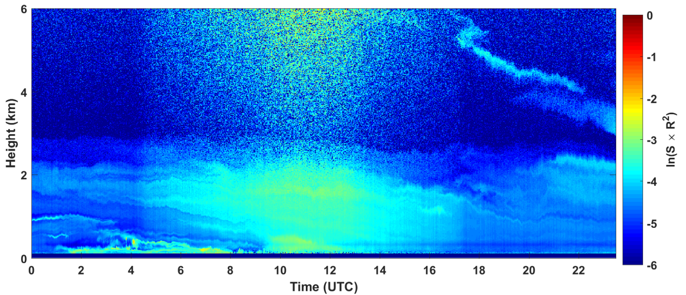
2018-04-08 RCS quick look CHM15k - ILVA LIDAR2 PARCHI
