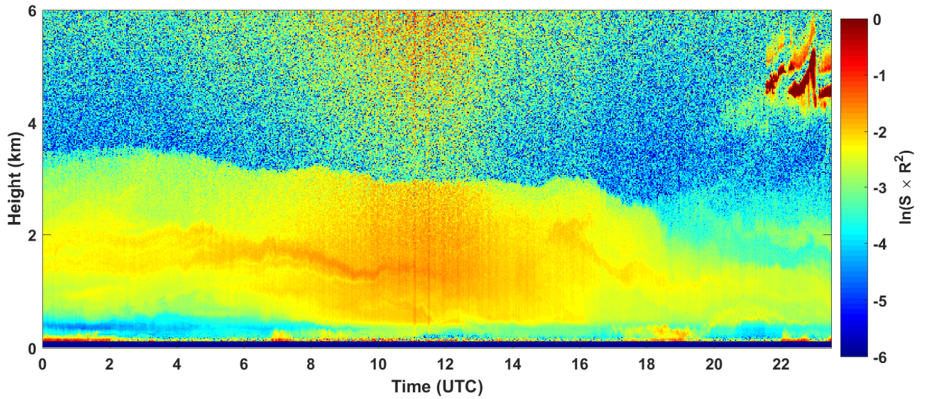
2018-04-28 RCS quick look CHM15k - ILVA LIDAR1 DIREZIONE
