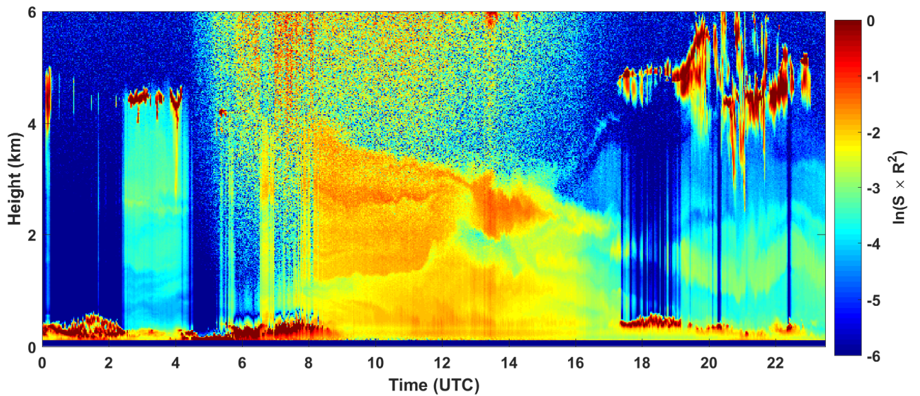
2018-04-12 RCS quick look CHM15k - ILVA LIDAR2 PARCHI
