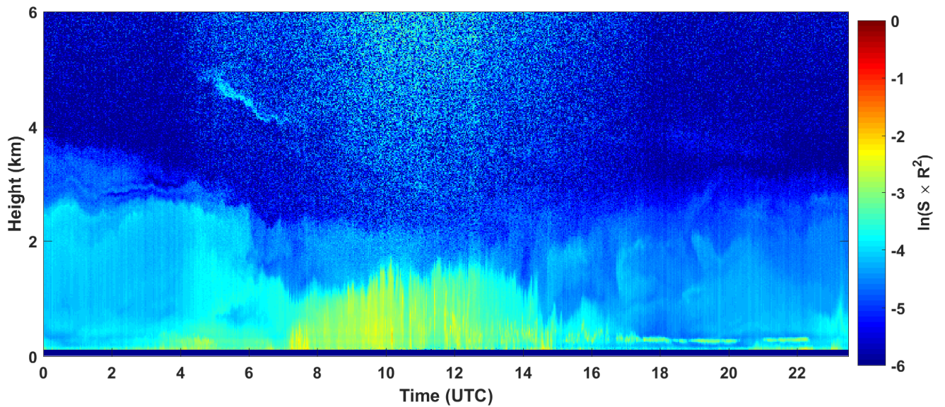
2018-04-20 RCS quick look CHM15k - ILVA LIDAR3 AGGLOMERATO
