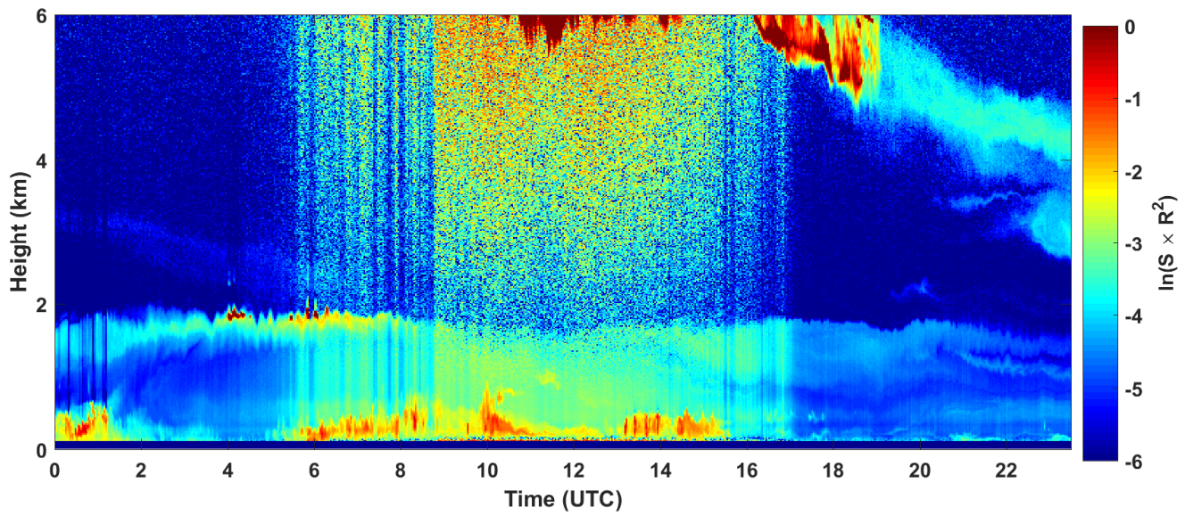
2018-04-10 RCS quick look CHM15k - ILVA LIDAR3 AGGLOMERATO
