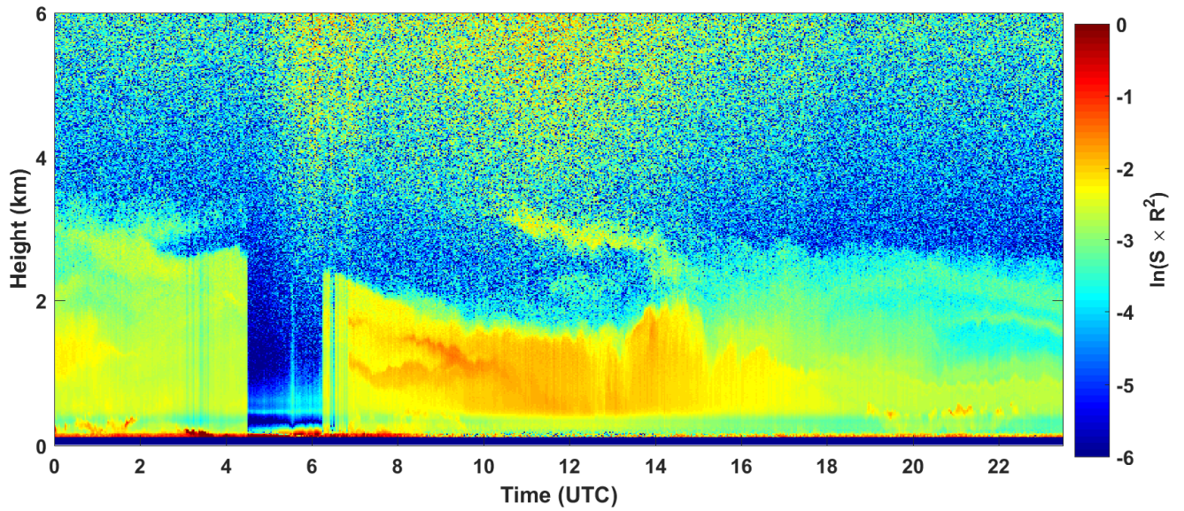
2018-04-14 RCS quick look CHM15k - ILVA LIDAR1 DIREZIONE
