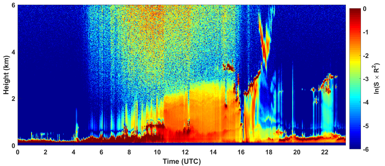
2018-04-16 RCS quick look CHM15k - ILVA LIDAR3 AGGLOMERATO
