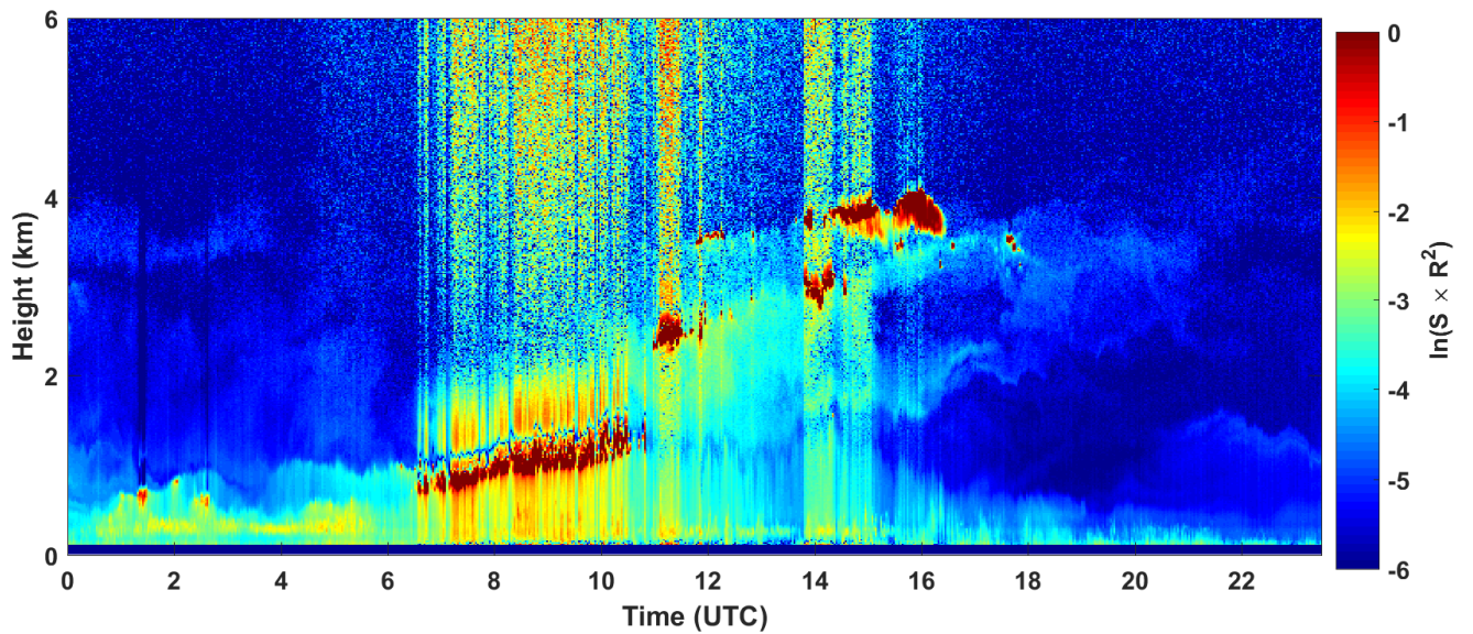
2018-04-06 RCS quick look CHM15k - ILVA LIDAR3 AGGLOMERATO
