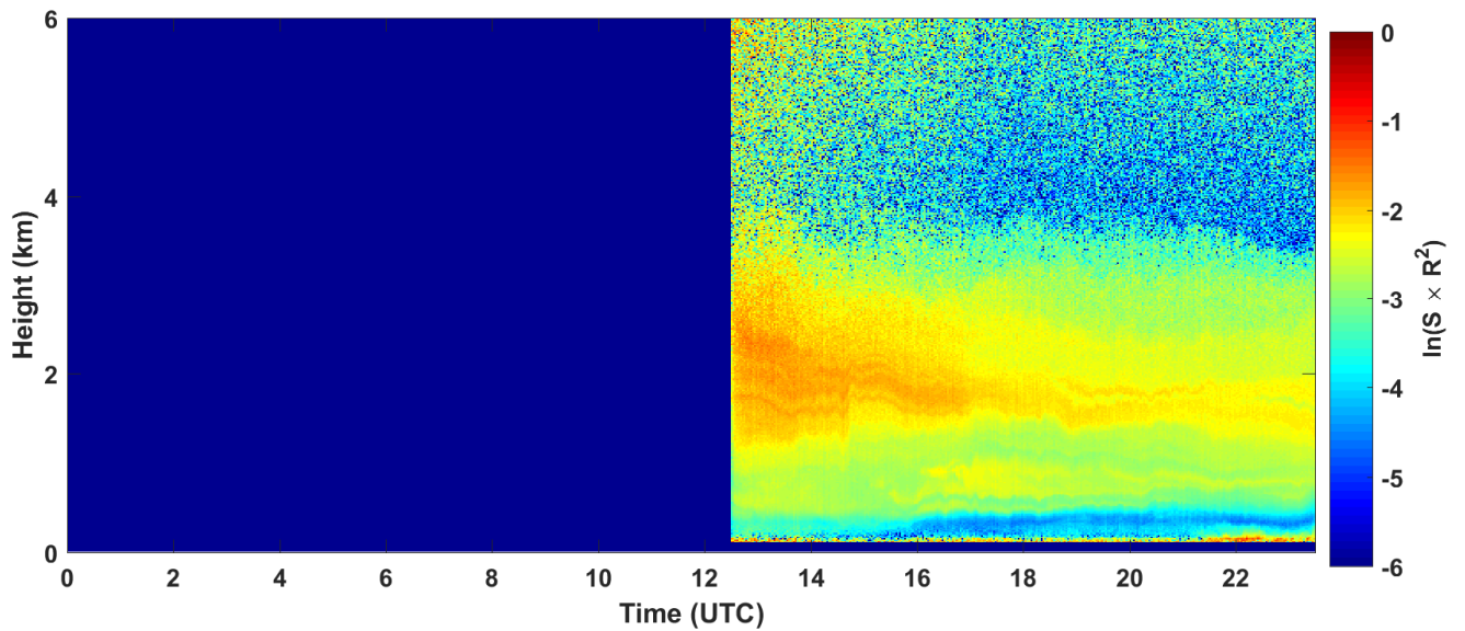
2018-04-26 RCS quick look CHM15k - ILVA LIDAR1 DIREZIONE
