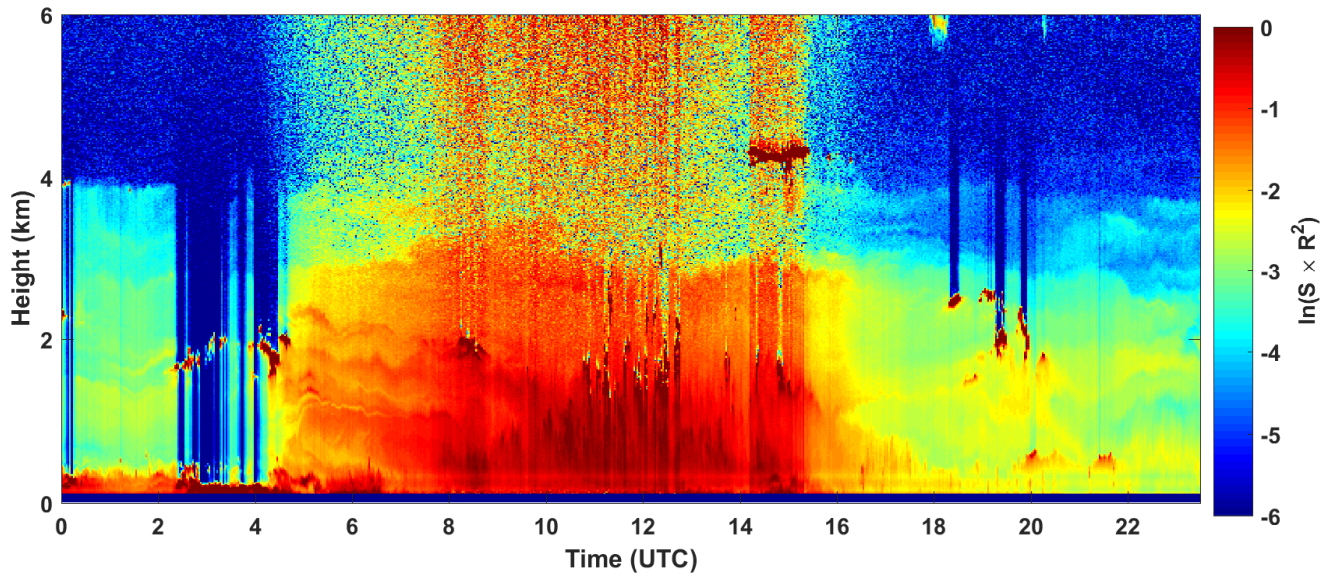
2018-04-18 RCS quick look CHM15k - ILVA LIDAR2 PARCHI
