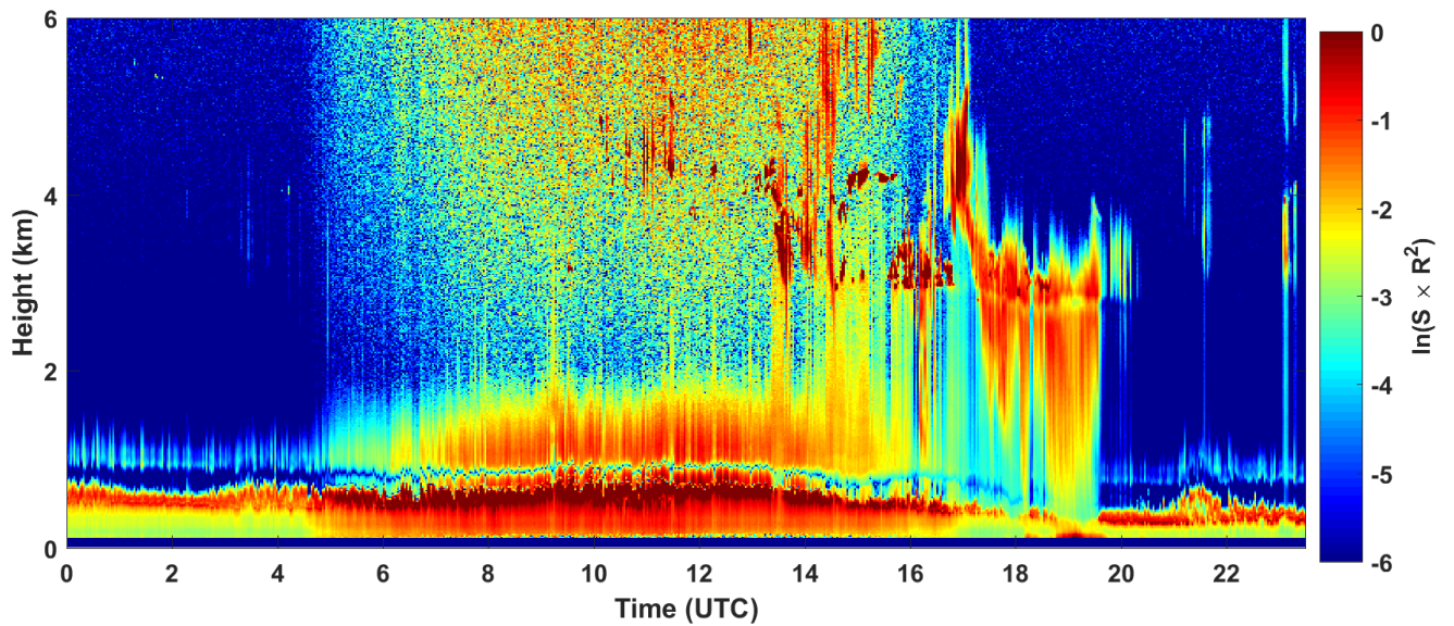
2018-04-04 RCS quick look CHM15k - ILVA LIDAR3 AGGLOMERATO
