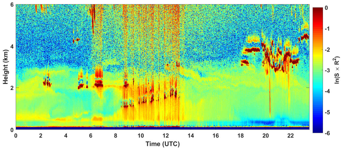
2018-04-18 RCS quick look CHM15k - ILVA LIDAR1 DIREZIONE
