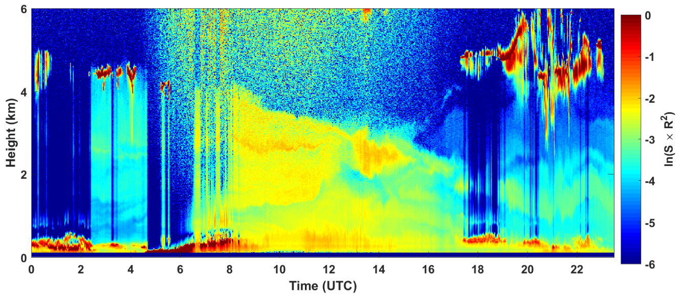
2018-04-12 RCS quick look CHM15k - ILVA LIDAR3 AGGLOMERATO
