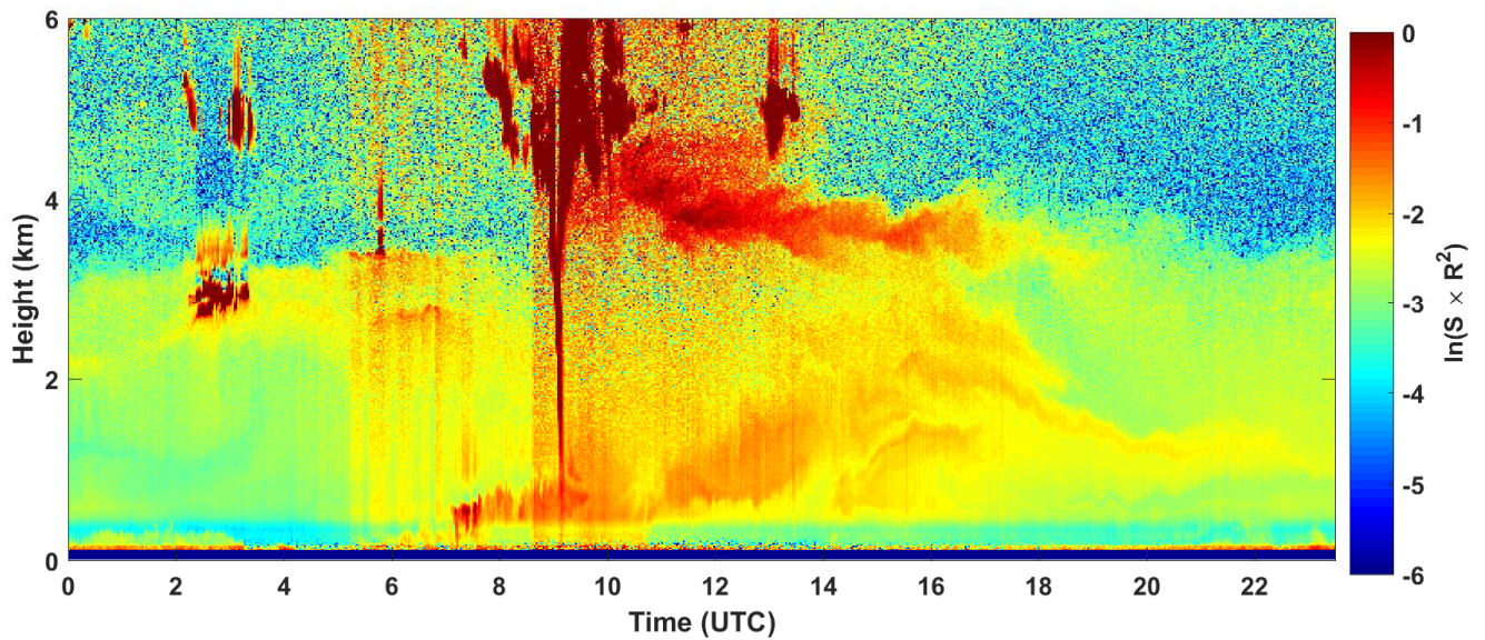
2018-04-29 RCS quick look CHM15k - ILVA LIDAR1 DIREZIONE
