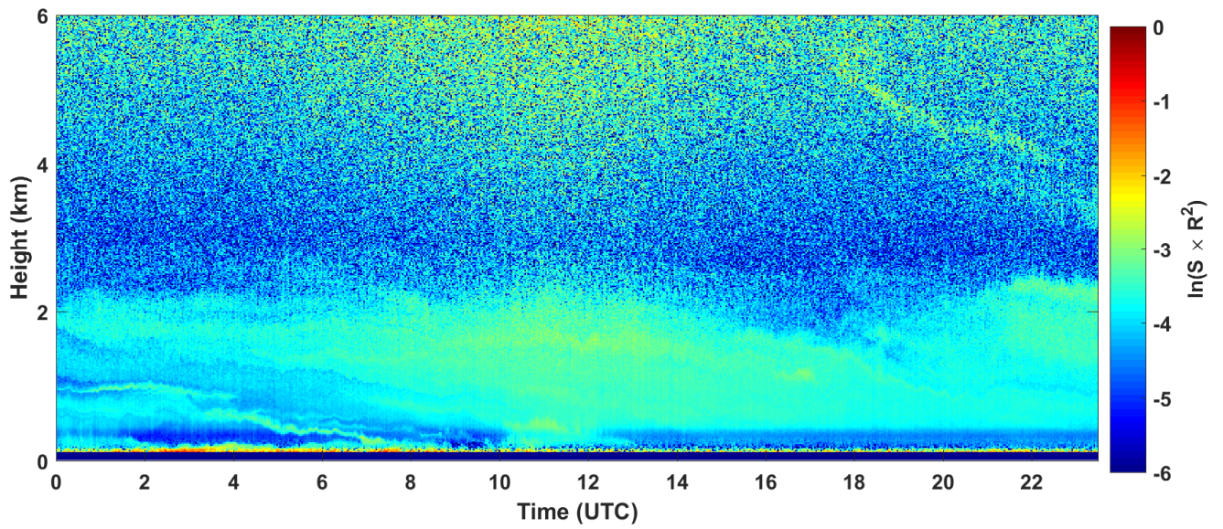
2018-04-08 RCS quick look CHM15k - ILVA LIDAR1 DIREZIONE
