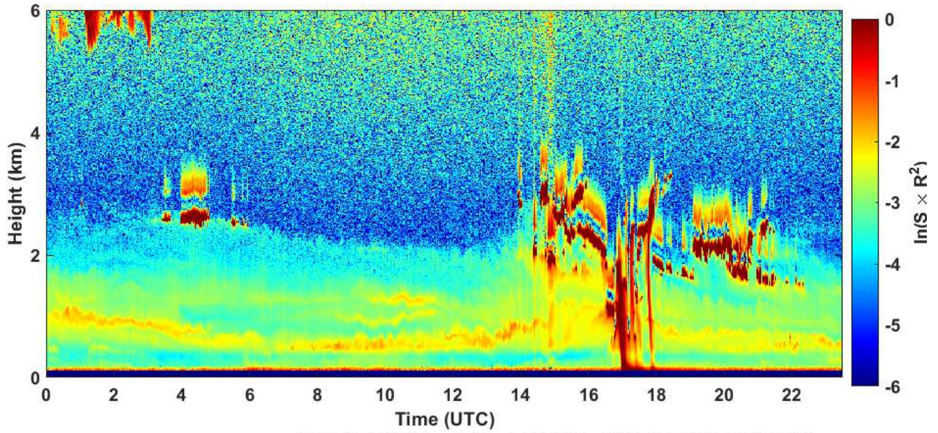
2020-11-14 RCS quick look CHM15k - ILVA LIDAR1 DIREZIONE
