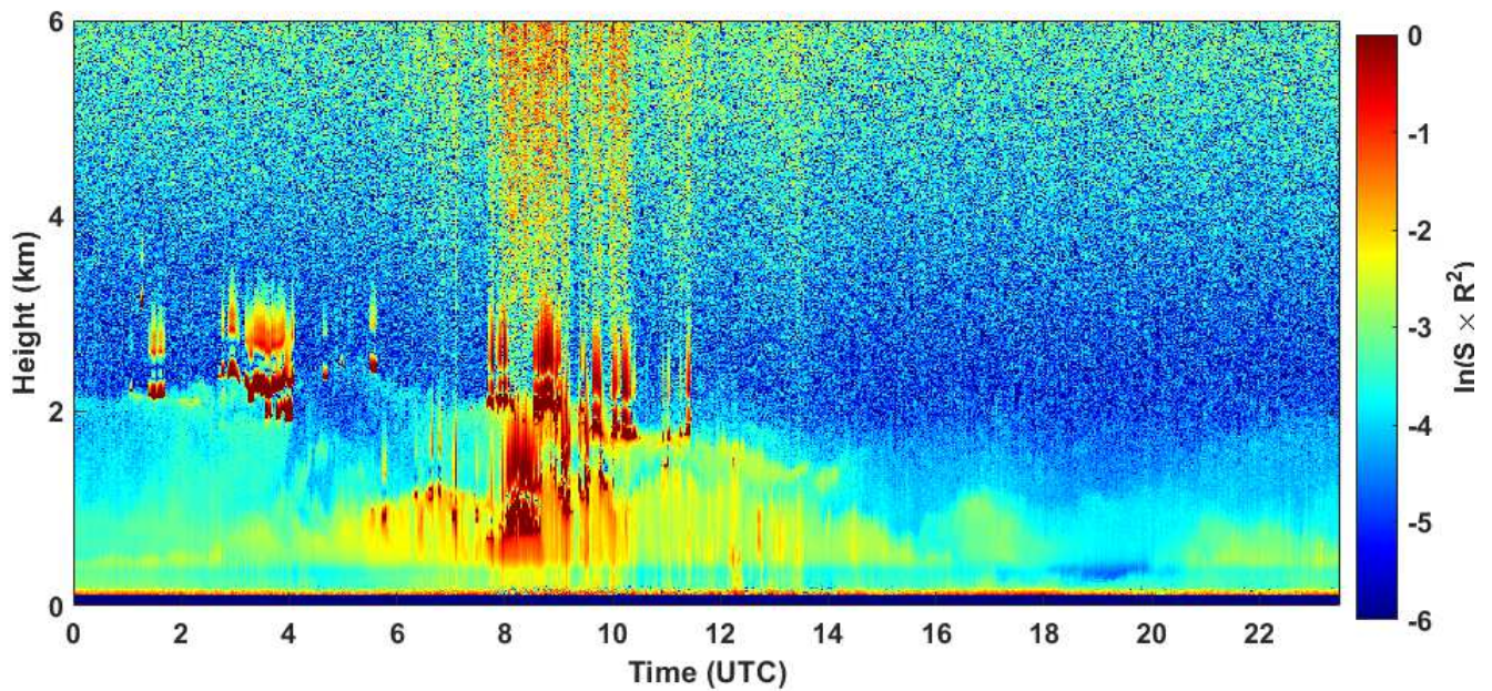
2020-11-06 RCS quick look CHM15k - ILVA LIDAR1 DIREZIONE
