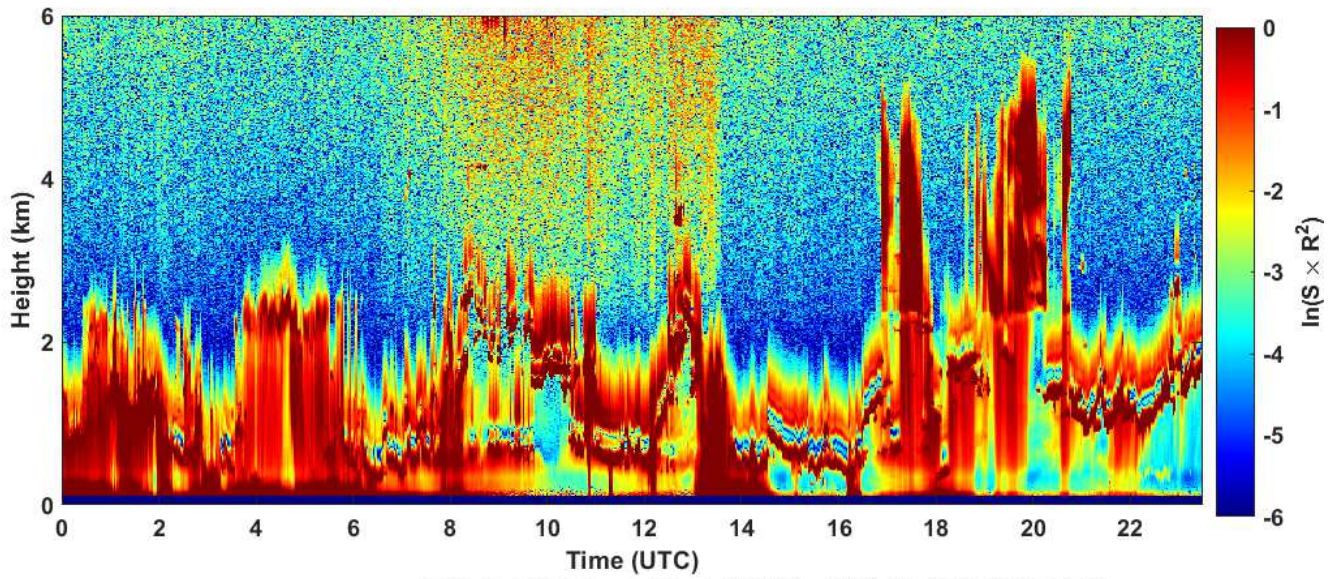
2020-11-30 RCS quick look CHM15k - ILVA LIDAR1 DIREZIONE
