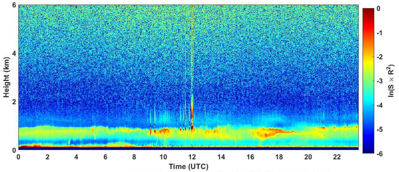
2020-11-28 RCS quick look CHM15k - ILVA LIDAR1 DIREZIONE
