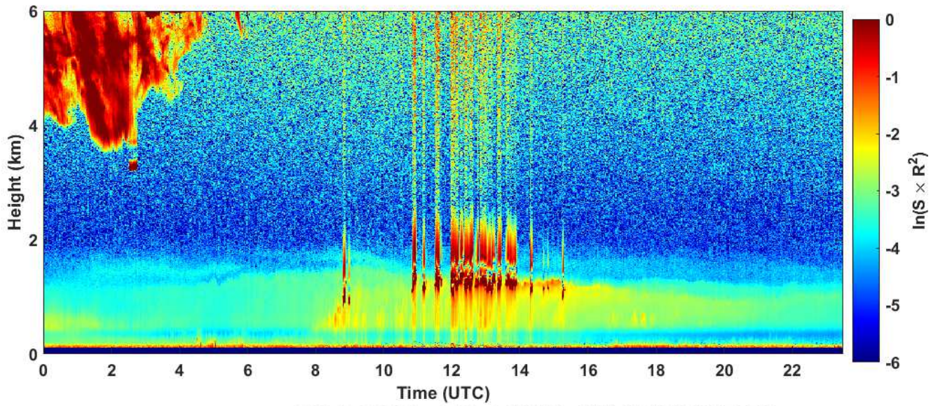
2020-11-26 RCS quick look CHM15k - ILVA LIDAR1 DIREZIONE
