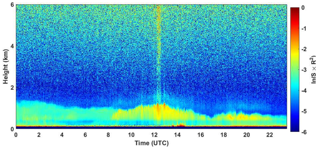
2020-11-08 RCS quick look CHM15k - ILVA LIDAR1 DIREZIONE
