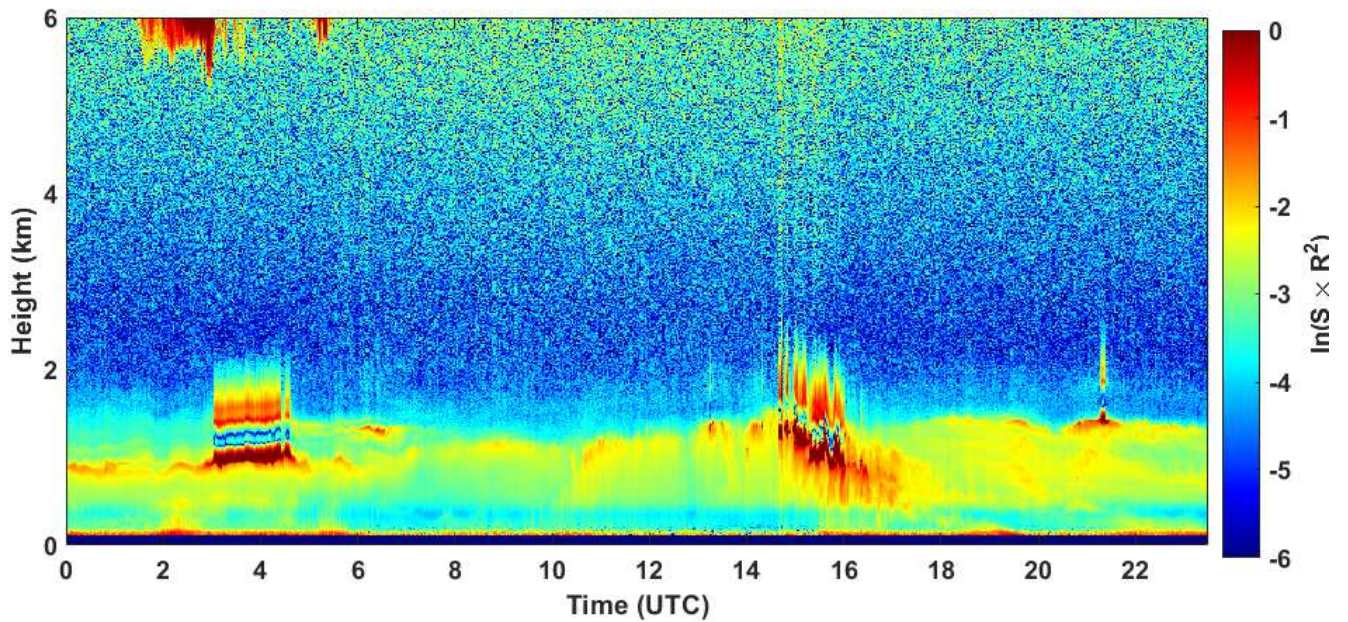
2020-11-02 RCS quick look CHM15k - ILVA LIDAR1 DIREZIONE
