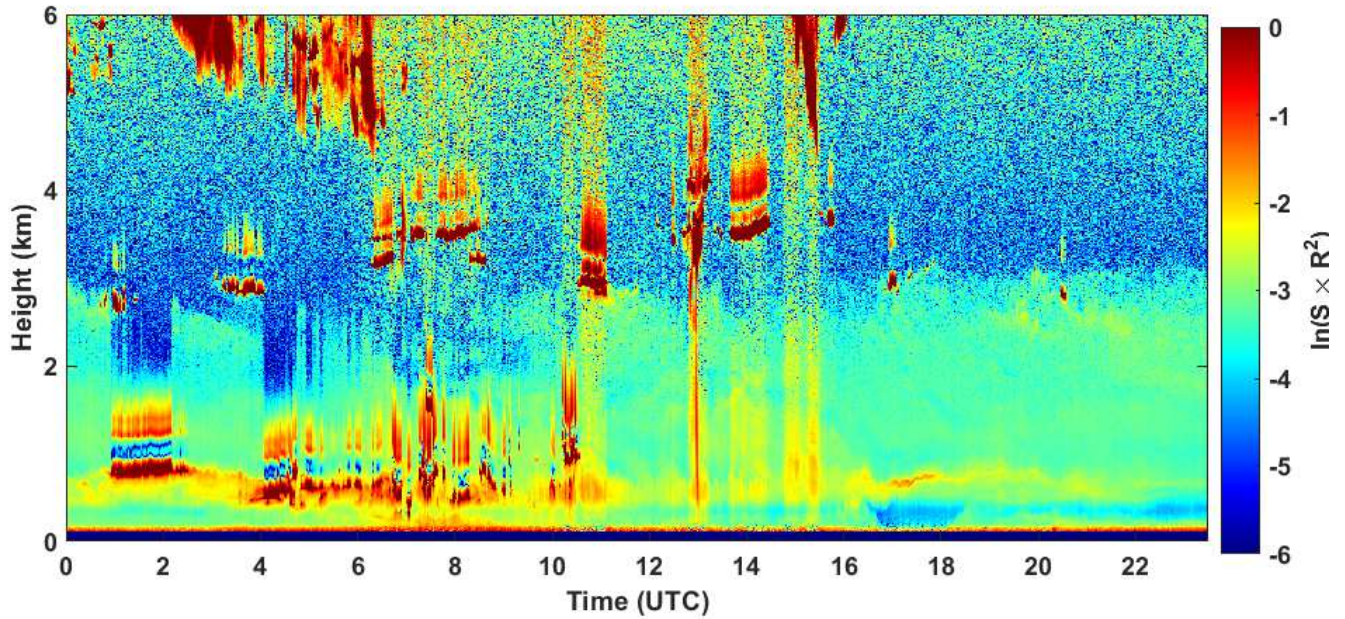
2020-11-16 RCS quick look CHM15k - ILVA LIDAR1 DIREZIONE
