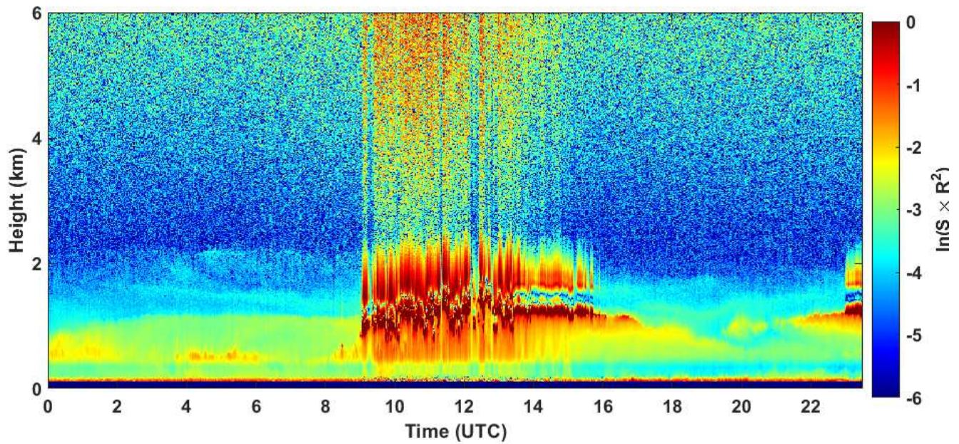
2020-11-12 RCS quick look CHM15k - ILVA LIDAR1 DIREZIONE
