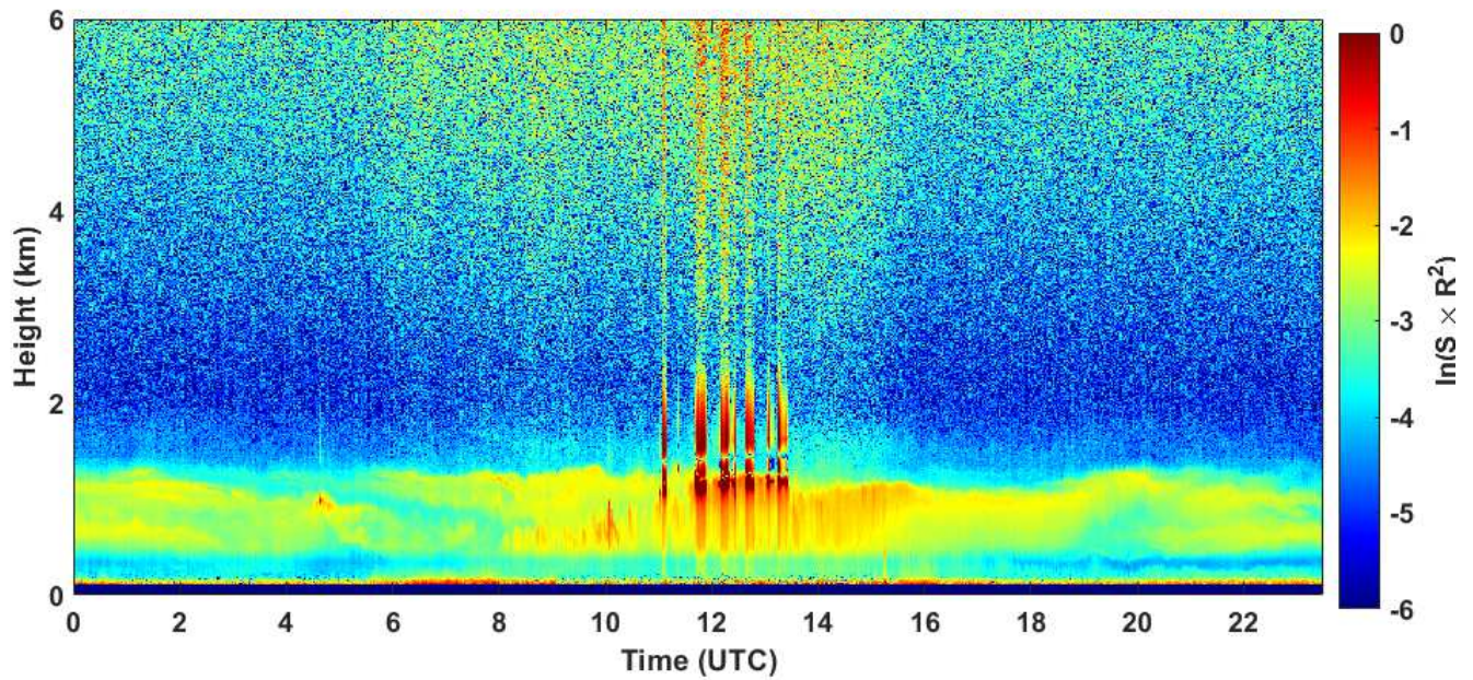
2020-11-04 RCS quick look CHM15k - ILVA LIDAR1 DIREZIONE
