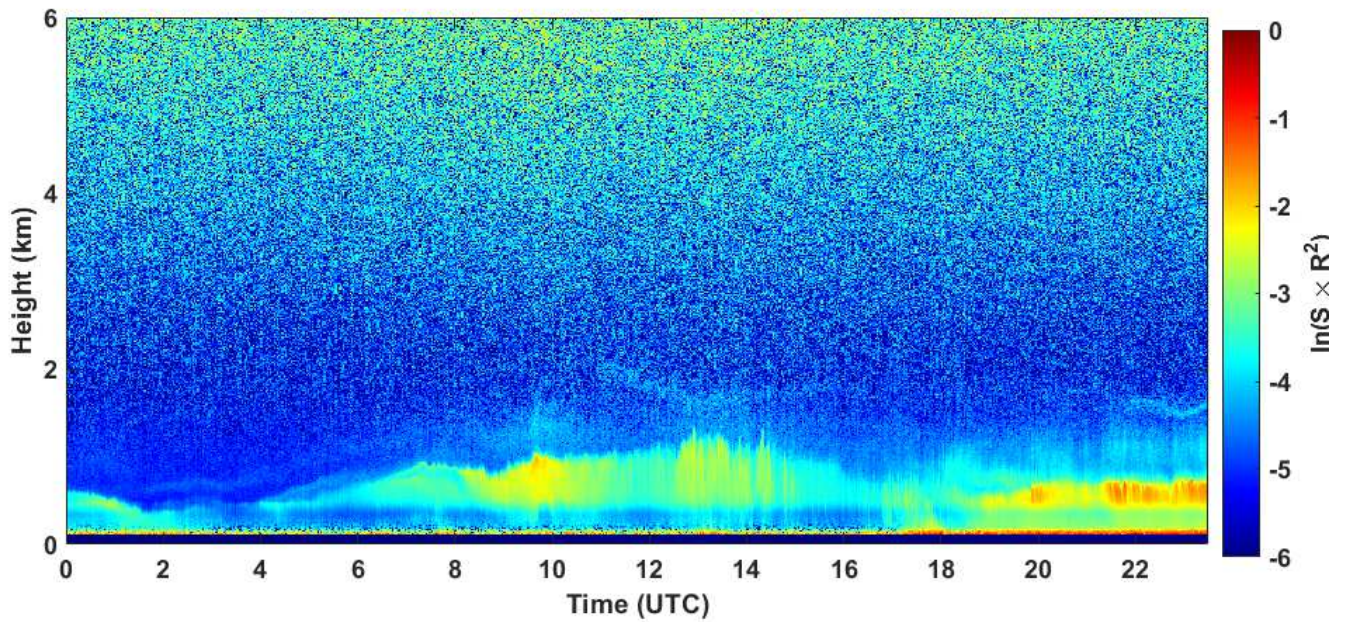
2020-11-10 RCS quick look CHM15k - ILVA LIDAR1 DIREZIONE
