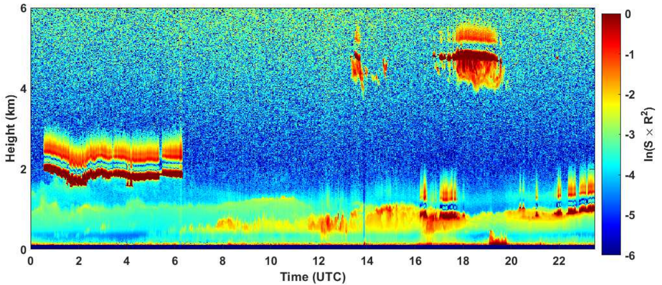
2020-11-24 RCS quick look CHM15k - ILVA LIDAR1 DIREZIONE
