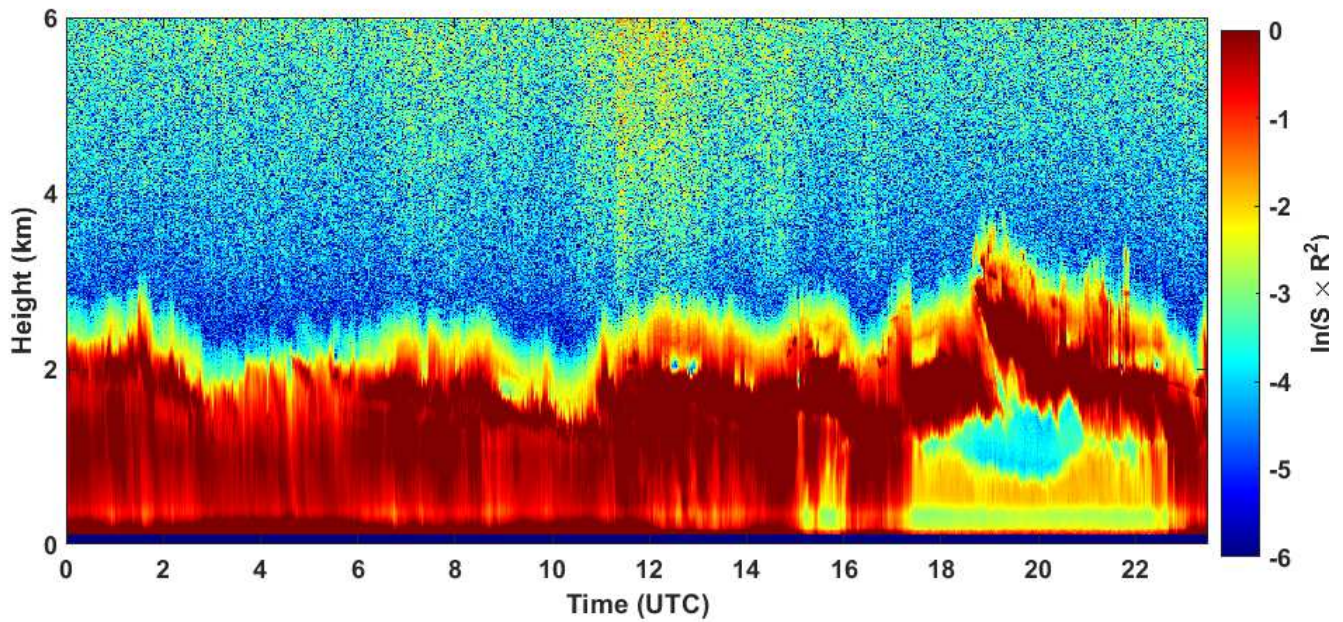
2020-11-22 RCS quick look CHM15k - ILVA LIDAR1 DIREZIONE
