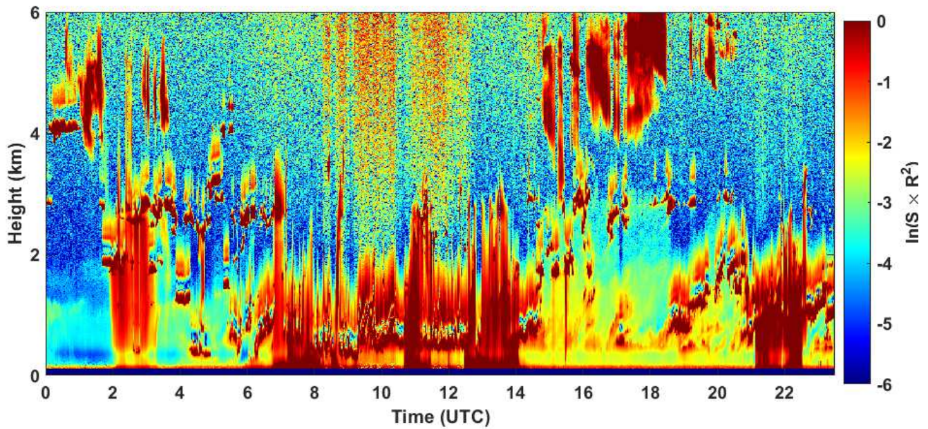
2020-11-18 RCS quick look CHM15k - ILVA LIDAR1 DIREZIONE
