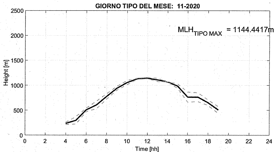
Fig. 2: Giorno tipo del parametro Mixing Layer Height nel mese di NOVEMBRE 2020, rappresentato mediante media oraria (linea blu continua) e deviazione standard (linee celesti tratteggiate).
