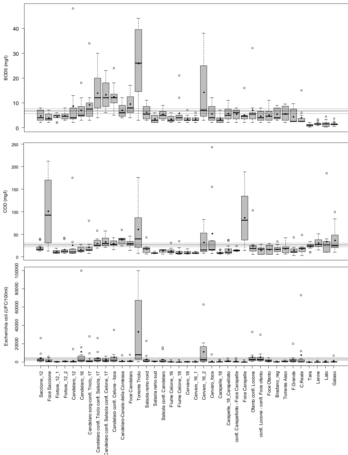
Box plots relativi ai parametri BOD5 (mg/l), COD (mg/l), Escherichia coli (UFC/100ml) misurati durante il periodo aprile 2014 – marzo 2015 nei corpi idrici della categoria “Corsi d’acqua” della Regione Puglia. Sono rappresentate anche le misure che, per alcuni corpi idrici, vengono riportate in tabella con la dicitura “minore del limite di quantificazione” (m.l.q.). Il pallino nero indica il valore medio, la barra nera indica la mediana, il limite superiore e inferiore del box indicano rispettivamente il 75esimo e il 25esimo percentile, le barre di errore indicano il limite superiore ed inferiore degli outliers, i pallini vuoti indicano gli outliers. La linea orizzontale continua e le linee tratteggiate identificano, rispettivamente, il valore medio e gli intervalli di confidenza al 99% dell’intero set di dati.
