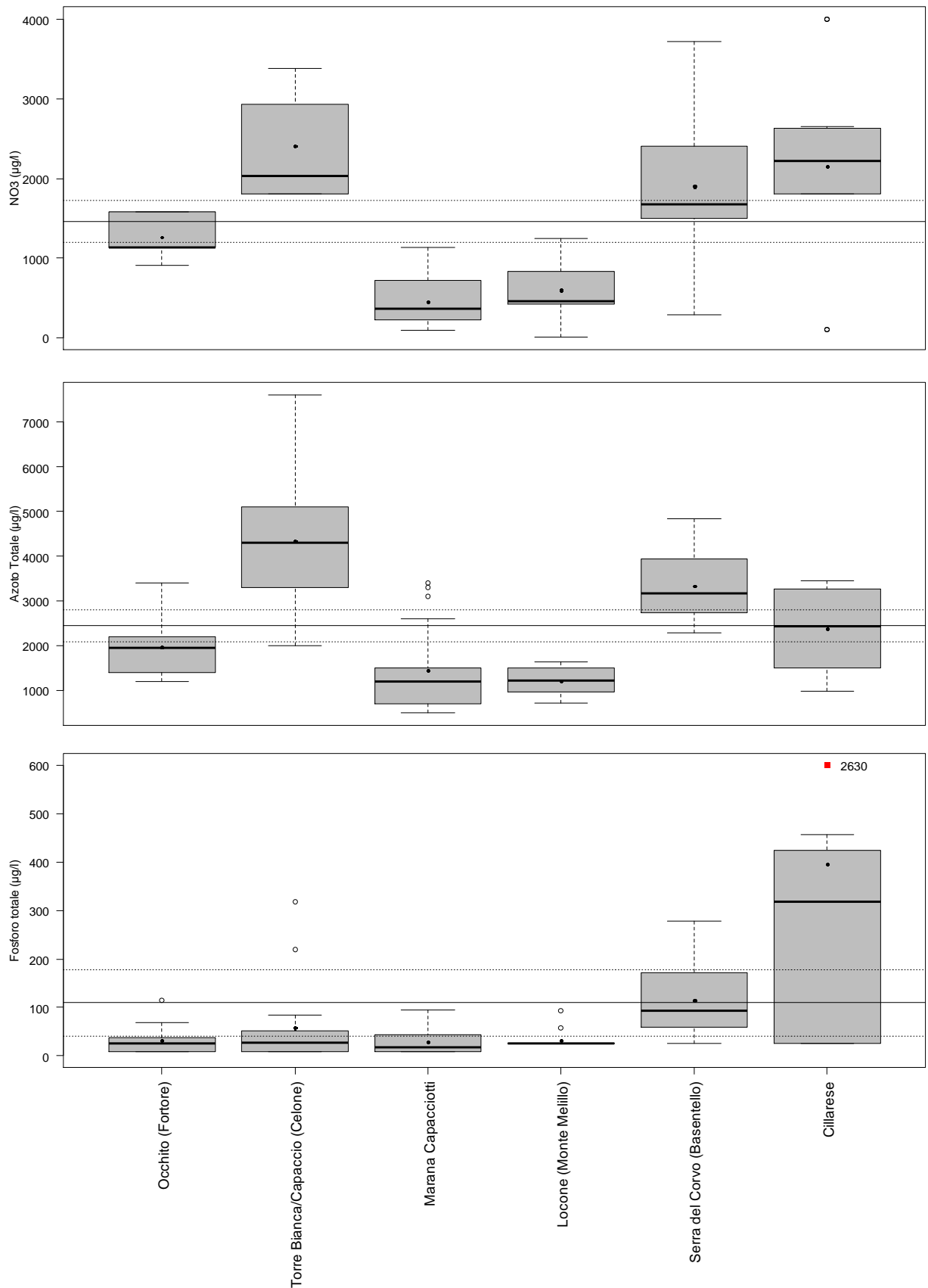
Box plots relativi ai parametri NO 3 (µg/l), azoto totale (µg/l), fosforo totale (µg/l) misurati durante il periodo aprile 2014 – marzo 2015 nei corpi idrici della categoria “Laghi e Invasi” della Regione Puglia. Sono rappresentate anche le misure che, per alcuni corpi idrici, vengono riportate in tabella con la dicitura “minore del limite di quantificazione” (m.l.q.). Il pallino nero indica il valore medio, la barra nera indica la mediana, il limite superiore e inferiore del box indicano rispettivamente il 75esimo e il 25simo percentile, le barre di errore indicano il limite superiore ed inferiore degli outliers, i pallini vuoti indicano gli outliers. La linea orizzontale continua e le linee tratteggiate identificano, rispettivamente, il valore medio e gli intervalli di confidenza al 99% dell’intero set di dati.
