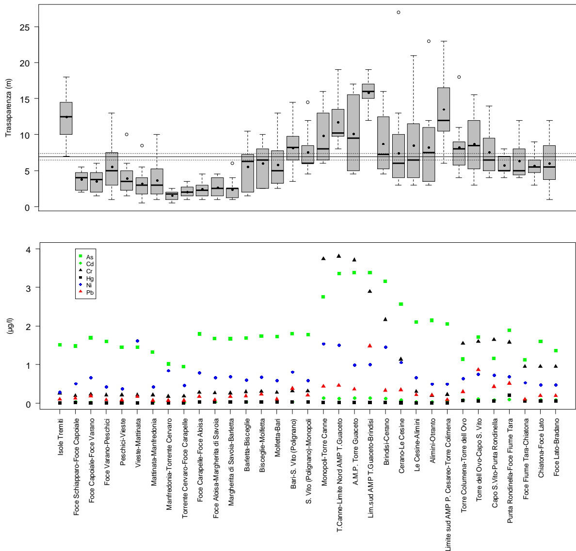
Box plot relativo al parametro trasparenza (m) e grafico dei valori medi dei metalli pesanti Arsenico, Cadmio, Cromo, Mercurio, Nichel, Piombo, misurati durante il periodo aprile 2014 – marzo 2015 nei corpi idrici della categoria “Acque Marino Costiere” della Regione Puglia. Sono rappresentate anche le misure che, per alcuni corpi idrici, vengono riportate in tabella con la dicitura “minore del limite di quantificazione” (m.l.q.). Il pallino nero indica il valore medio, la barra nera indica la mediana, il limite superiore e inferiore del box indicano rispettivamente il 75esimo e il 25esimo percentile, le barre di errore indicano il limite superiore ed inferiore degli outliers, i pallini vuoti indicano gli outliers. La linea orizzontale continua e le linee tratteggiate identificano, rispettivamente, il valore medio e gli intervalli di confidenza al 99% dell’intero set di dati.
