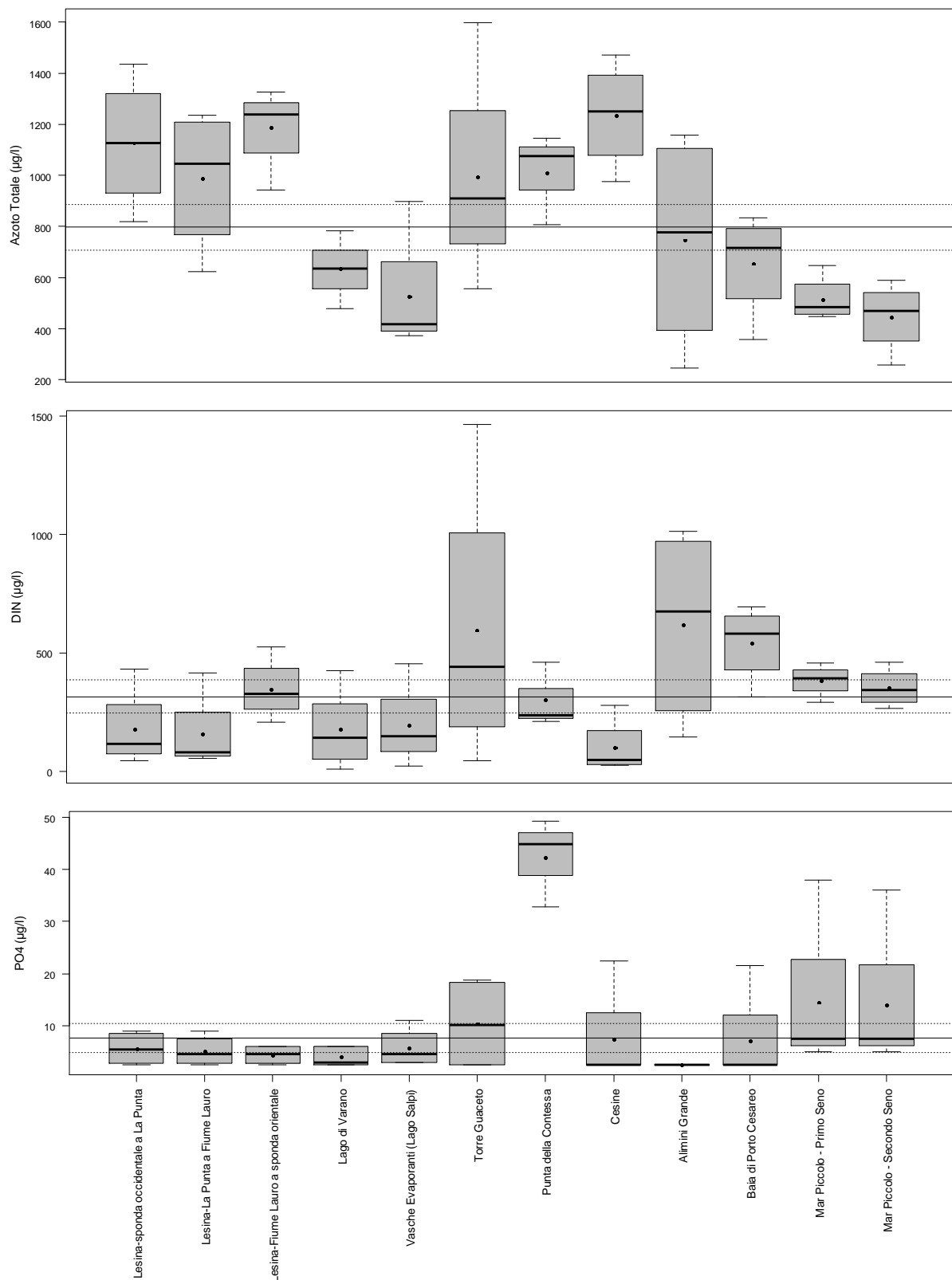
Box plots relativi ai parametri azoto totale ( \mu\text{g/l} ), DIN ( \mu\text{g/l} ), e \text{PO}_4 ( \mu\text{g/l} ) misurati durante il periodo aprile 2014 – marzo 2015 nei corpi idrici della categoria “Acque di Transizione” della Regione Puglia. Sono rappresentate anche le misure che, per alcuni corpi idrici, vengono riportate in tabella con la dicitura “minore del limite di quantificazione” (m.l.q.). Il pallino nero indica il valore medio, la barra nera indica la mediana, il limite superiore e inferiore del box indicano rispettivamente il 75esimo e il 25esimo percentile, le barre di errore indicano il limite superiore ed inferiore degli outliers, i pallini vuoti indicano gli outliers. La linea orizzontale continua e le linee tratteggiate identificano, rispettivamente, il valore medio e gli intervalli di confidenza al 99% dell’intero set di dati.
